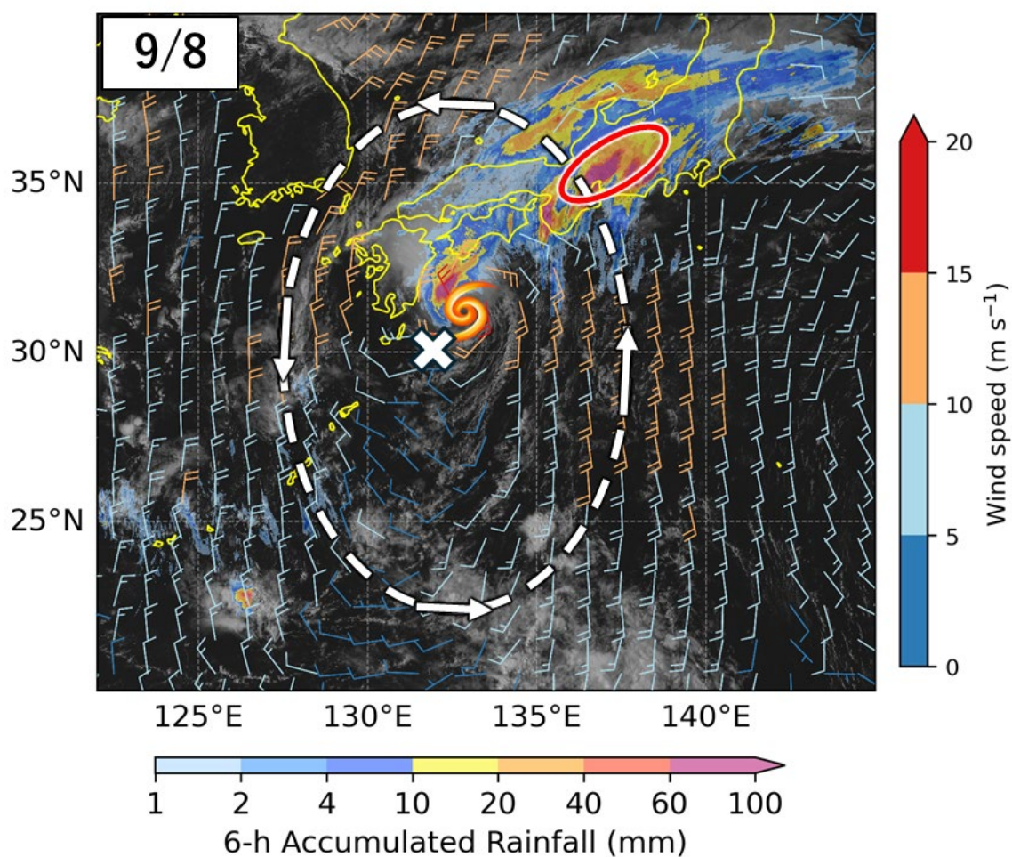
図7. 9月8日におけるモンスーンジャイアの流れと東海地方で発生した線状降水帯。 背景は気象衛星ひまわりの可視画像(白黒)、衛星で観測された海上風(矢羽根)、及び9月8日13時から19時までの6時間積算雨量(カラー)を示す。白破線の楕円はモンスーンジャイアに伴う強い風のおおよその位置、白×はモンスーンジャイアの中心位置、赤丸は線状降水帯が発生した領域を示す。台風マークは元台風第24号(熱帯低気圧)の位置(8日15時頃)を示す。8日はモンスーンジャイアが南北に伸び、形が崩れつつあった。モンスーンジャイアの強風域が日本の南海上で南北に伸びており、これに沿って大量の水蒸気が東海地方に流入し、線状降水帯の発生に影響した可能性がある。
