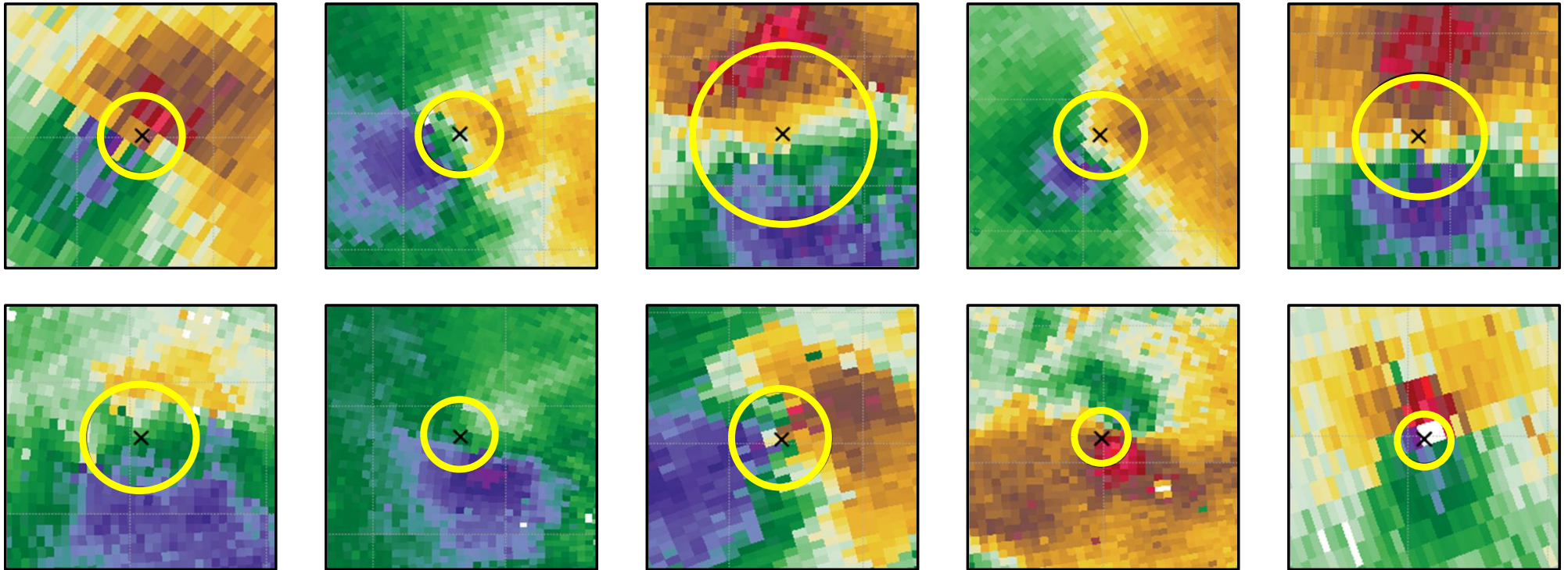
竜巻渦の正解として学習する画像の例 (黄色い丸が渦に伴うパターン)
