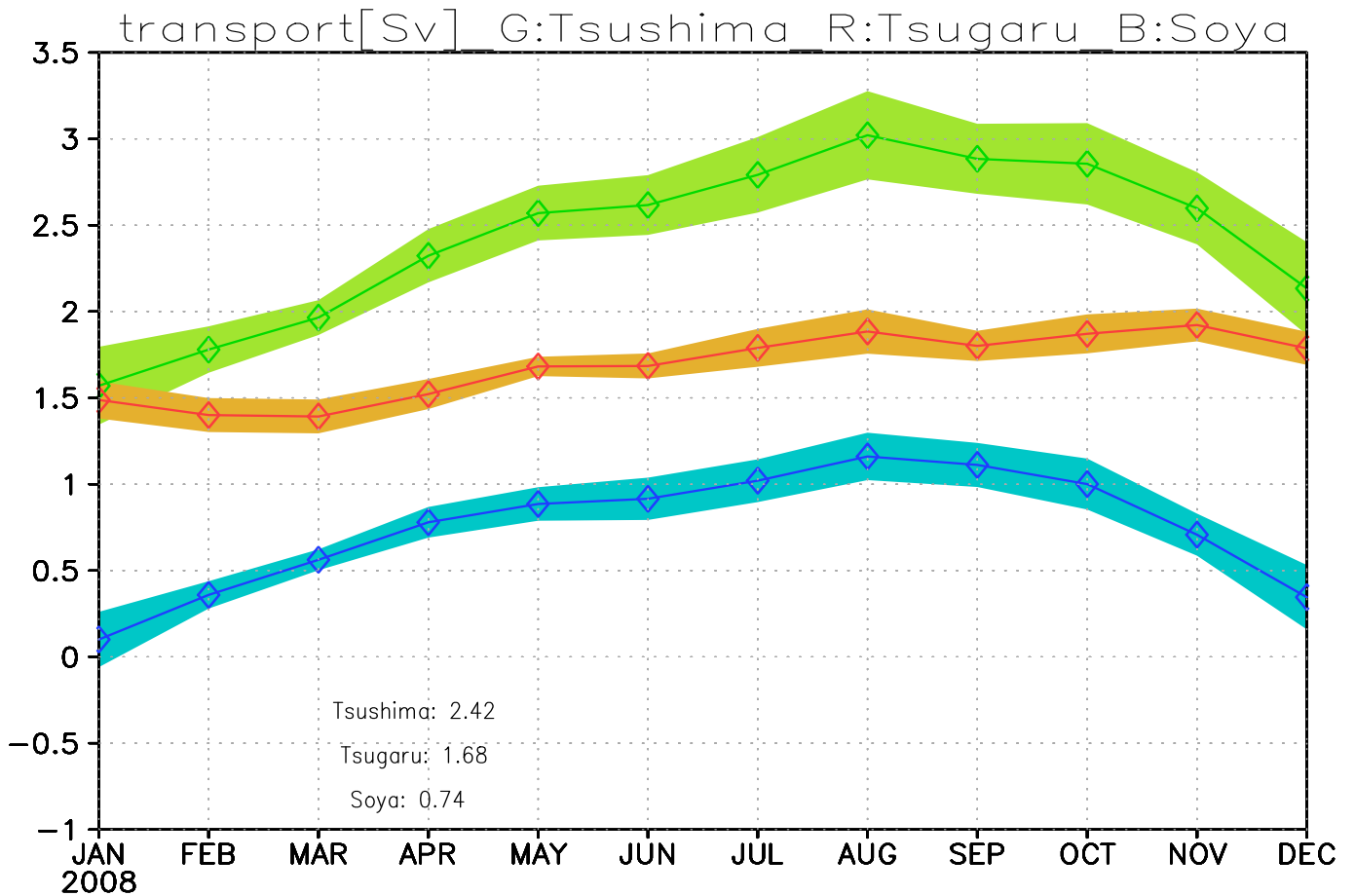
図K - 4 対馬暖流 (緑色), 津軽暖流 (橙色) 及び宗谷暖流 (水色) の流量の季節変化 ( \text{Sv} )。陰影は年々変動の標準偏差を示す。図中の数字は年平均値 ( \text{Sv} ) である。
