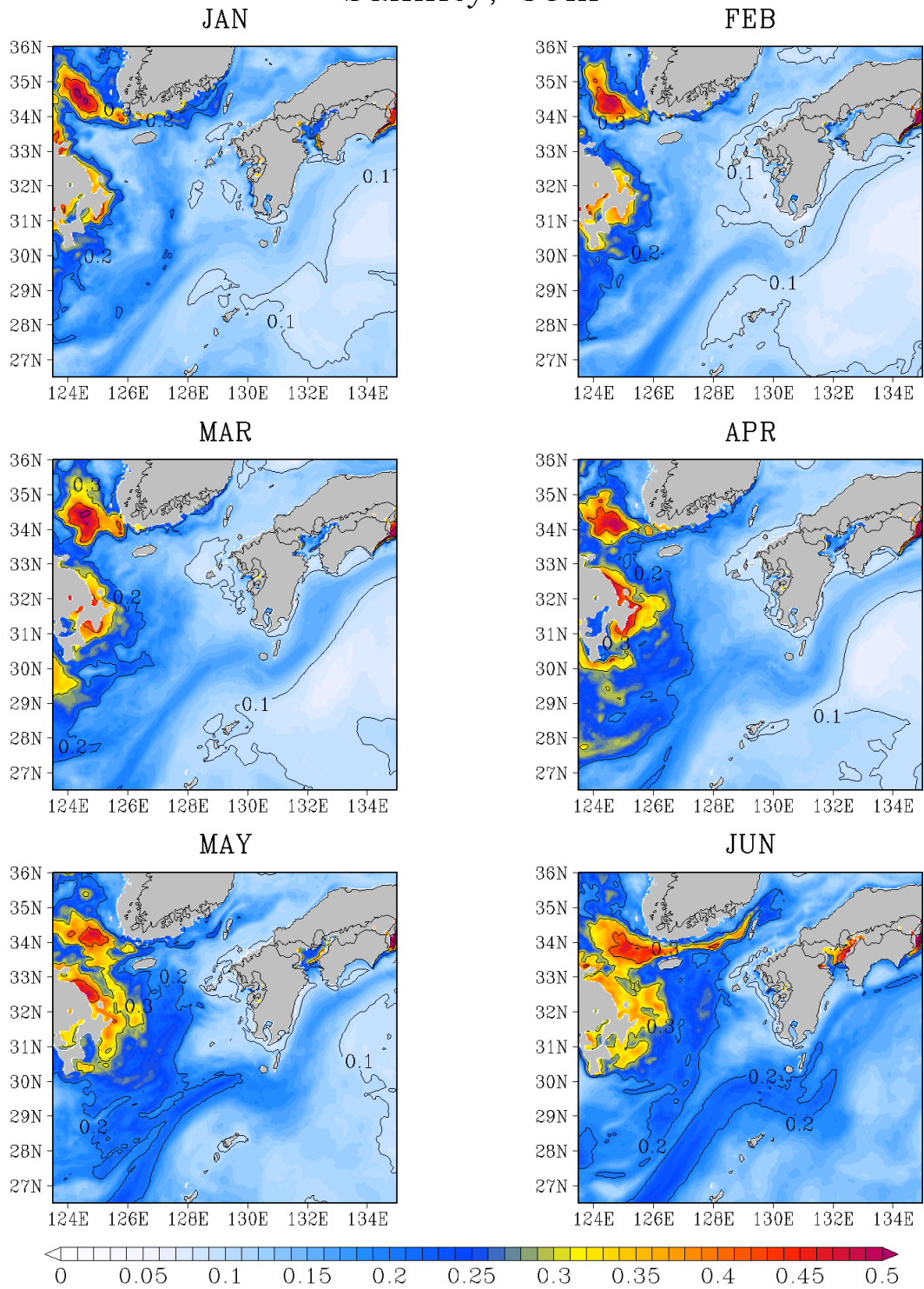
図 G - 17 50 m 深の塩分 標準偏差 (unitless)
