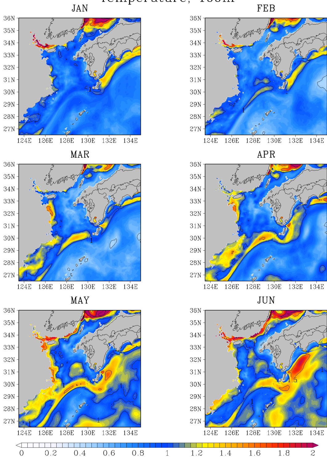
図 G - 8 100 m 深の水温 標準偏差 (°C)
