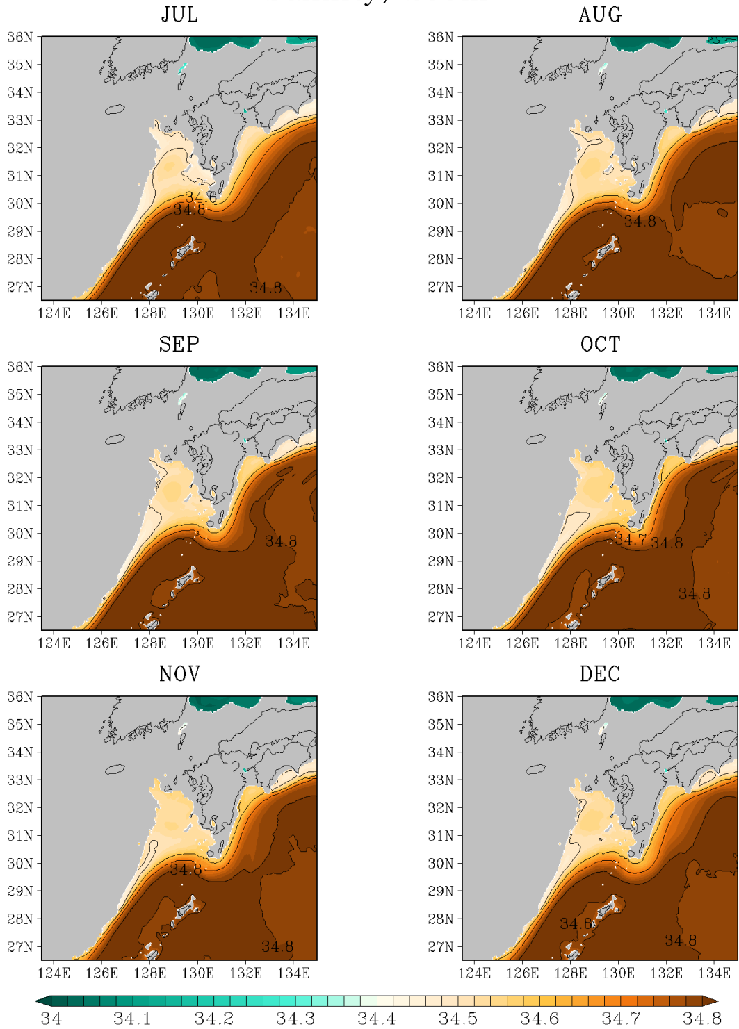
図G - 14 (続く) 200 m 深の塩分 (unitless)
