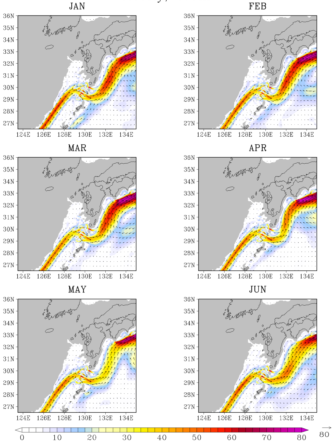
図 G - 25 400 m 深の流速 (cm/s)
