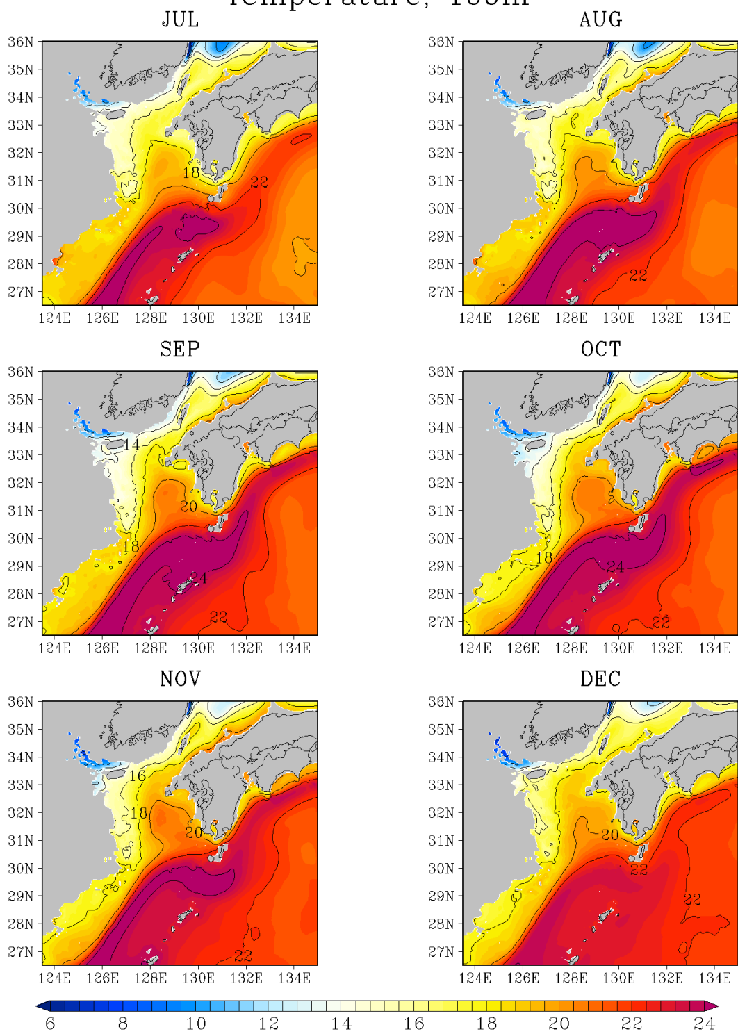
図G - 3 (続く) 100 m 深の水温 (°C)
