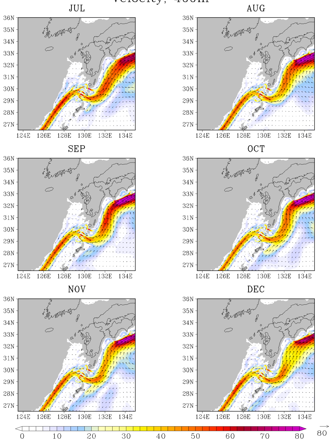
図 G - 25 (続く) 400 m 深の流速 (cm/s)
