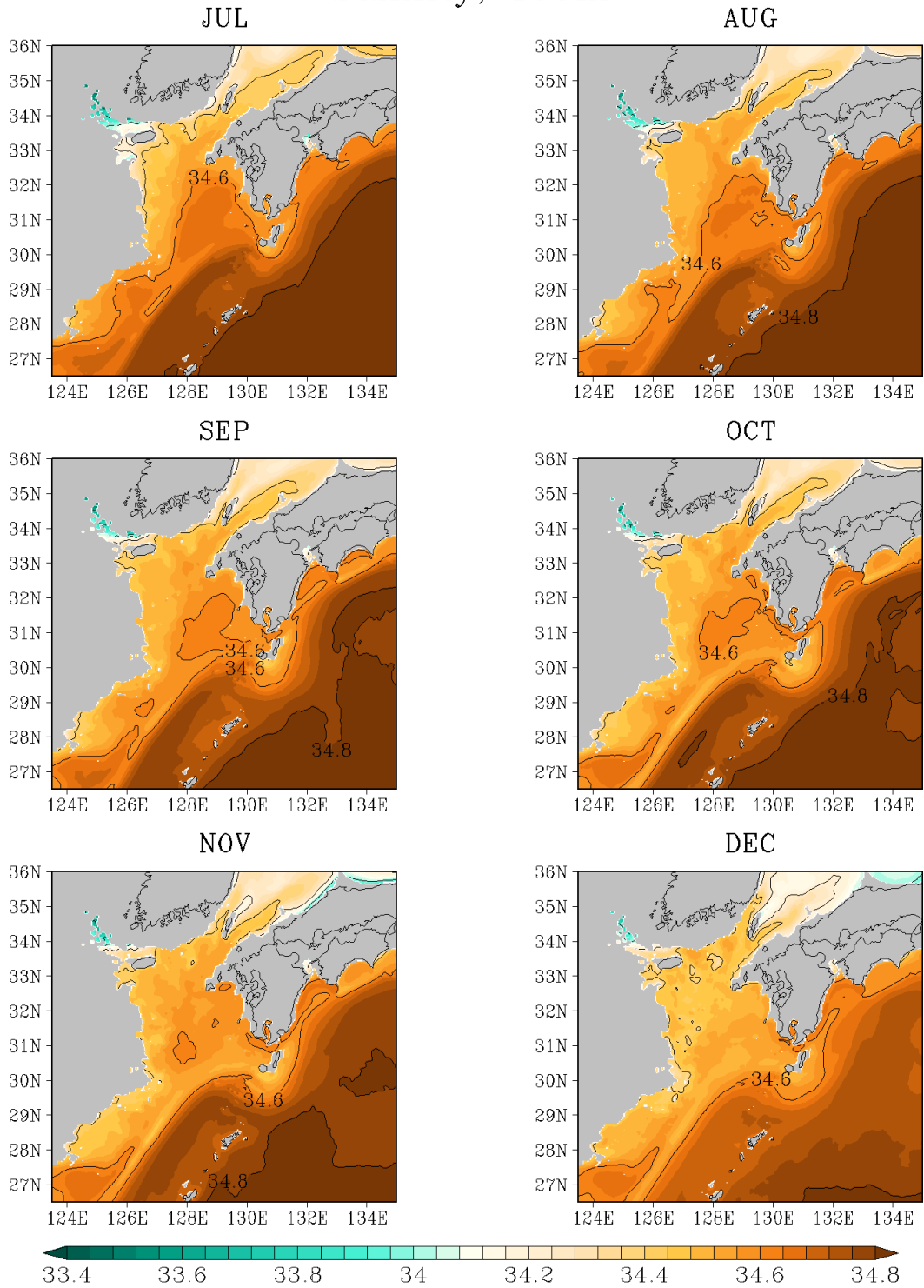
図G - 13 (続く) 100 m 深の塩分 (unitless)
