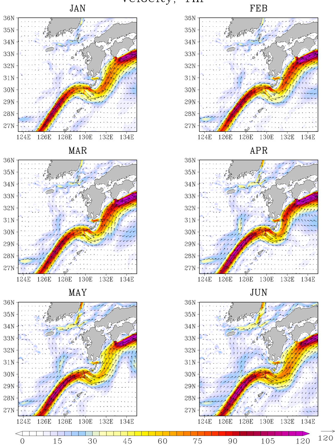
図 G - 21 1 m 深の流速 (cm/s)
