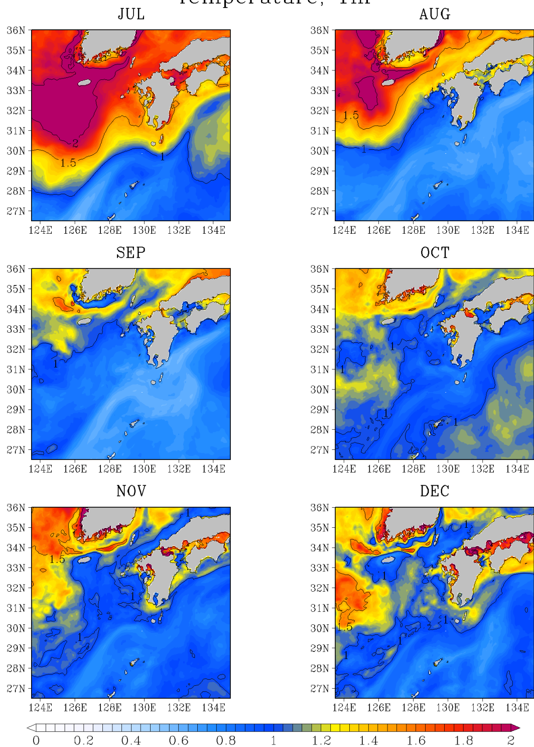
図G - 6 (続く) 1 m 深の水温 標準偏差 (°C)
