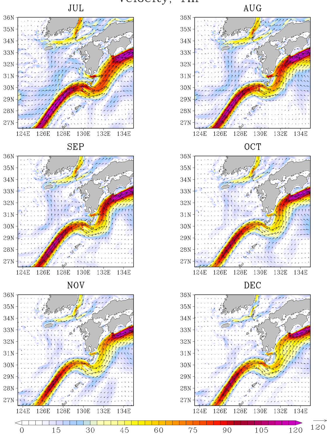
図 G - 21 (続く) 1 m 深の流速 ( cm/s )
