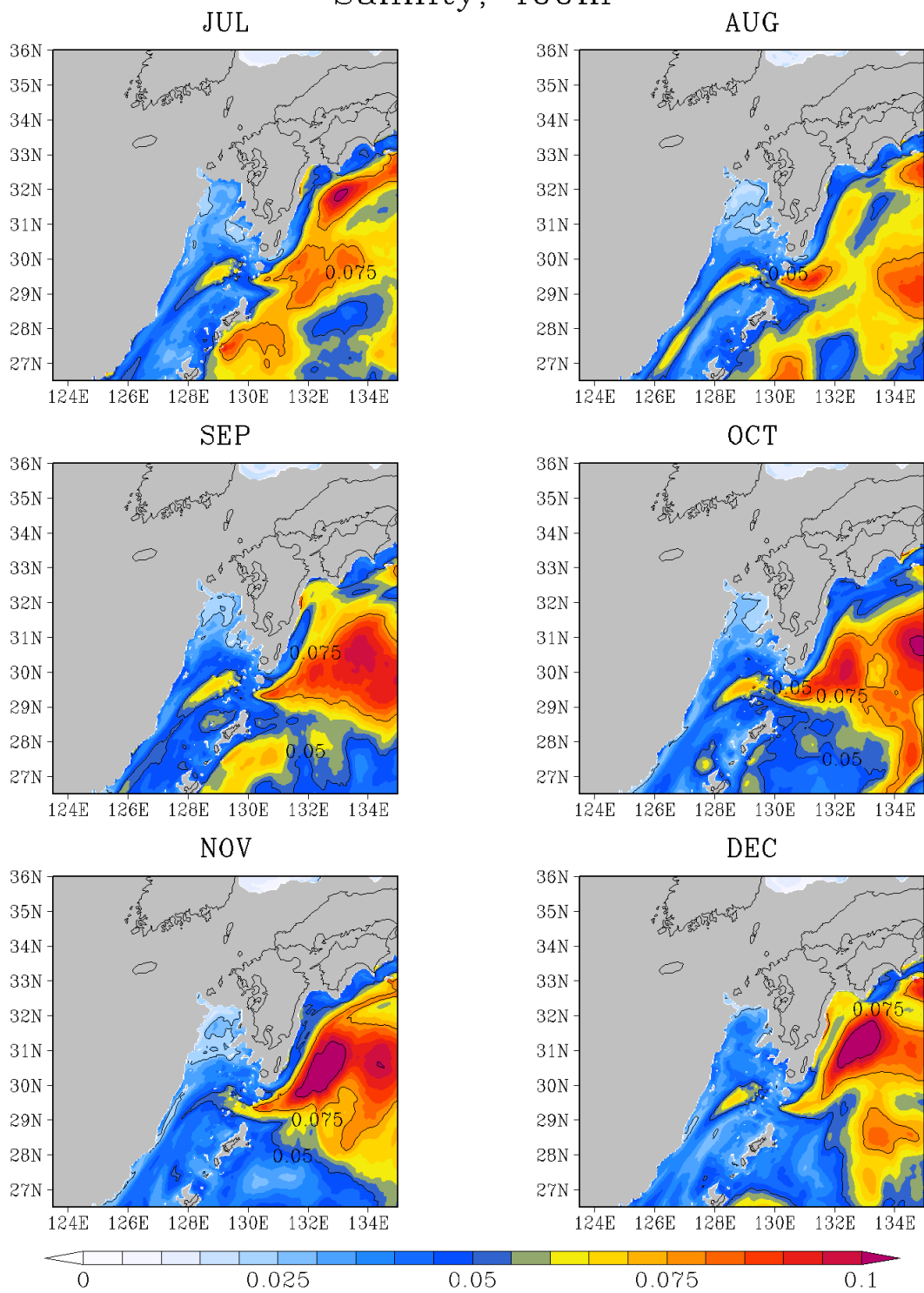
図G - 20 (続く) 400 m 深の塩分 標準偏差 (unitless)
