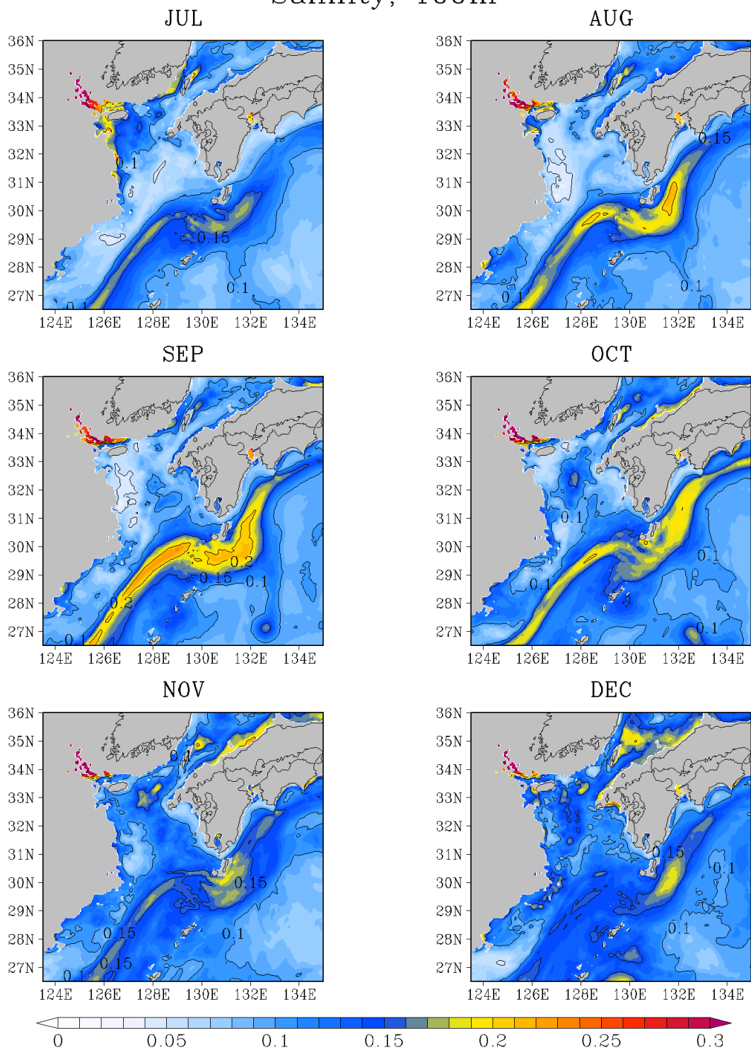
図G - 18 (続く) 100 m 深の塩分 標準偏差 (unitless)
