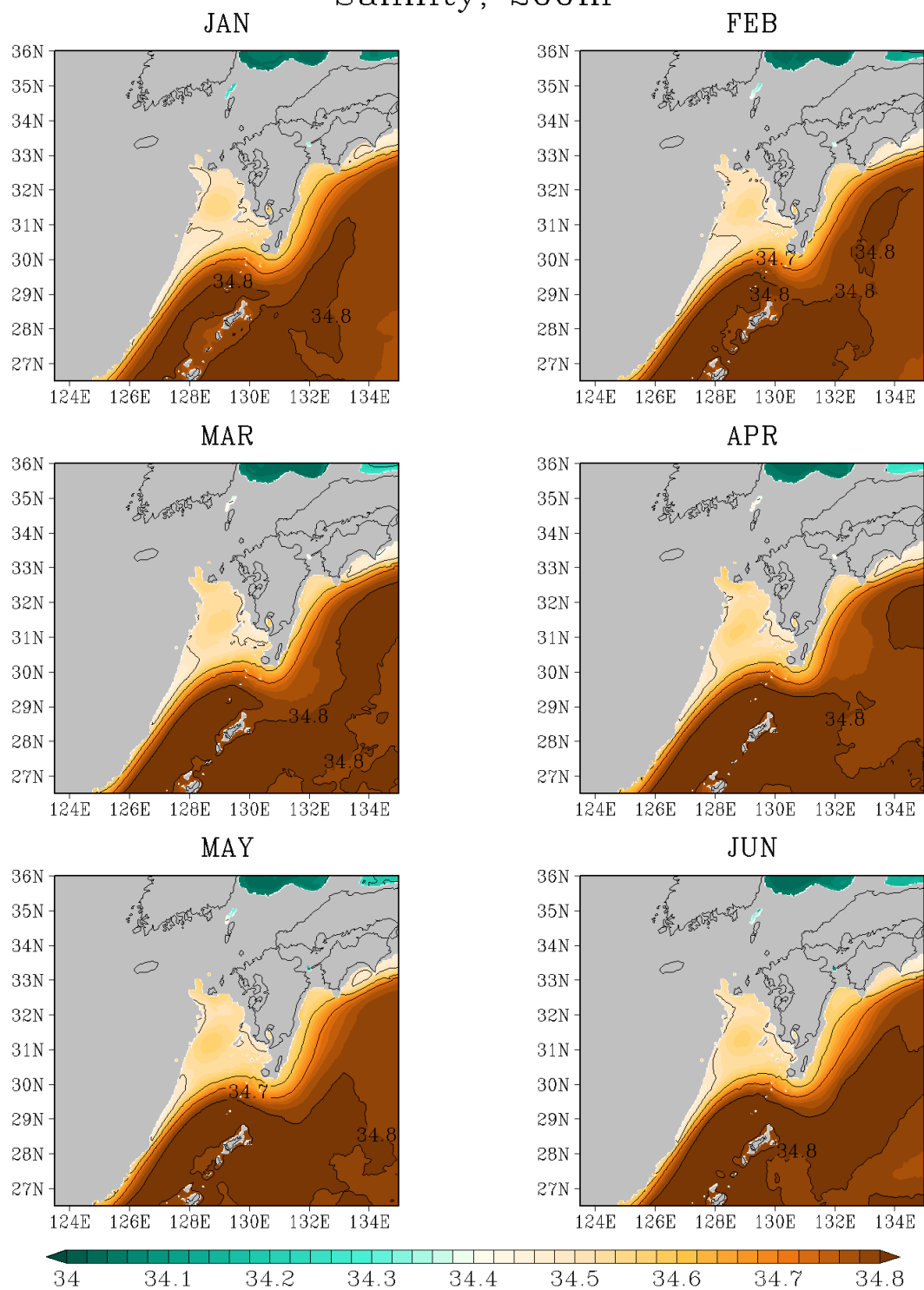
図 G - 14 200 m 深の塩分 (unitless)
