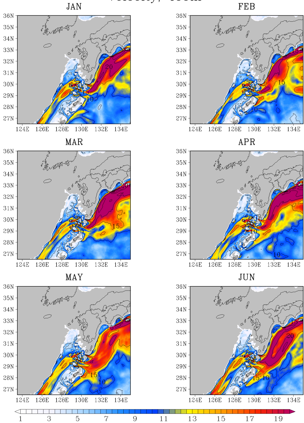
図G - 30 400 m 深の流速 標準偏差 (cm/s)
