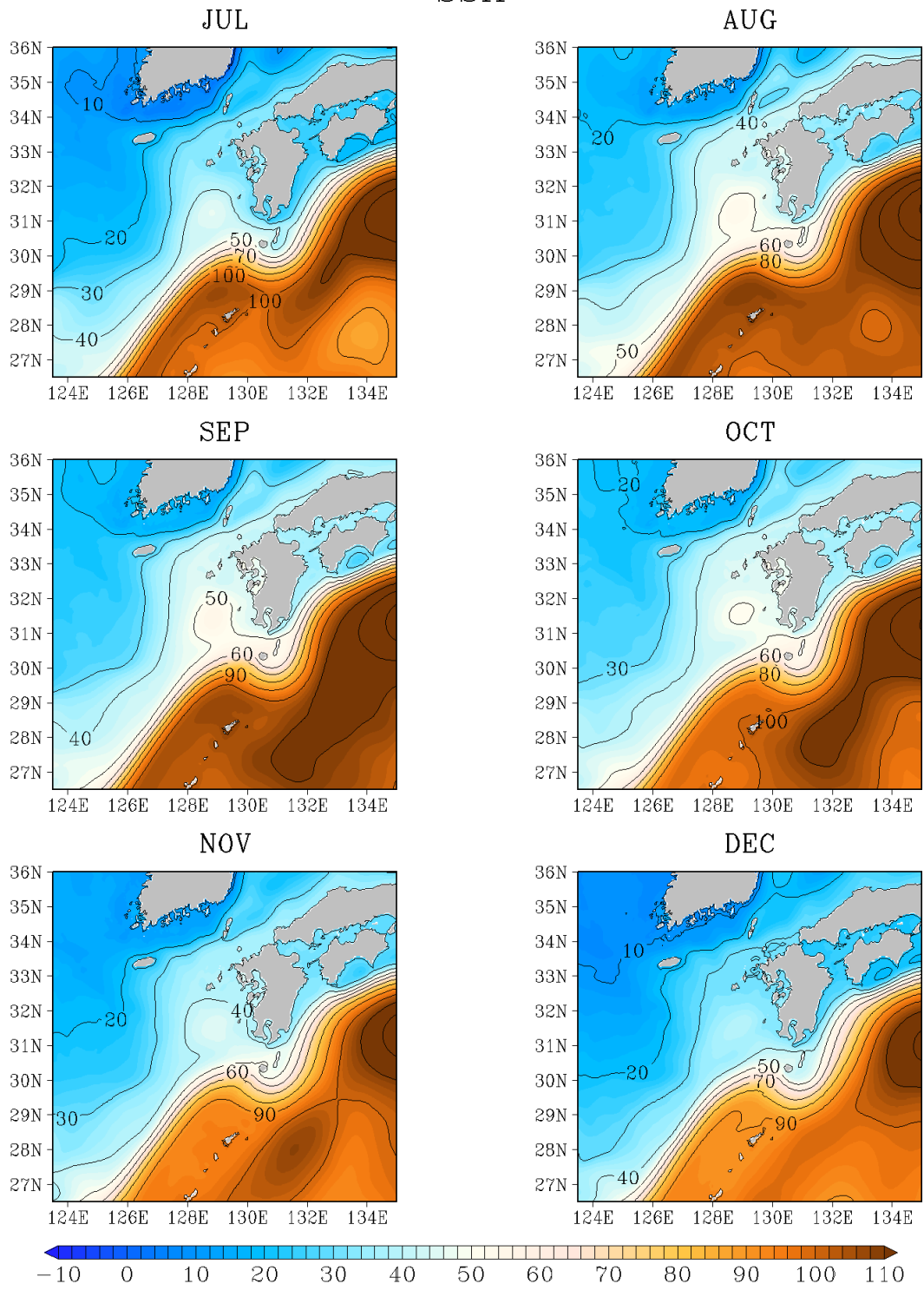
図 G - 31 (続) 海面水位 (cm)
