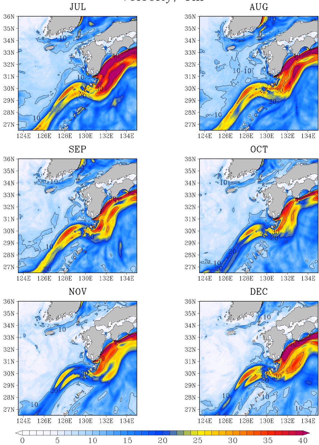
図G - 26 (続く) 1 m 深の流速 標準偏差 (cm/s)
