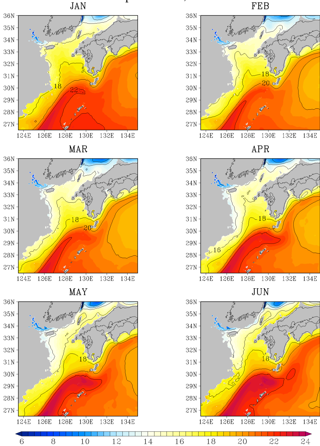
図 G - 3 100 m 深の水温 (°C)
