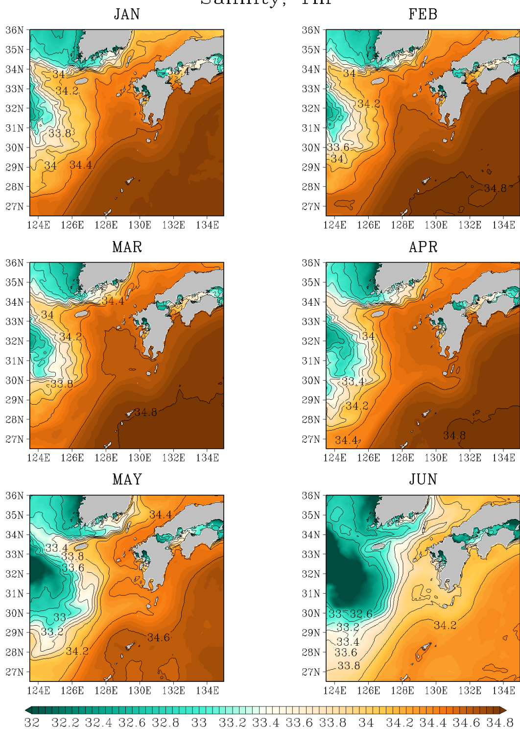
図 G - 11 1 m 深の塩分 (unitless)
