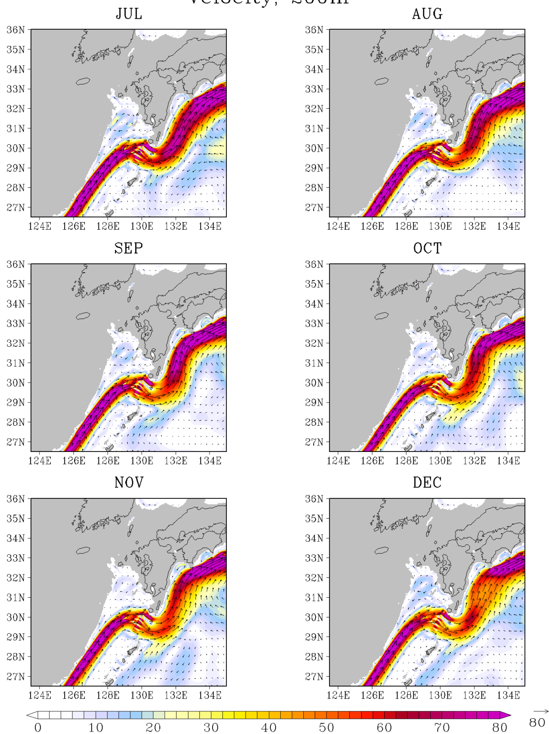
図 G - 24 (続く) 200 m 深の流速 (cm/s)
