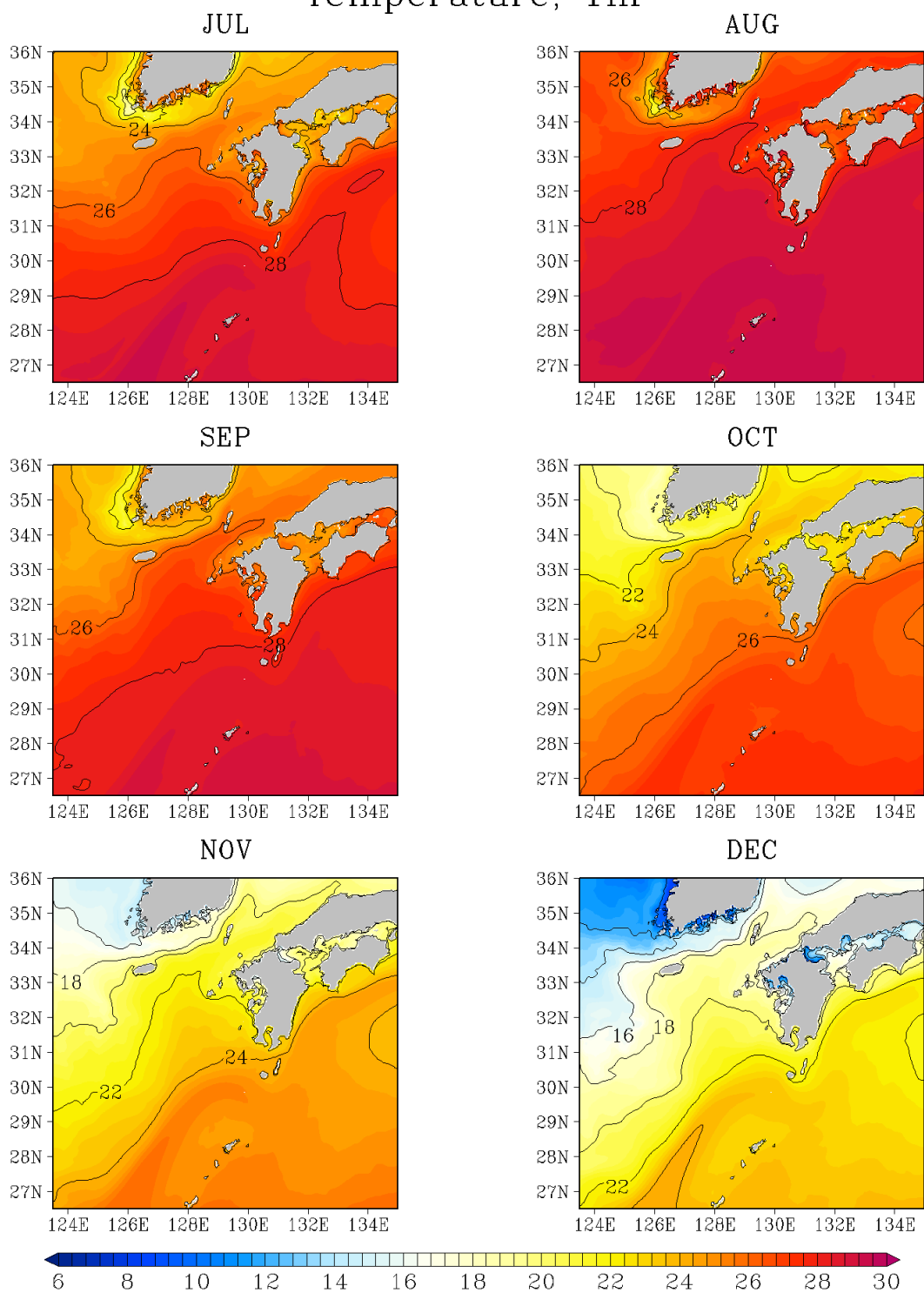
図G - 1 (続く) 1 m 深の水温 (°C)
