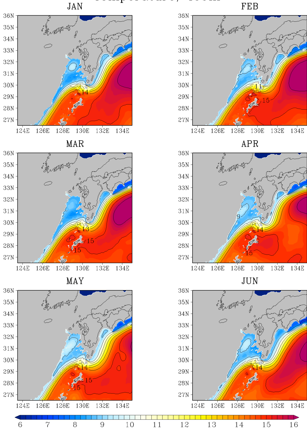
図 G - 5 400 m 深の水温 (°C)
