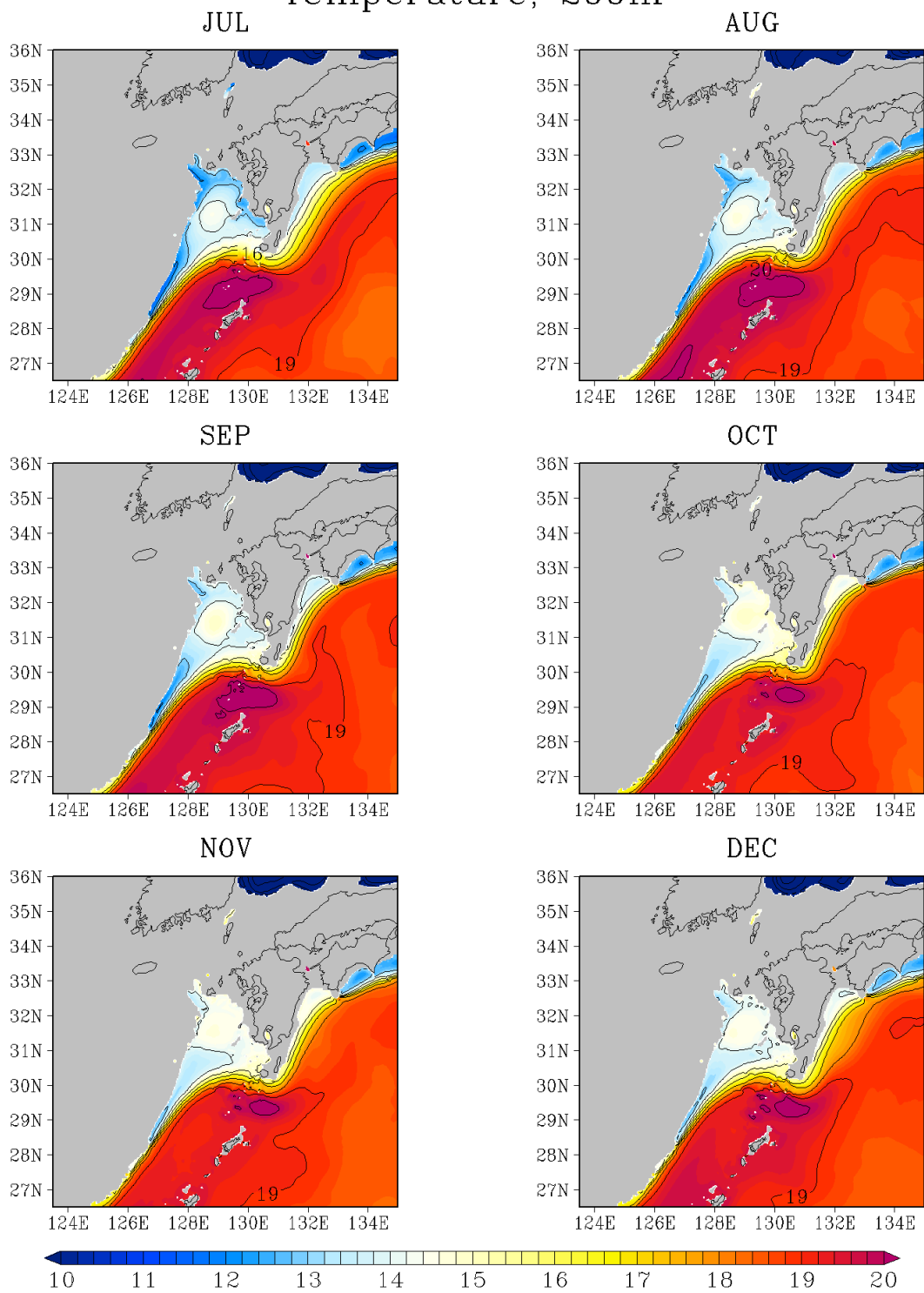
図G - 4 (続く) 200 m 深の水温 (°C)
