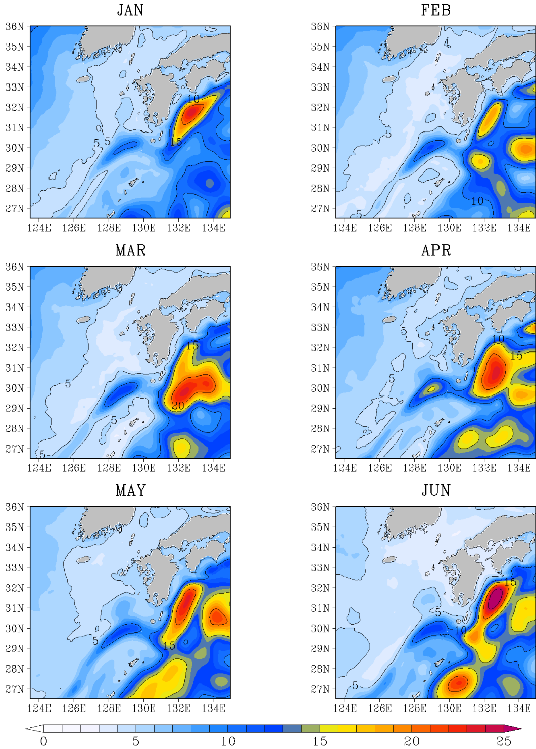
图 G - 32 海面水位 標準偏差 (cm)
