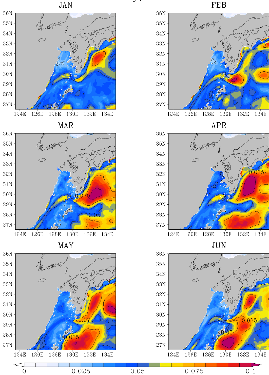
図G - 20 400 m 深の塩分 標準偏差 (unitless)
