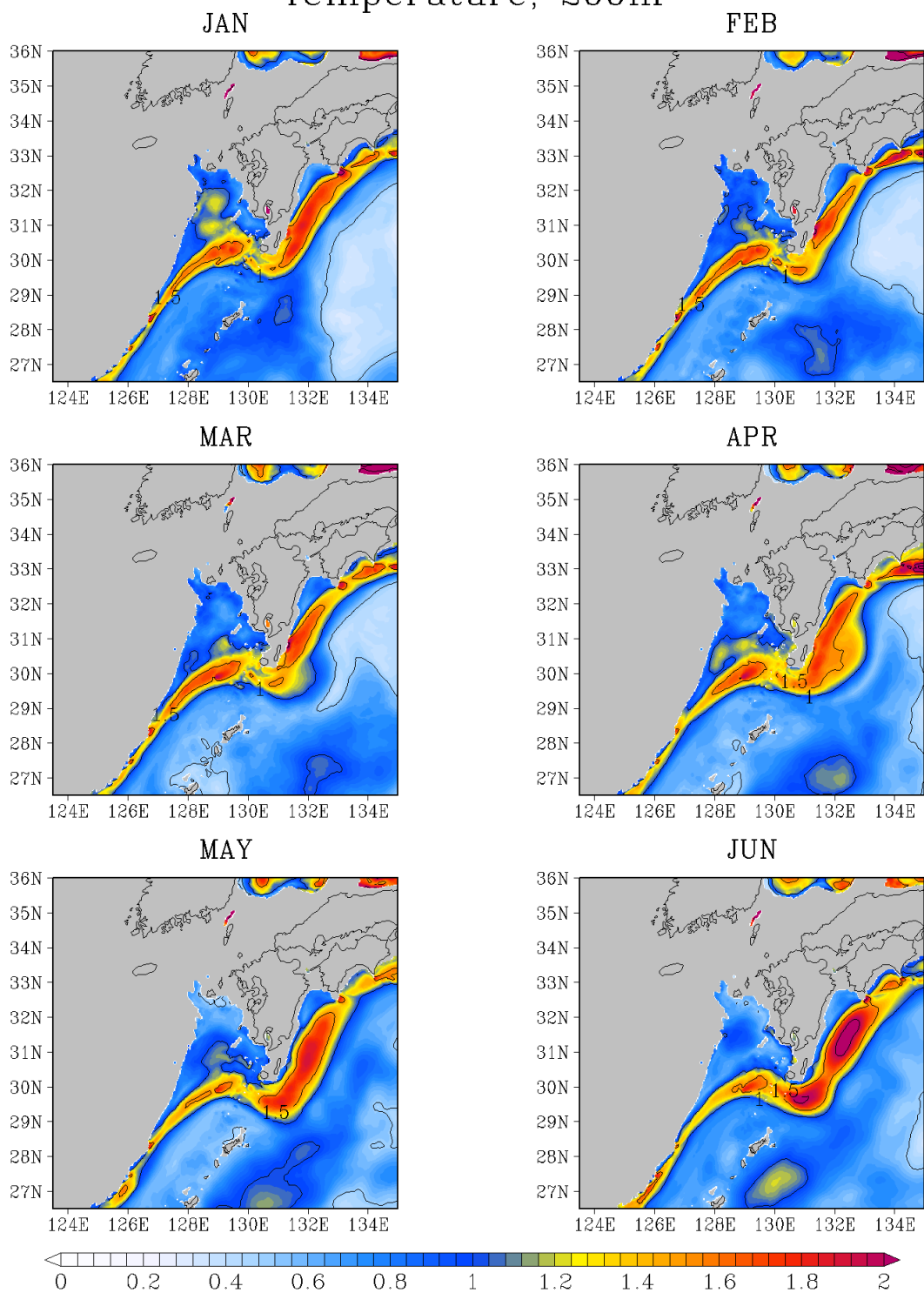
図 G - 9 200 m 深の水温 標準偏差 (°C)
