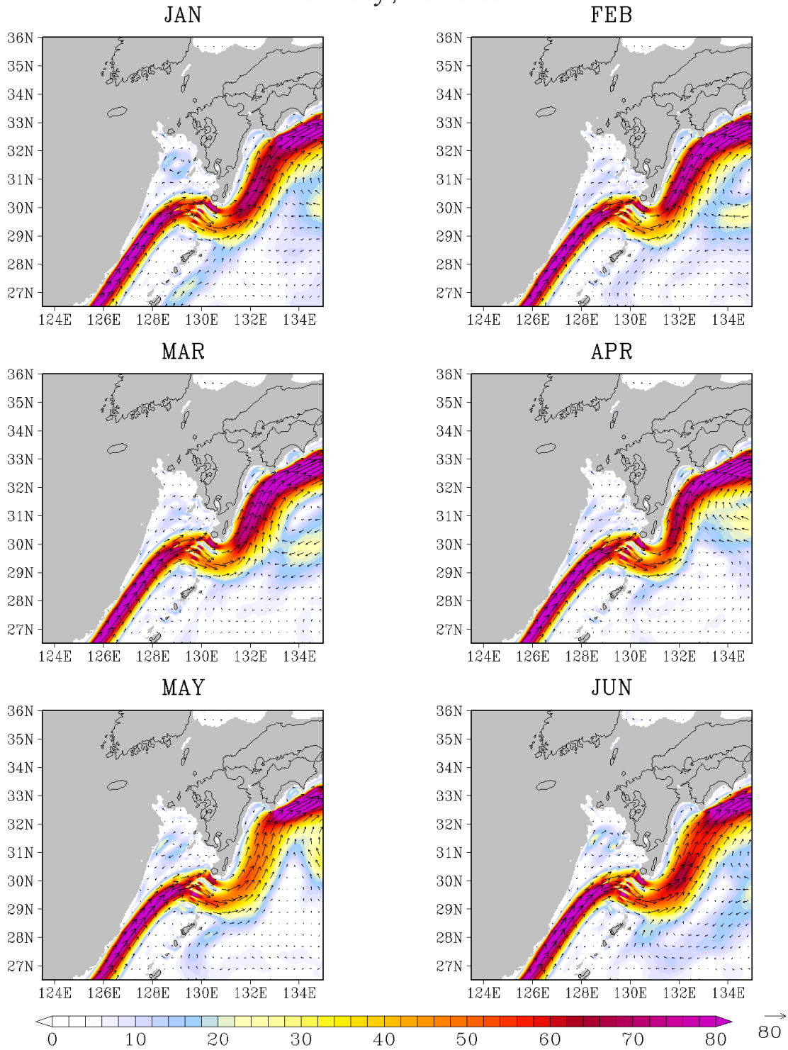
図 G - 24 200 m 深の流速 (cm/s)
