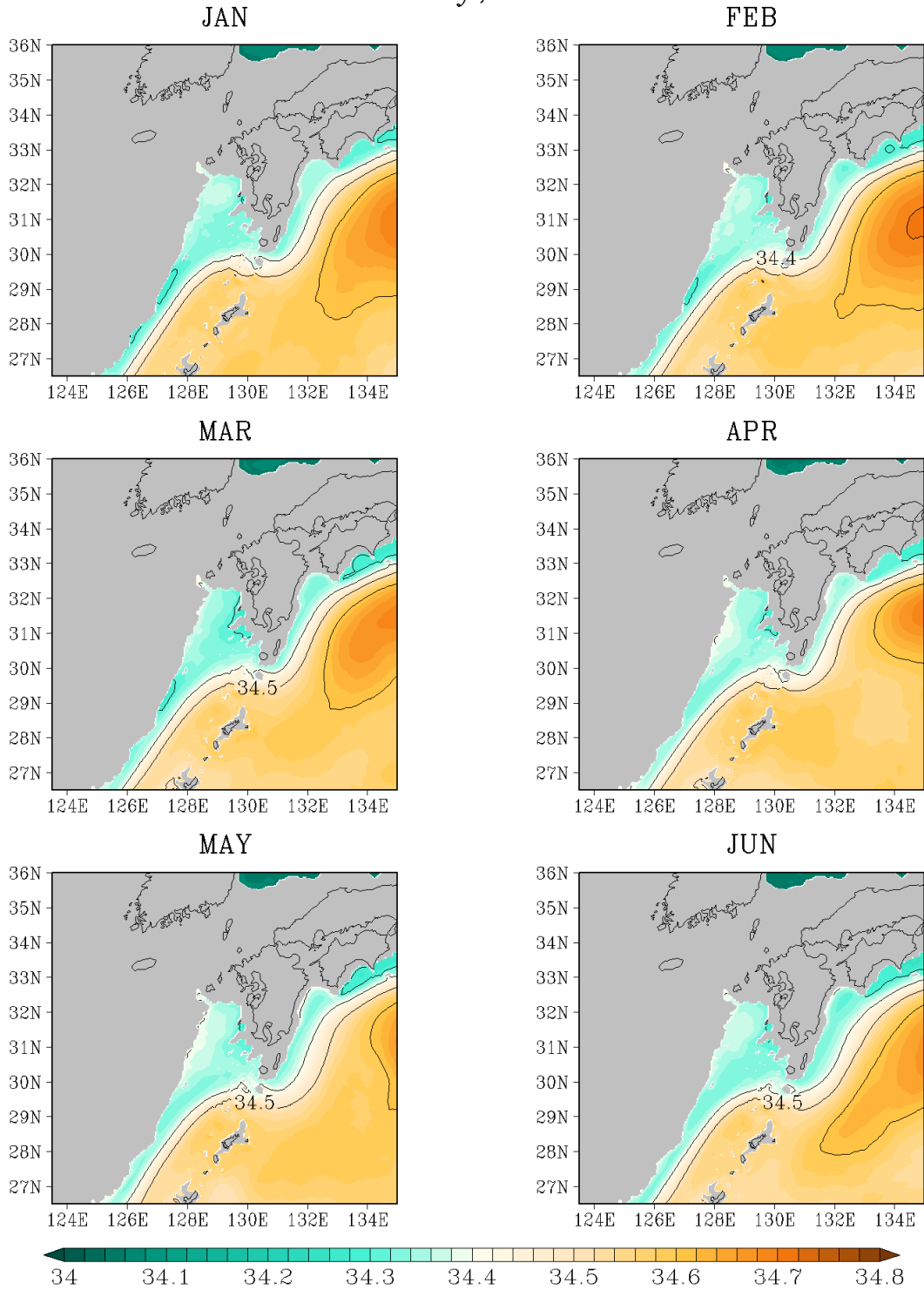
図 G - 15 400 m 深の塩分 (unitless)
