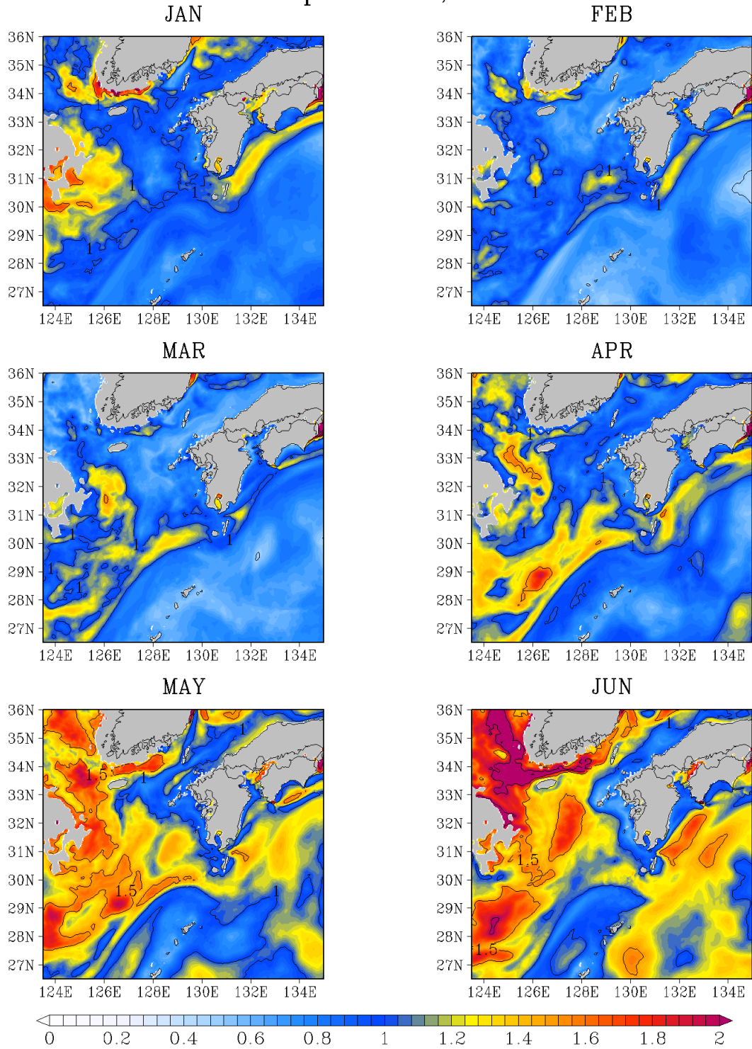
図G - 7 50 m 深の水温 標準偏差 (°C)
