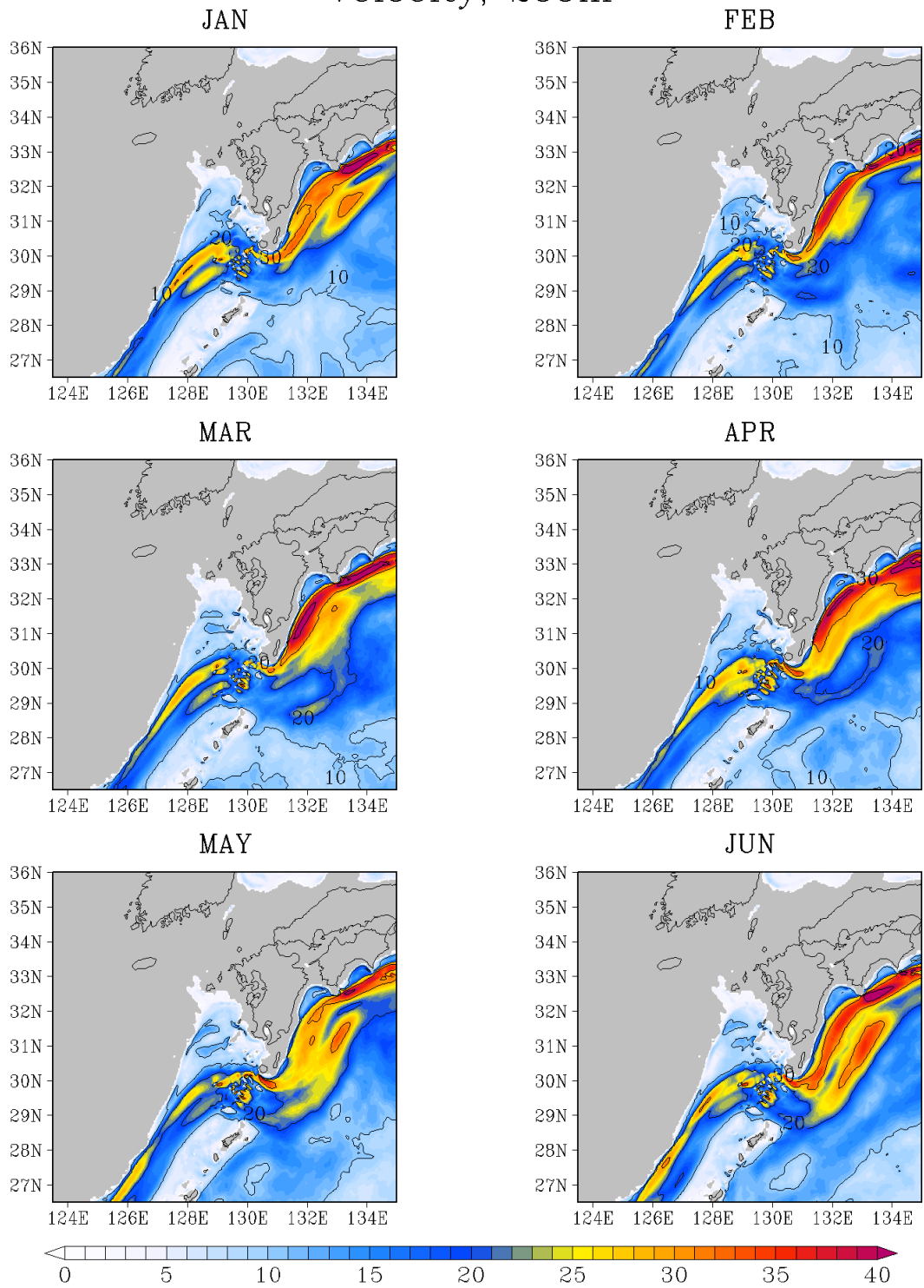
図G - 29 200 m 深の流速 標準偏差 (cm/s)
