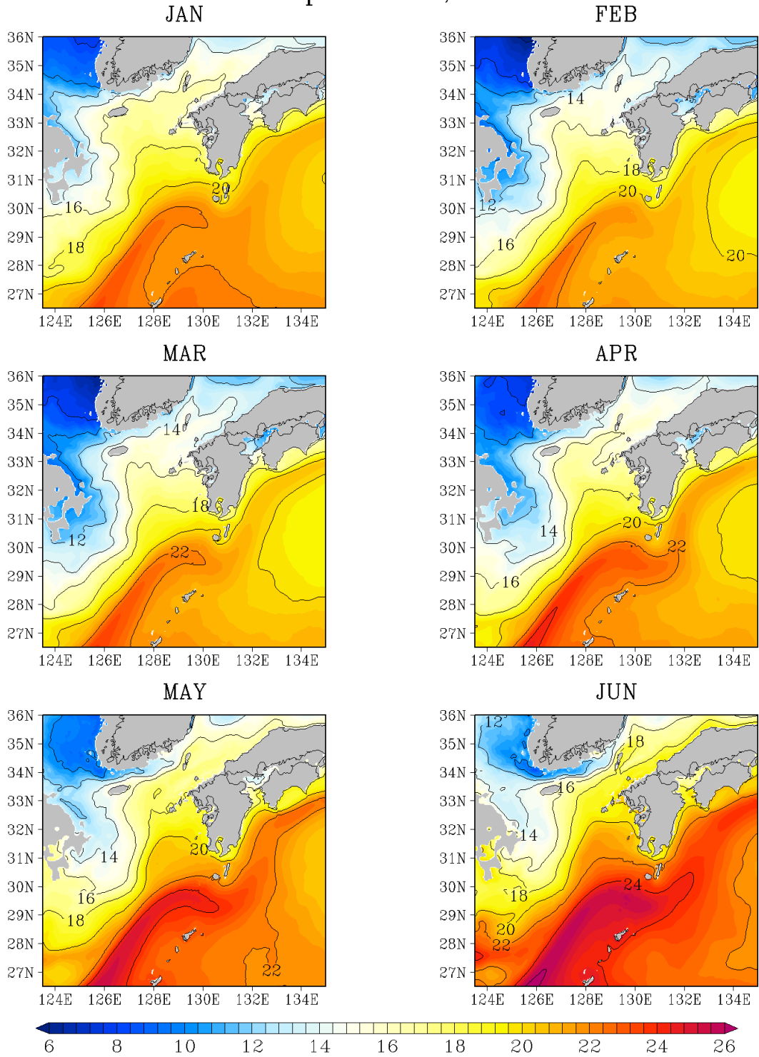
図G-2 50 m 深の水温 (°C)
