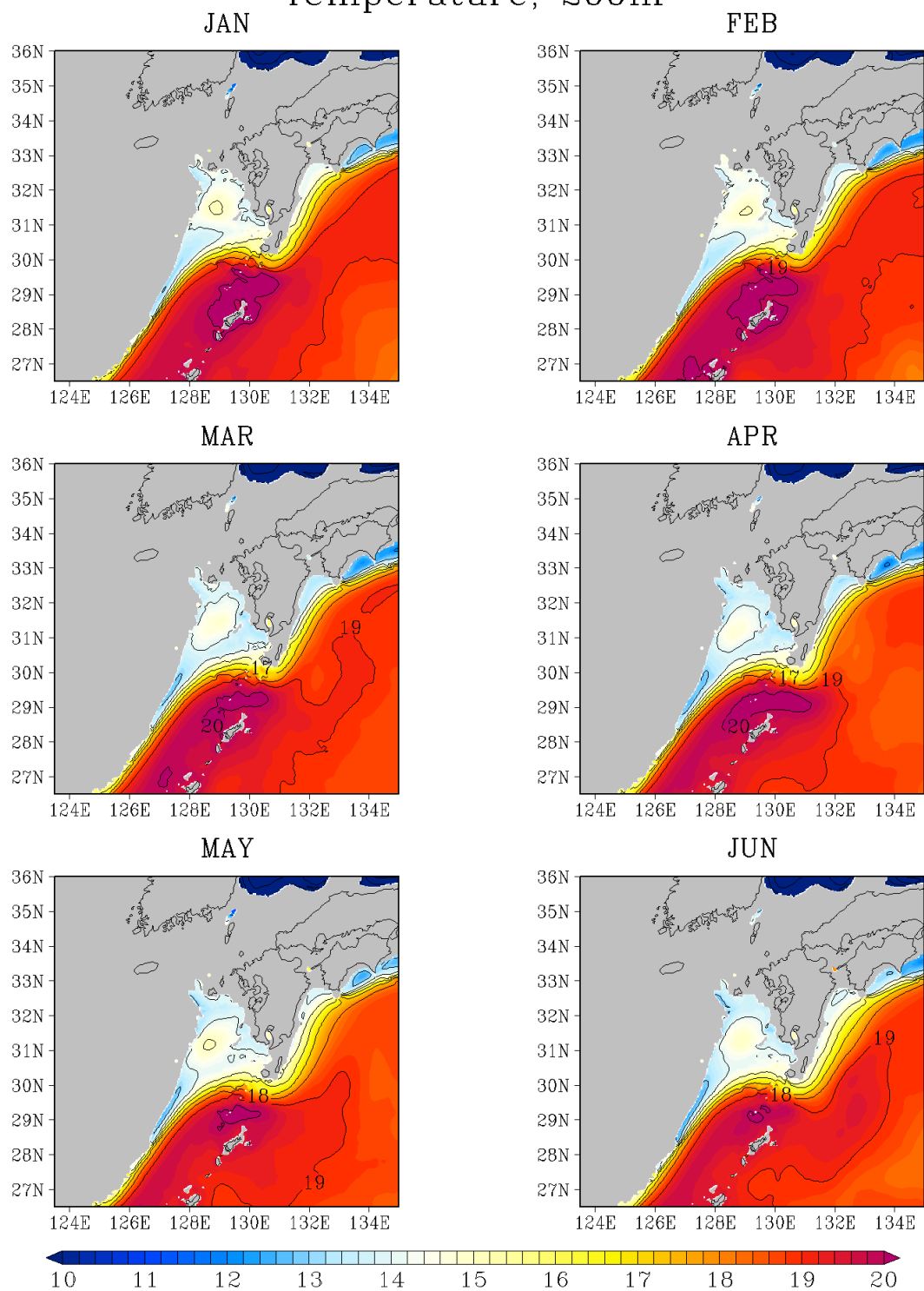
図 G - 4 200 m 深の水温 (°C)
