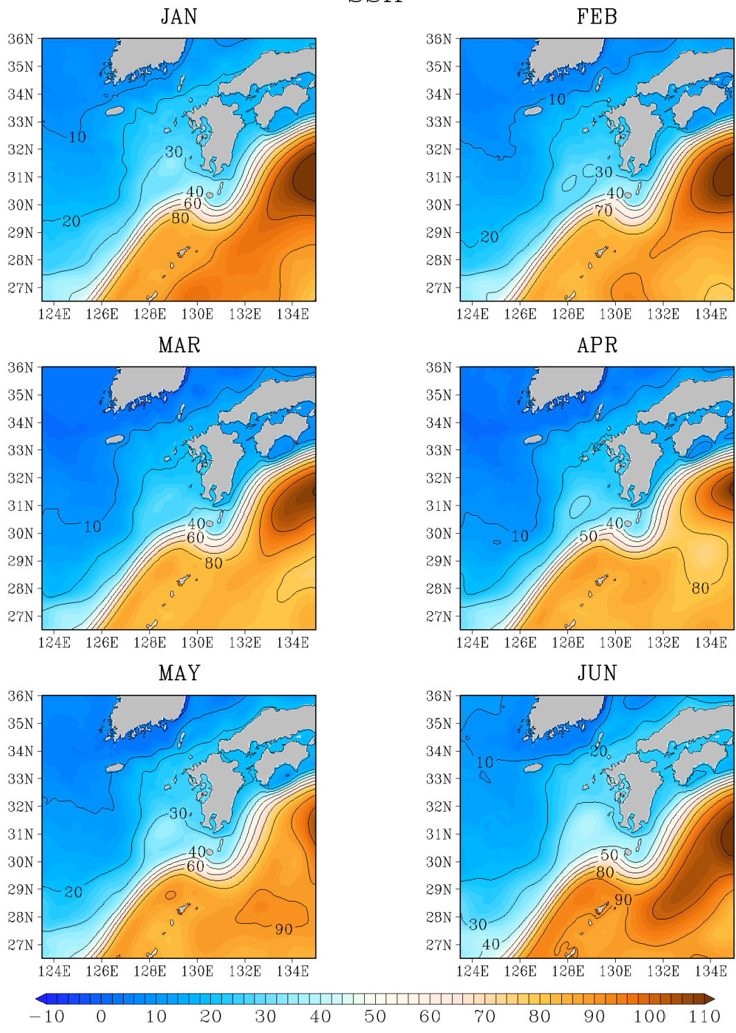
图 G - 31 海面水位 (cm)
