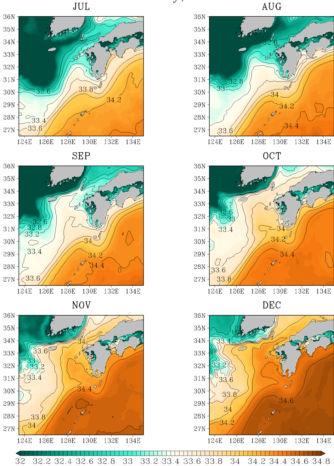
図G - 11 (続く) 1 m 深の塩分 (unitless)
