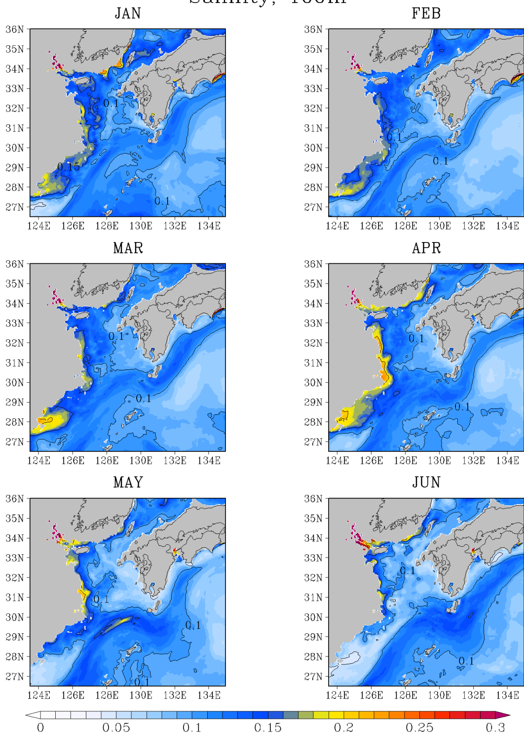
図G - 18 100 m 深の塩分 標準偏差 (unitless)
