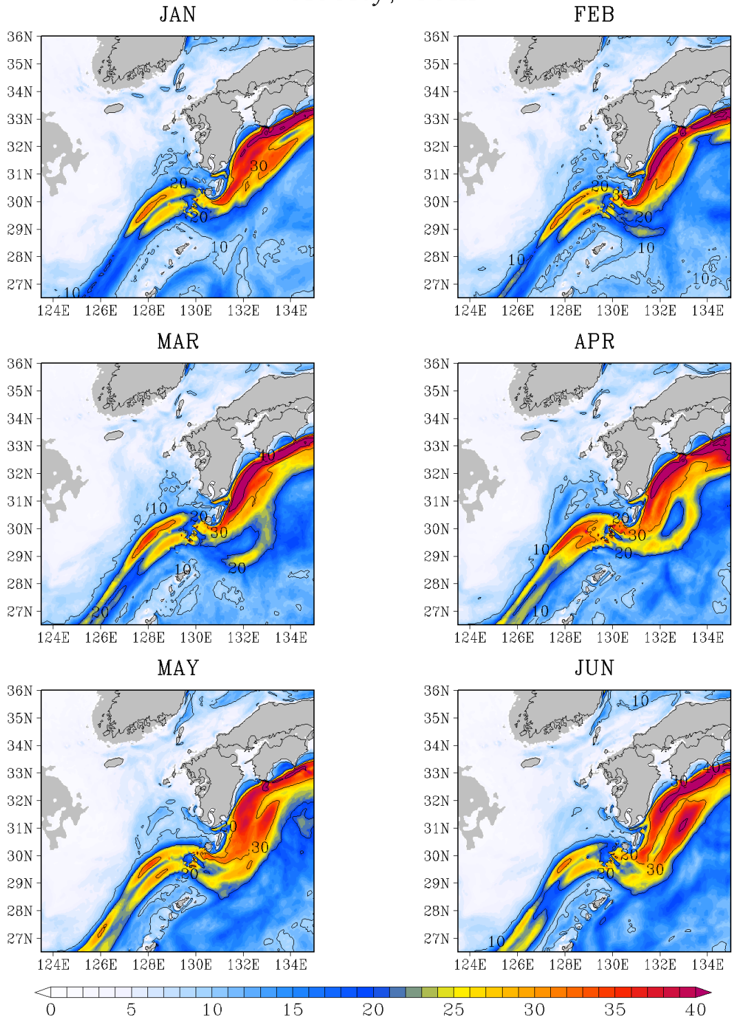
図 G - 27 50 m 深の流速 標準偏差 (cm/s)
