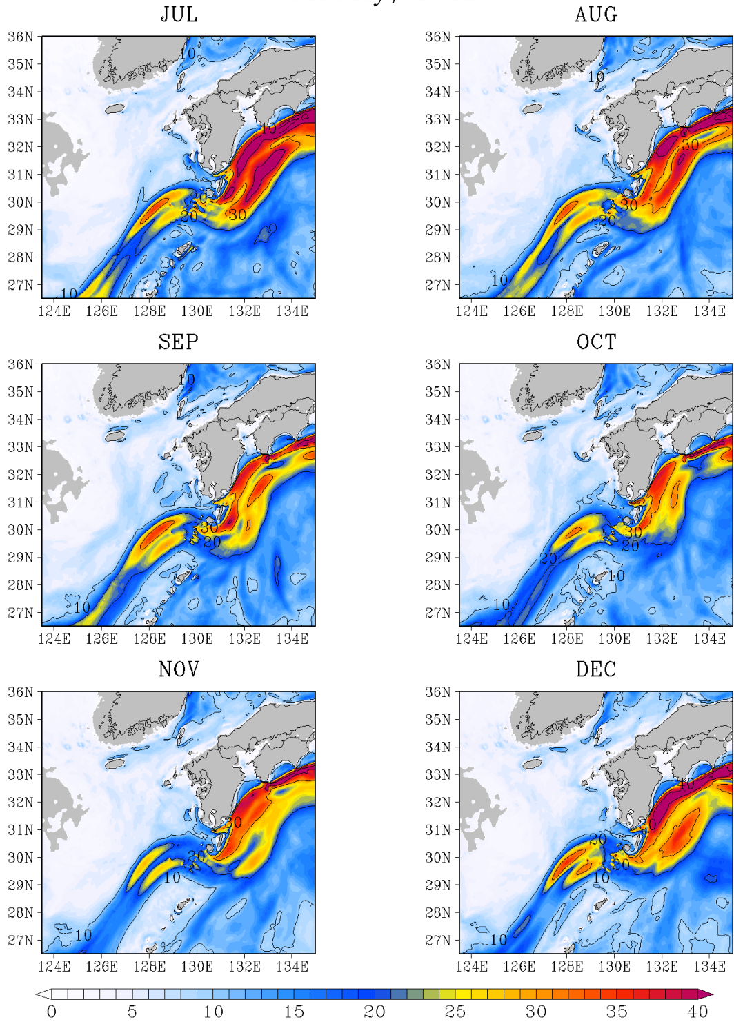
図 G - 27 (続く) 50 m 深の流速 標準偏差 (cm/s)
