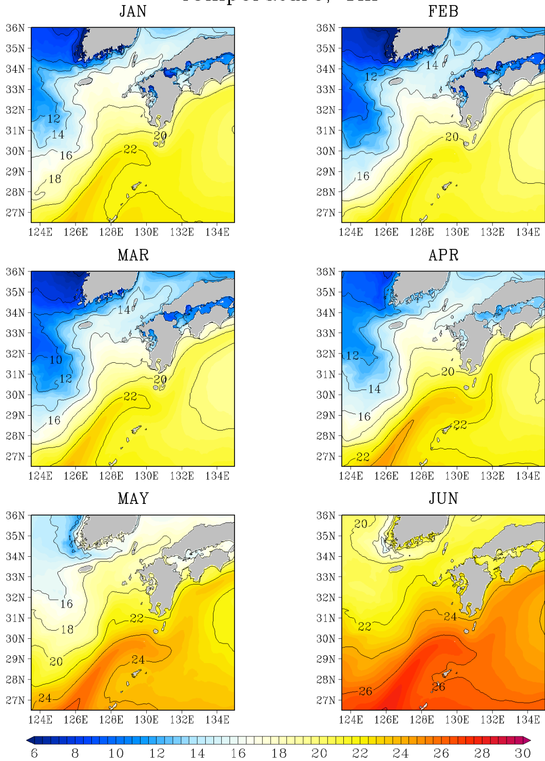
図 G - 1 1 m 深の水温 (°C)
