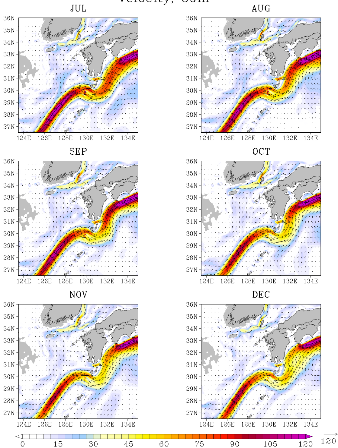
図G - 22 (続く) 50 m 深の流速 ( cm/s )
