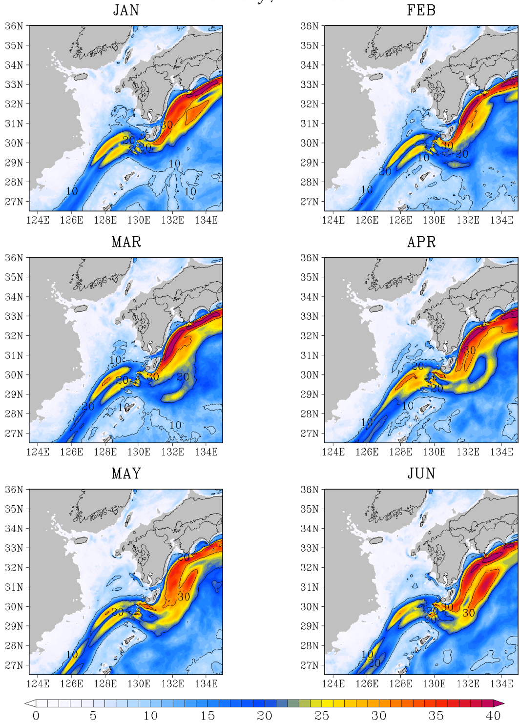
図G - 28 100 m 深の流速 標準偏差 ( cm/s )
