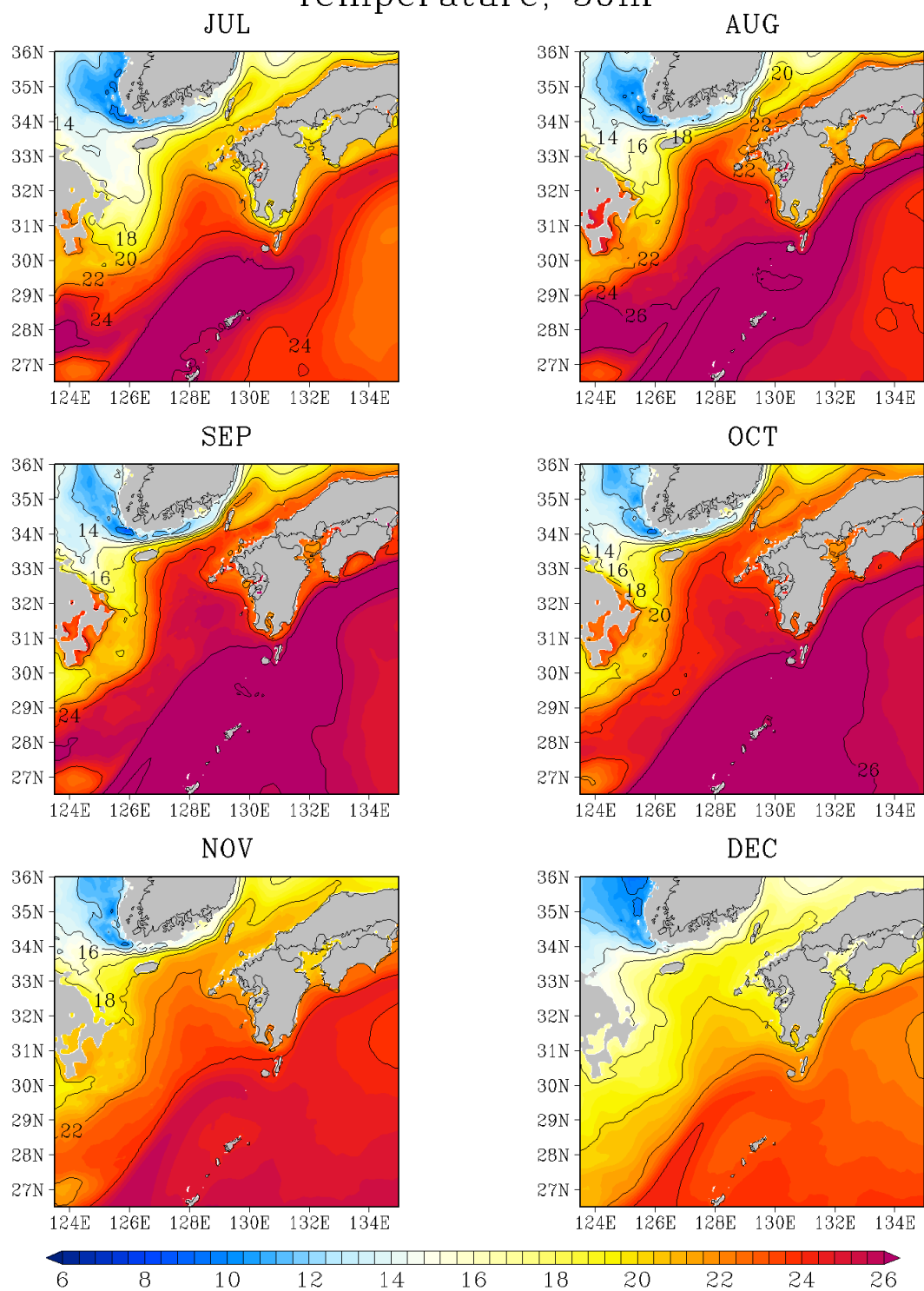
図G - 2 (続く) 50 m 深の水温 (°C)
