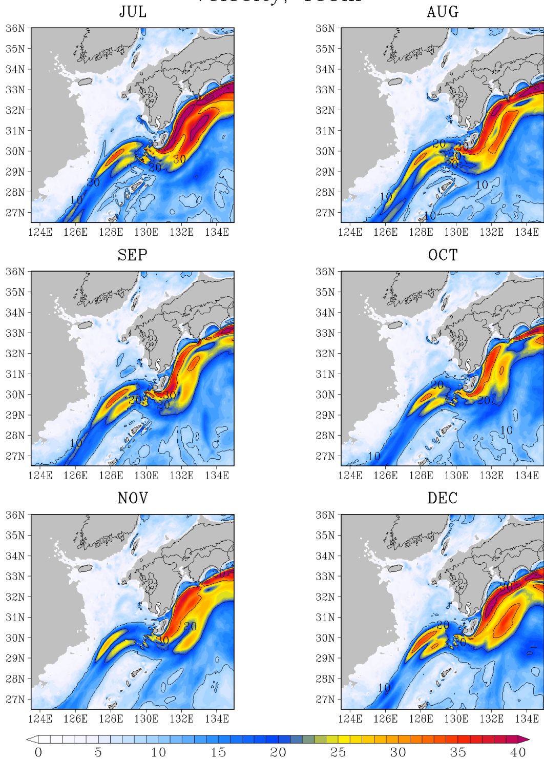
図G - 28 (続く) 100 m 深の流速 標準偏差 (cm/s)
