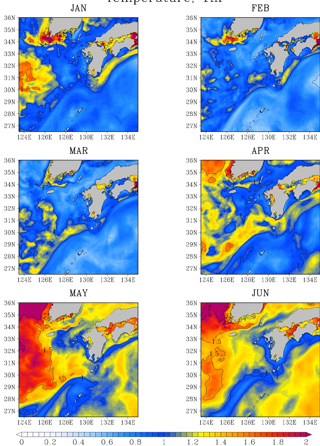
図G - 6 1 m 深の水温 標準偏差 (°C)
