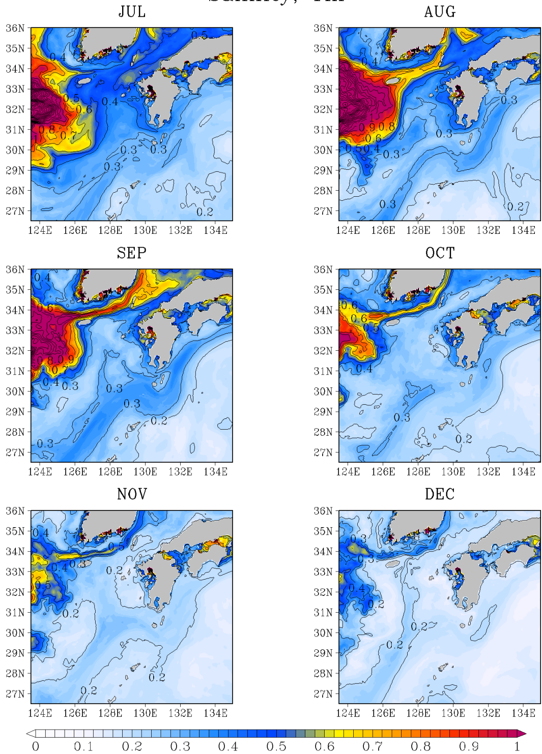
図G - 16 (続く) 1 m 深の塩分 標準偏差 (unitless)
