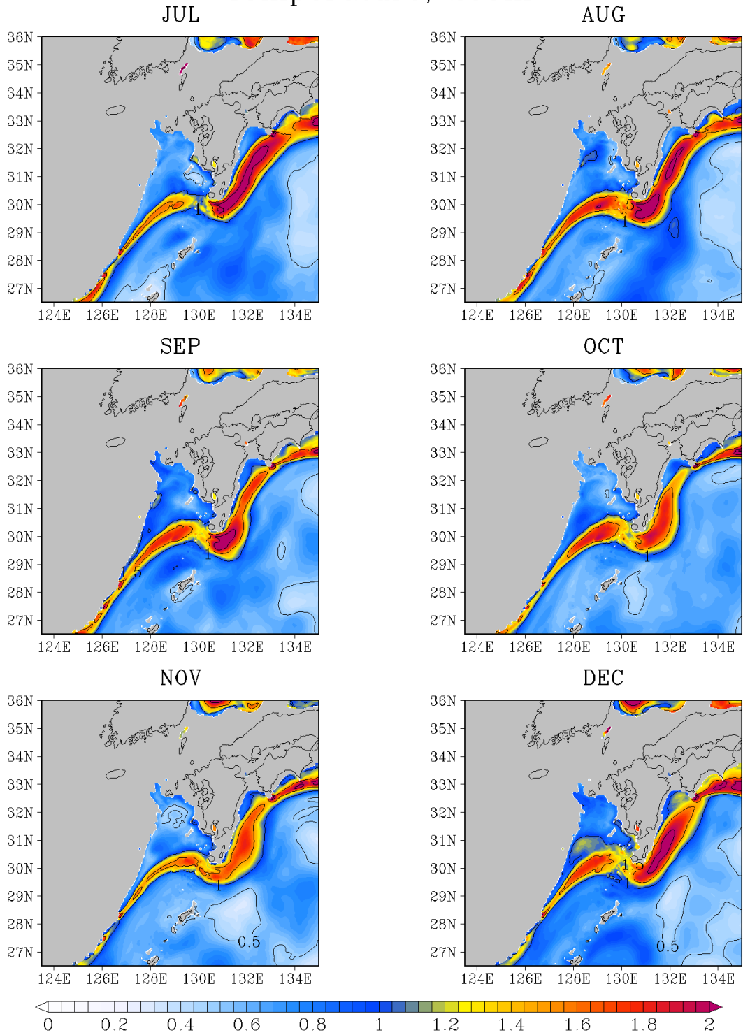
図 G - 9 (続く) 200 m 深の水溫 標準偏差 (°C)
