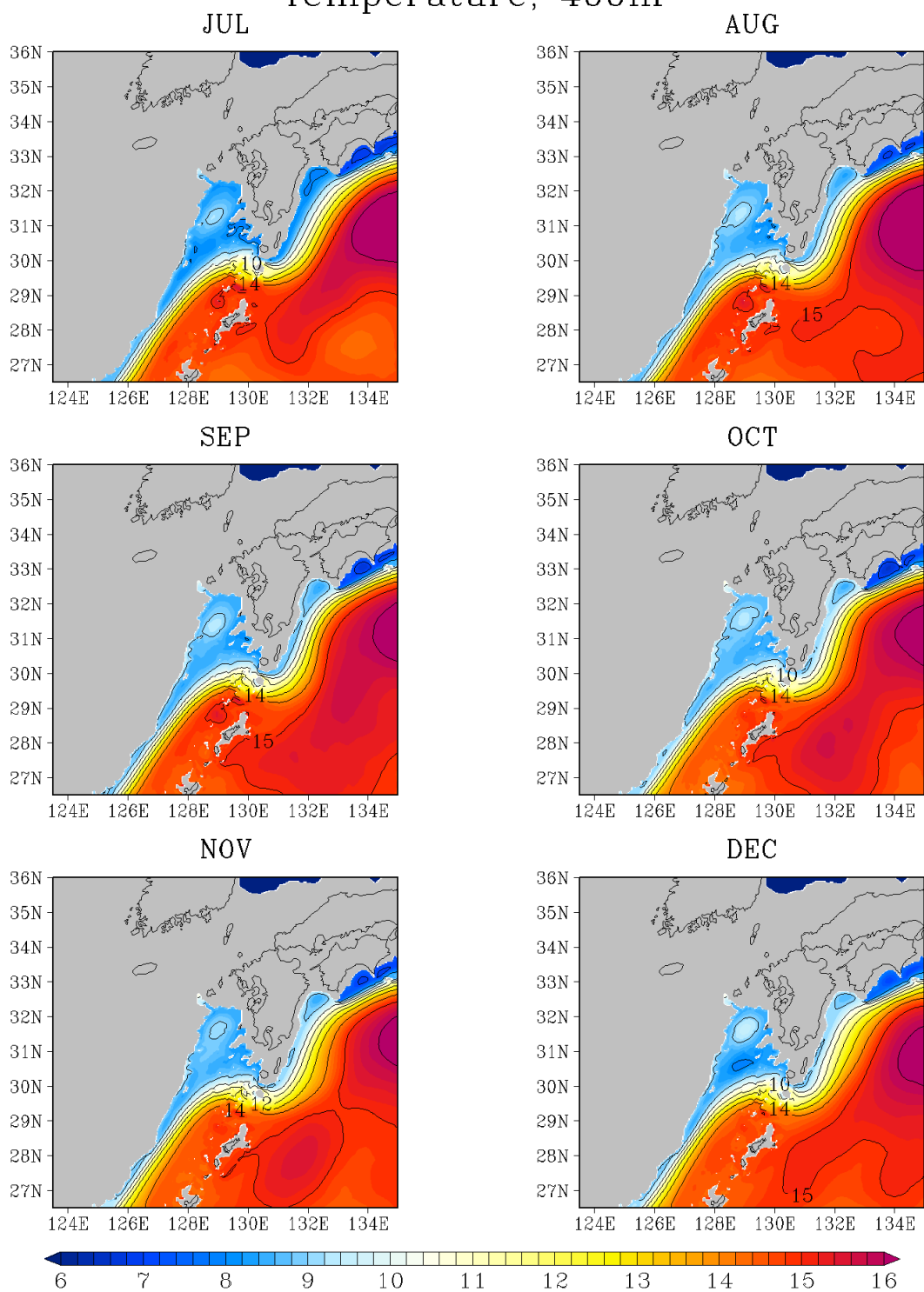
図G - 5 (続く) 400 m 深の水温 (°C)
