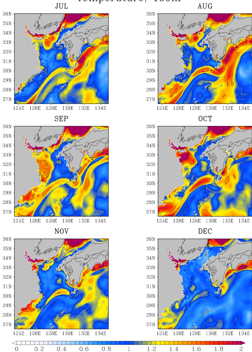
図G - 8 (続く) 100 m 深の水溫 標準偏差 (°C)
