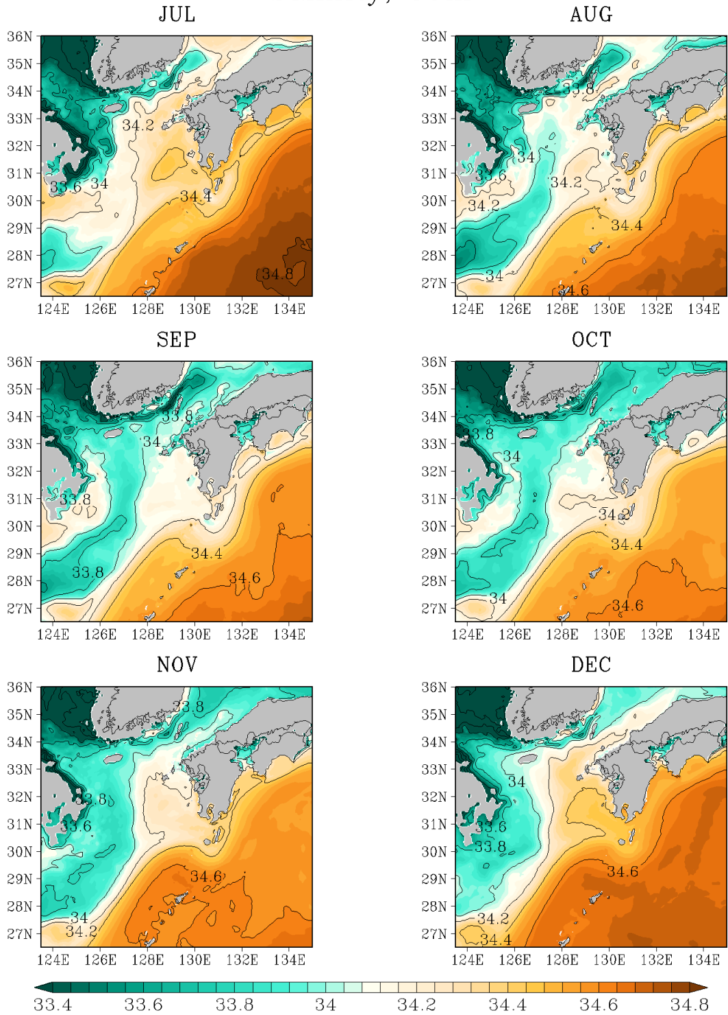
図G - 12 (続く) 50 m 深の塩分 (unitless)
