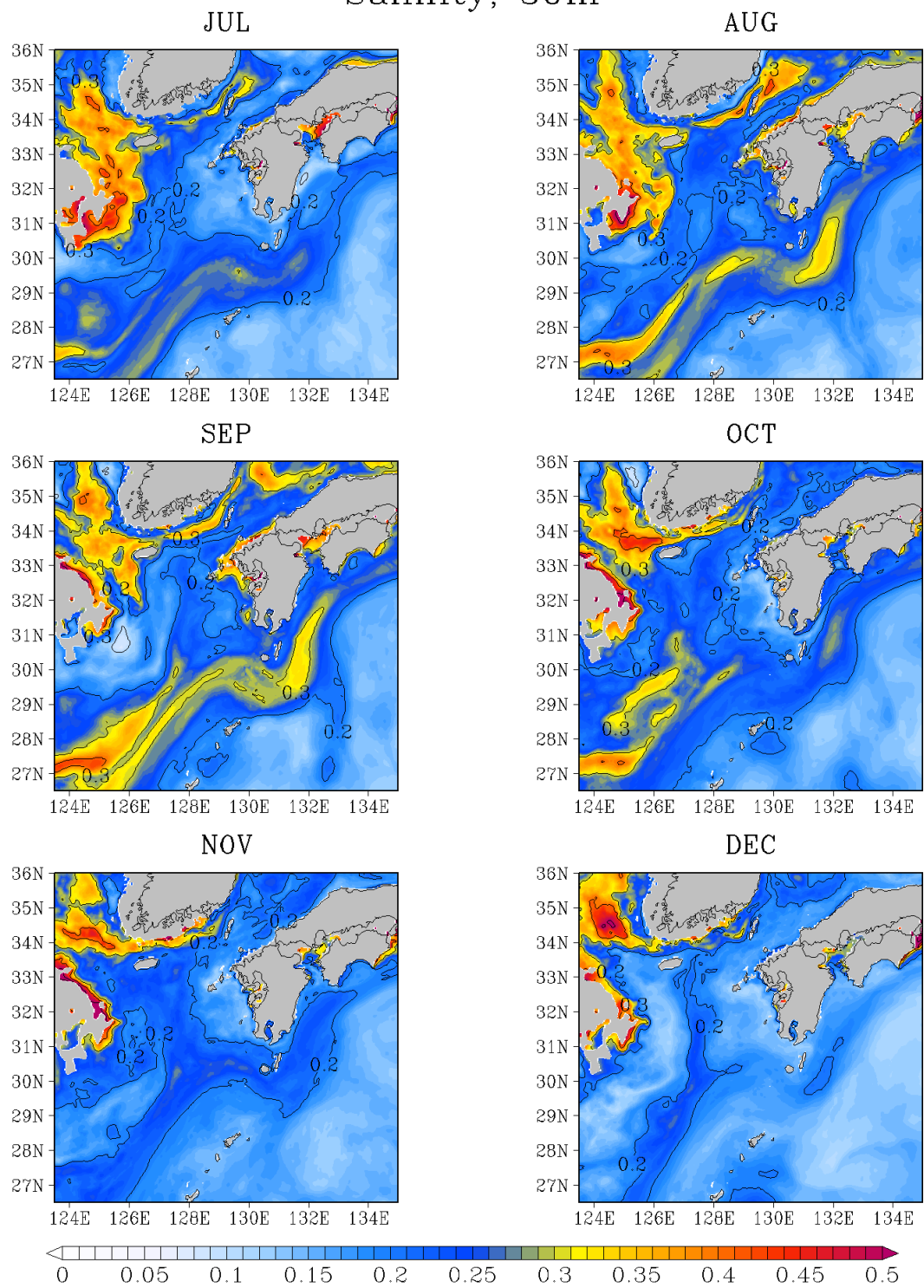
図 G - 17 (続く) 50 m 深の塩分 標準偏差 (unitless)
