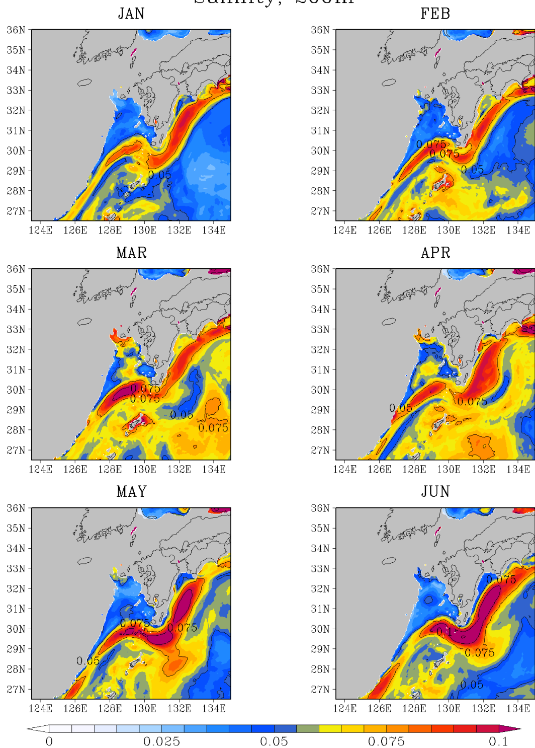
図G - 19 200 m 深の塩分 標準偏差 (unitless)
