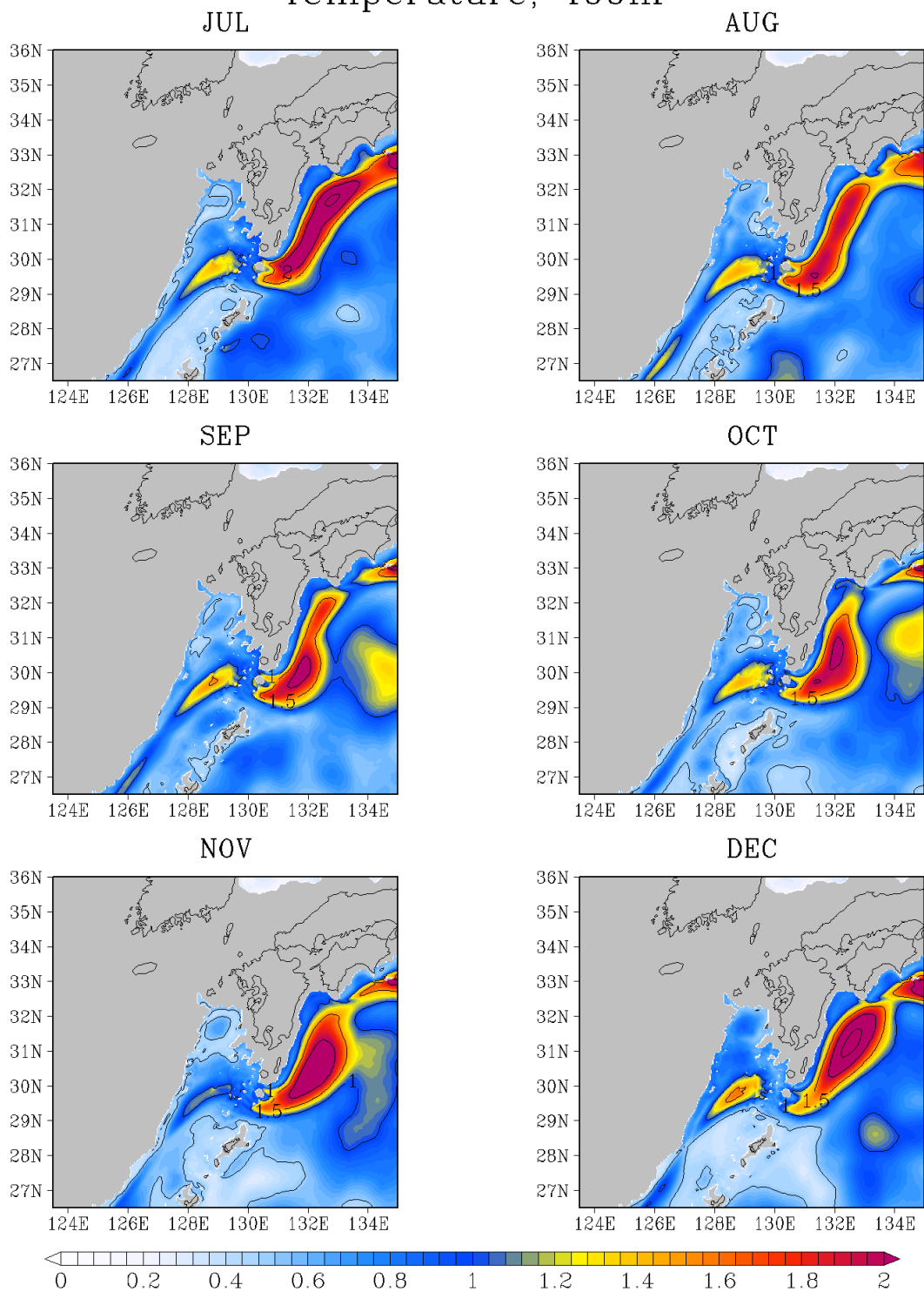
図G - 10 (続く) 400 m 深の水温 標準偏差 (°C)
