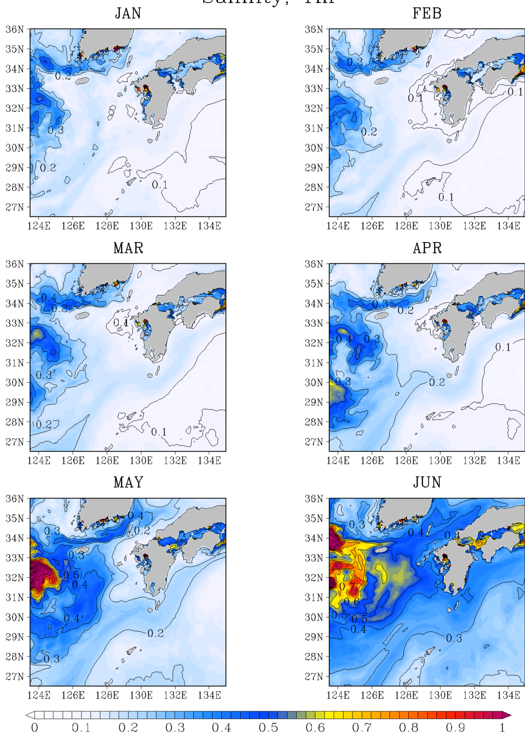
図G - 16 1 m 深の塩分 標準偏差 (unitless)
