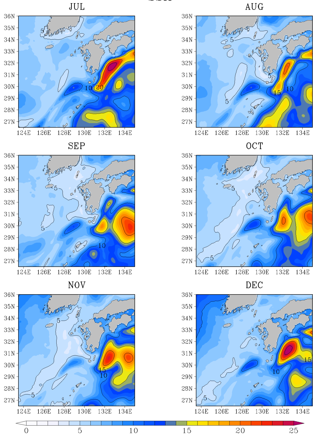
図 G - 32 (続く) 海面水位 標準偏差 (cm)
