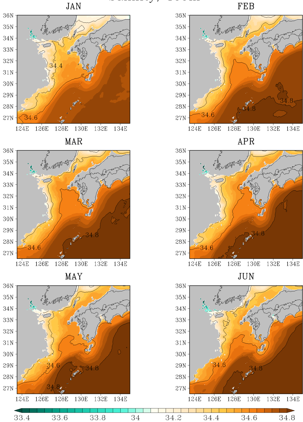
図 G - 13 100 m 深の塩分 (unitless)
