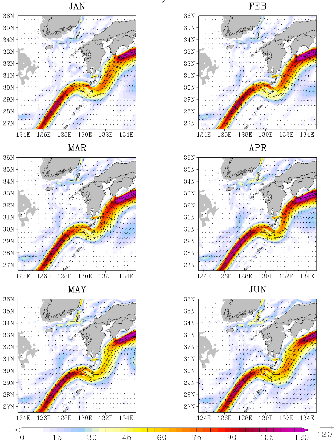
図G - 22 50 m 深の流速 ( cm/s )
