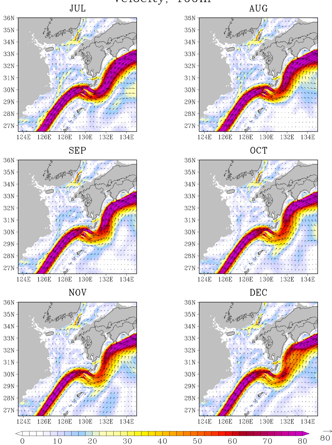
図 G - 23 (続く) 100 m 深の流速 ( cm/s )
