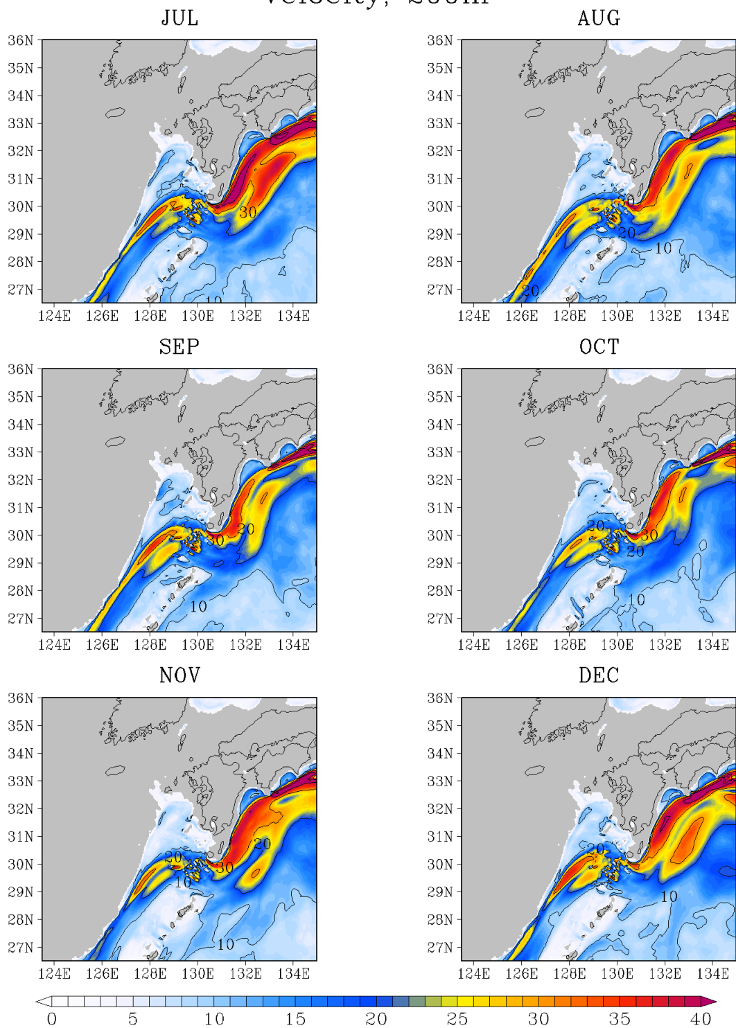
図G - 29 (続く) 200 m 深の流速 標準偏差 (cm/s)
