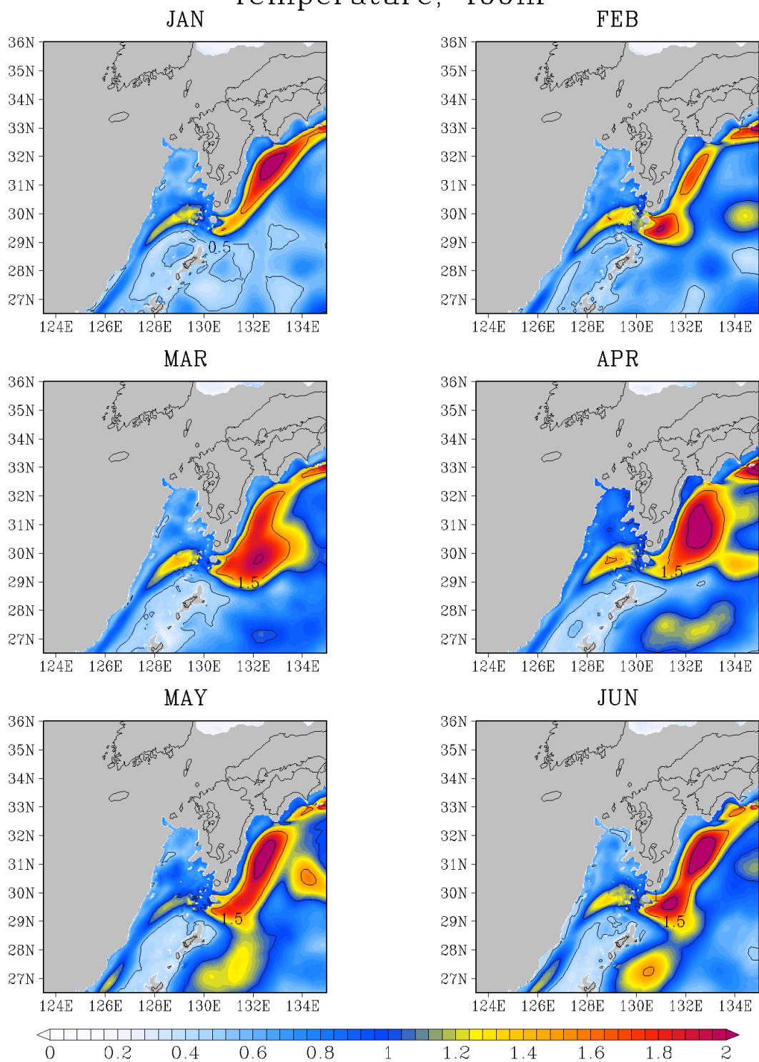
図G - 10 400 m 深の水温 標準偏差 (°C)
