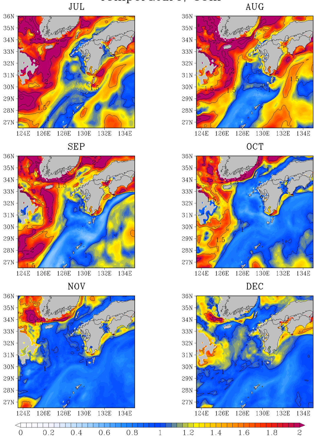
図G - 7 (続く) 50 m 深の水温 標準偏差 (°C)
