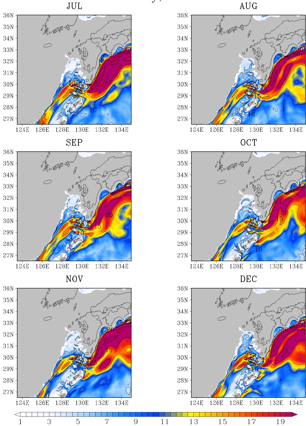
図G - 30 (続く) 400 m 深の流速 標準偏差 (cm/s)
