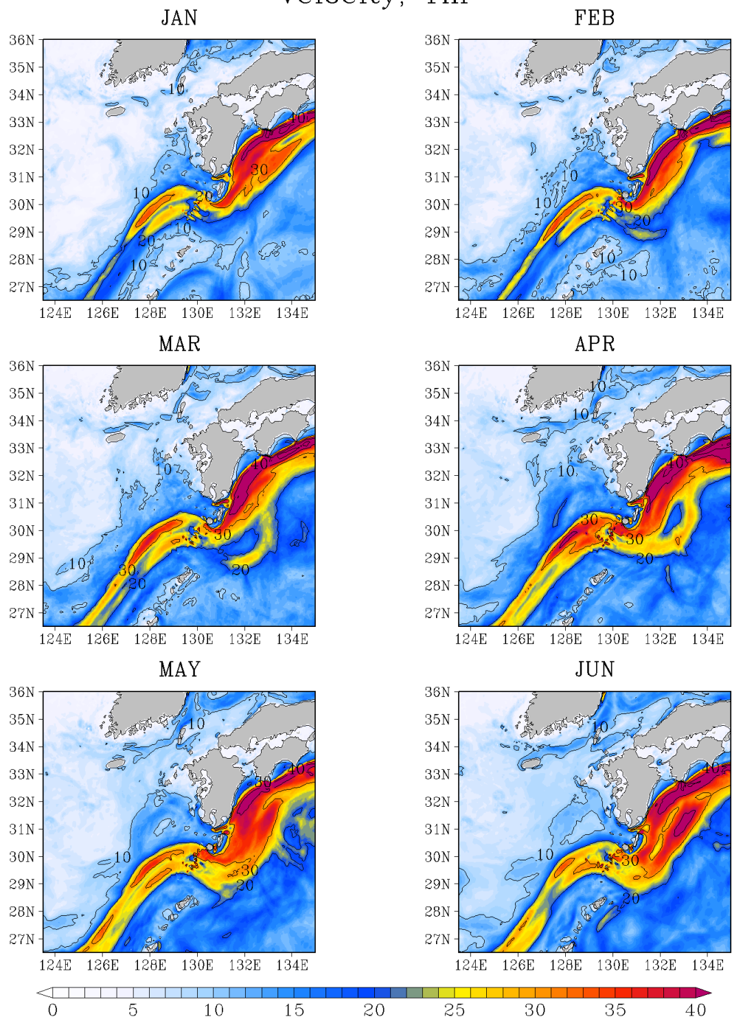
図G - 26 1 m 深の流速 標準偏差 (cm/s)
