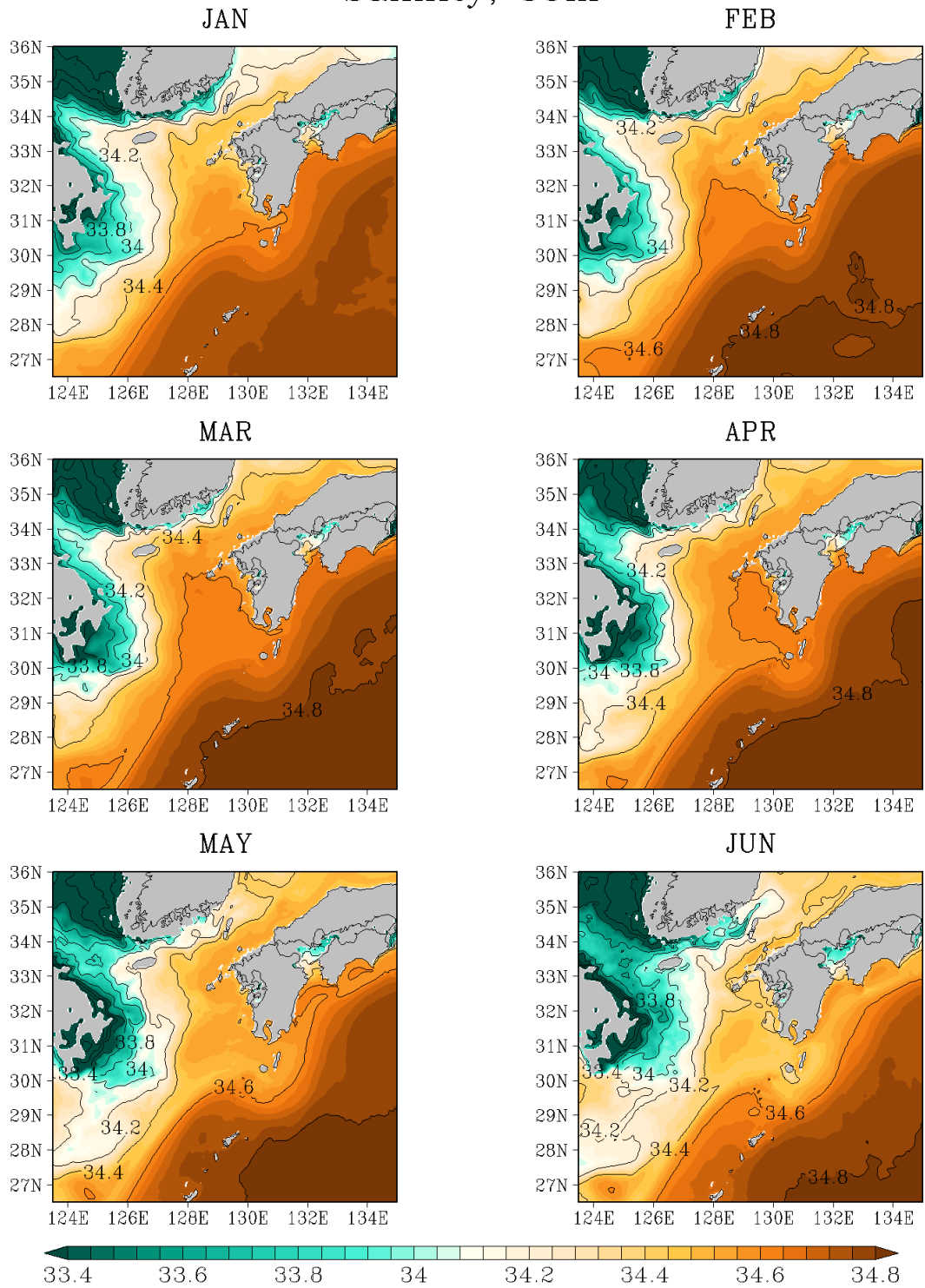
図G - 12 50 m 深の塩分 (unitless)
