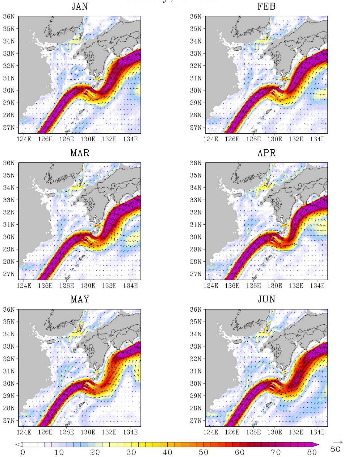
図 G - 23 100 m 深の流速 (cm/s)
