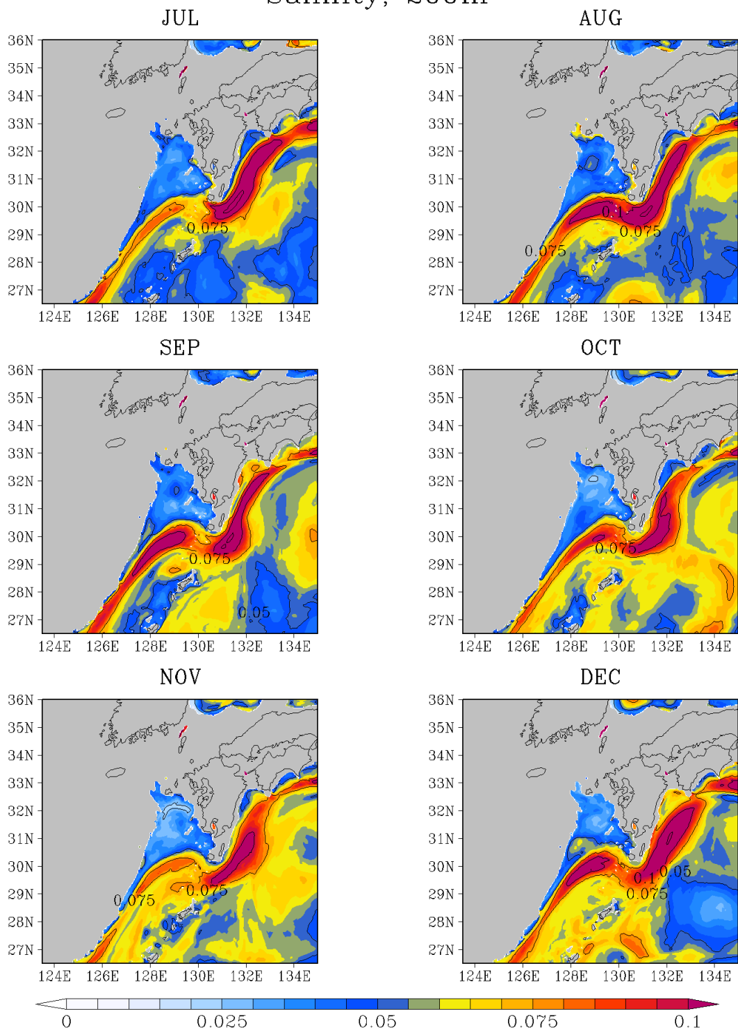
図G - 19 (続く) 200 m 深の塩分 標準偏差 (unitless)
