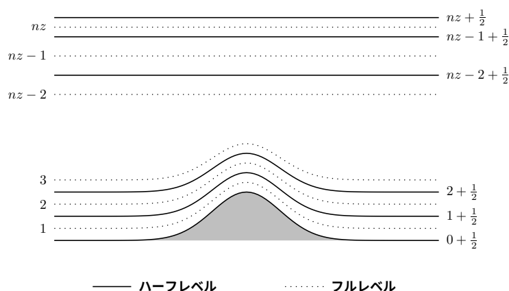
Figure D.1: エータ座標系の模式図 (GSM, RSM など)。地表面はハーフレベルの最下層に一致する。この地表面まで含めたときにハーフレベルの層数は鉛直層数 (フルレベルの層数) より 1 だけ多いことに注意。そのため、ハーフレベルに対応する値を格納する SUBC ETA の A , B の要素数が (鉛直層数+1) 必要になる。
