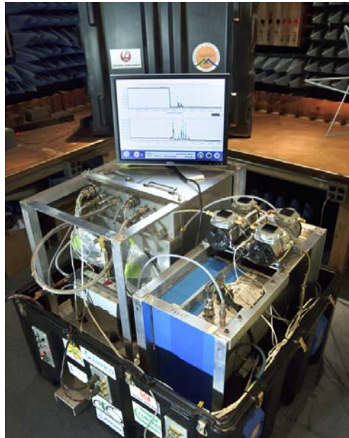
モジュール化して搭載される大気観測装置
