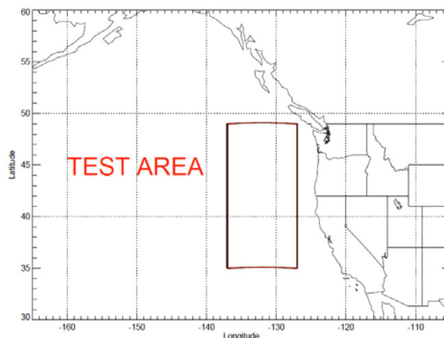
アメリカ西海岸における大気採取のテストエリア
