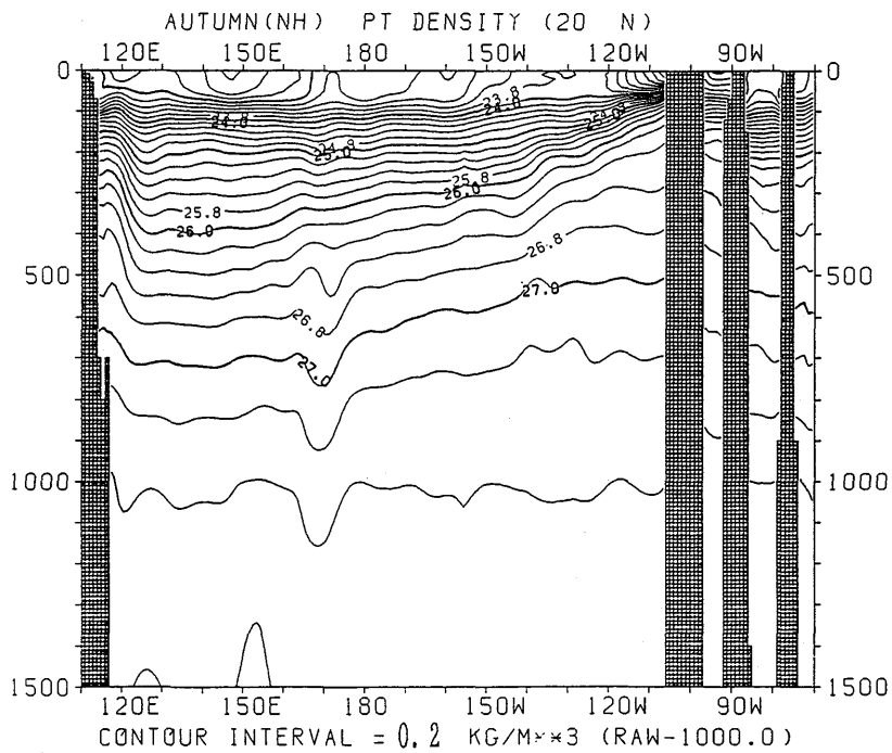
図 3.3.104 秋季におけるポテンシャル密度の東西断面分布 (20°N)
