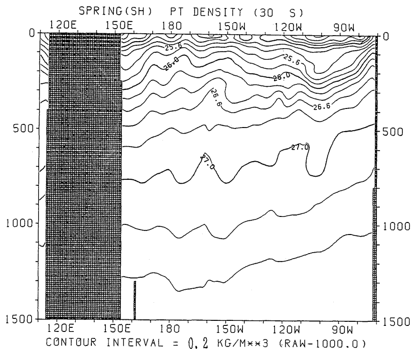
図 3.3.109 春季 (南半球) におけるポテンシャル密度の東西断面分布 (30°S)
