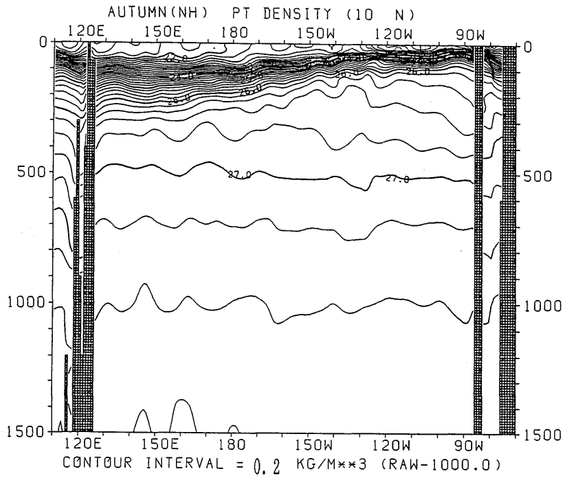
図 3.3.105 秋季におけるポテンシャル密度の東西断面分布 (10°N)
