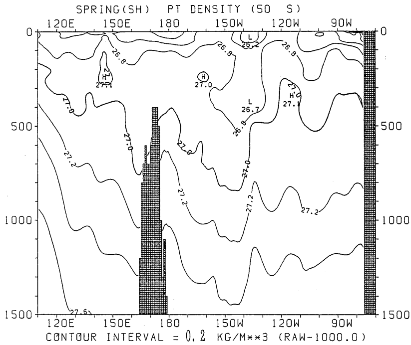
図 3.3.111 春季 (南半球) におけるポテンシャル密度の東西断面分布 (50°S)
