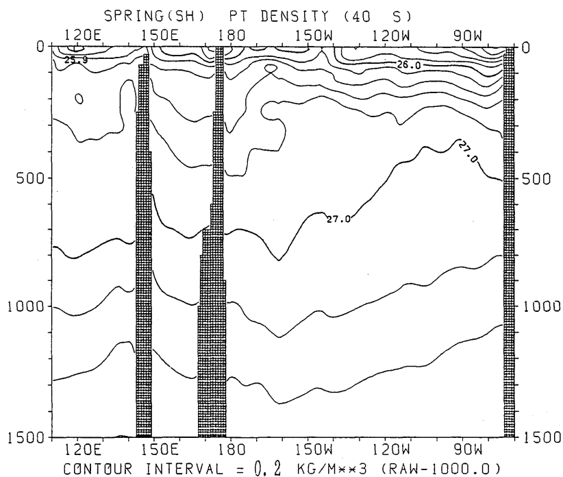
図 3.3.110 春季 (南半球) におけるポテンシャル密度の東西断面分布 (40°S)
