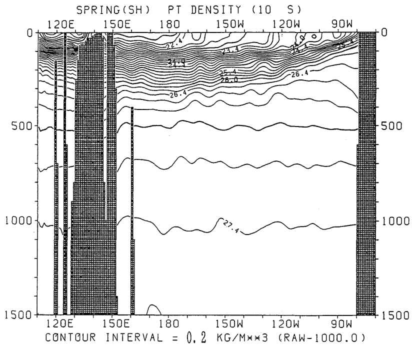
図 3.3.107 春季 (南半球) におけるポテンシャル密度の東西断面分布 (10°S)
