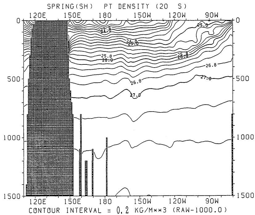
図 3.3.108 春季 (南半球) におけるポテンシャル密度の東西断面分布 (20°S)
