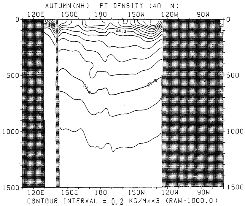
図 3.3.102 秋季におけるポテンシャル密度の東西断面分布 (40°N)
