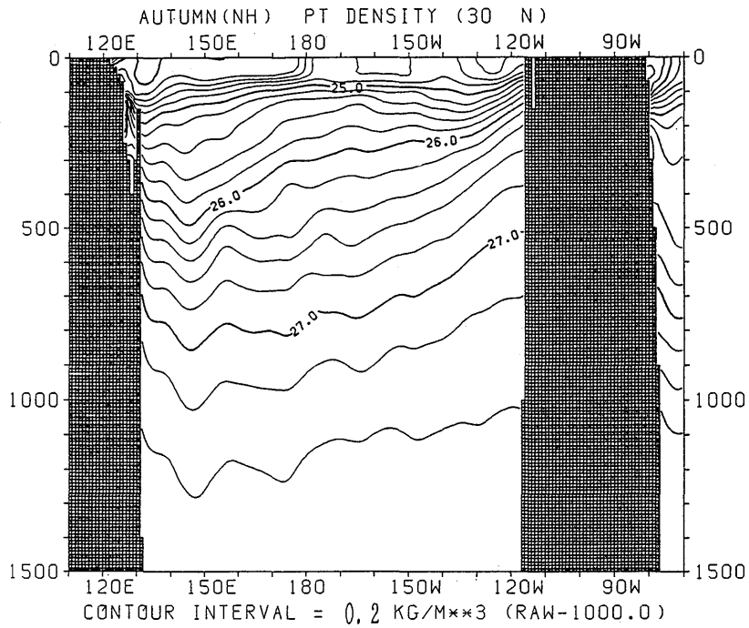
図 3.3.103 秋季におけるポテンシャル密度の東西断面分布 (30°N)
