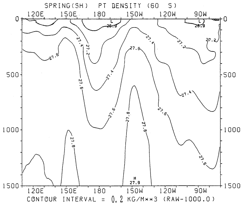
図 3.3.112 春季 (南半球) におけるポテンシャル密度の東西断面分布 (60°S)
