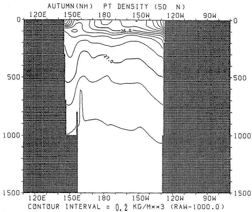
図 3.3.101 秋季におけるポテンシャル密度の東西断面分布 (50°N)
