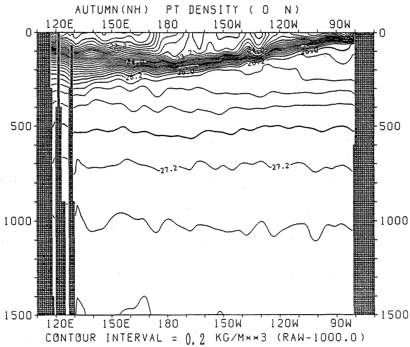
図 3.3.106 秋季におけるポテンシャル密度の東西断面分布 (赤道)
