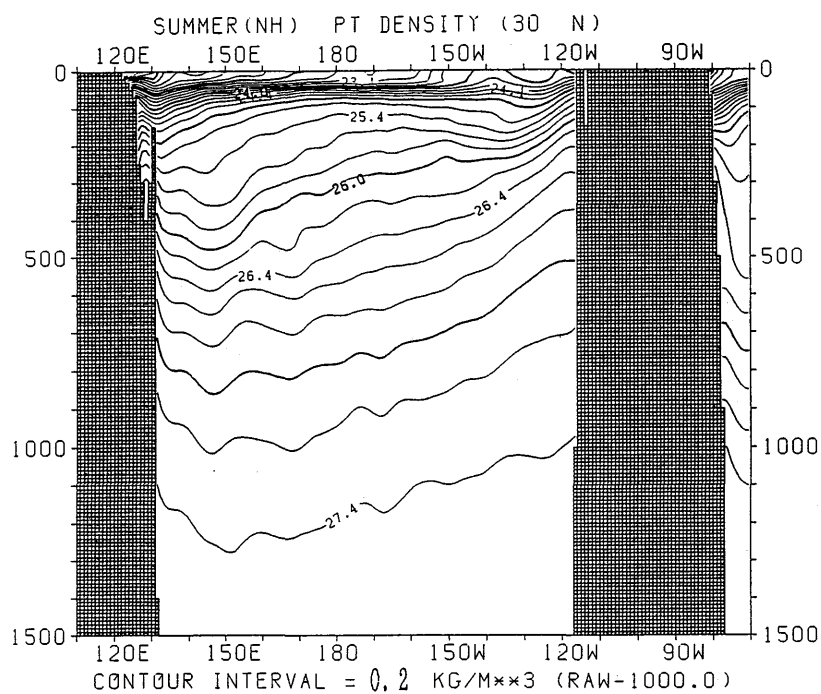
図 3.3.91 夏季におけるポテンシャル密度の東西断面分布 (30°N)
