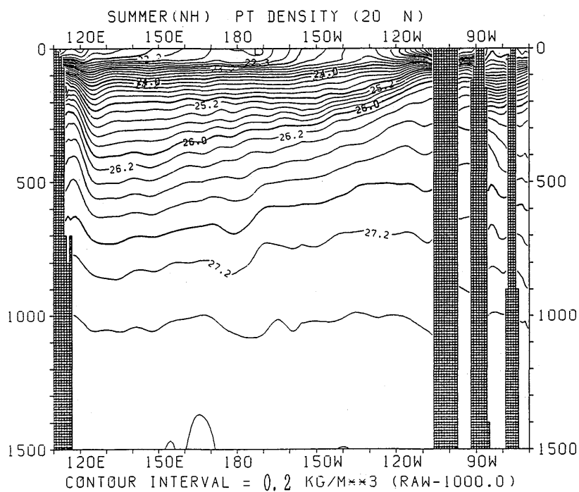
図 3.3.92 夏季におけるポテンシャル密度の東西断面分布 (20°N)
