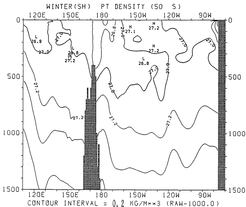
図 3.3.99 冬季 (南半球) におけるポテンシャル密度の東西断面分布 (50°S)
