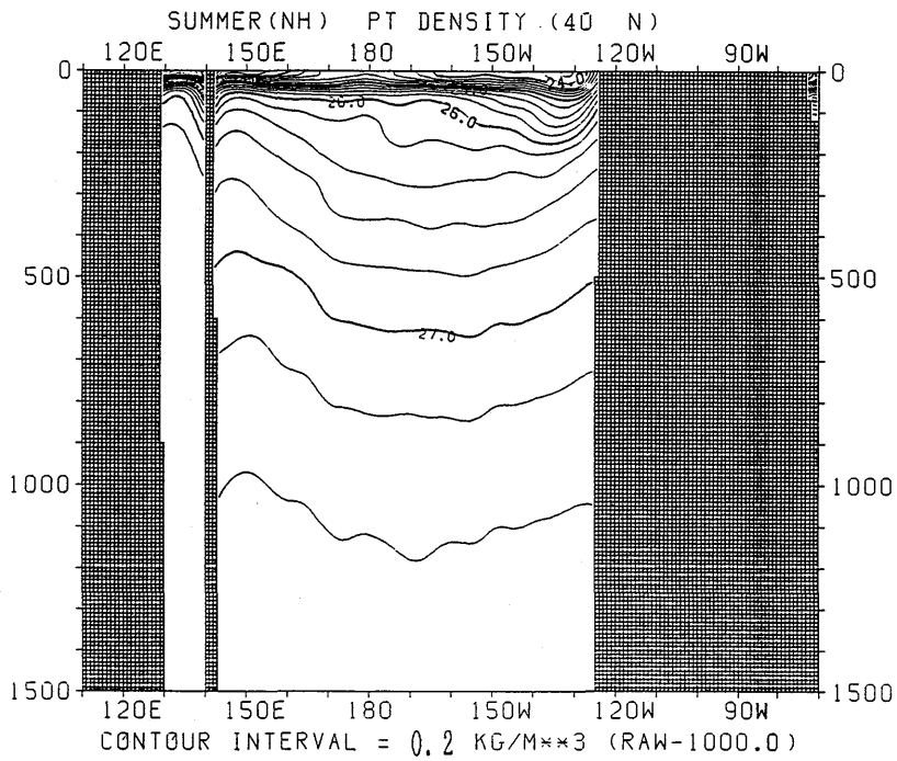
図 3.3.90 夏季におけるポテンシャル密度の東西断面分布 (40°N)
