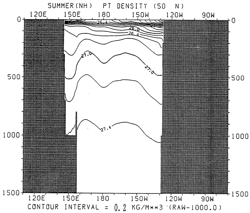
図 3.3.89 夏季におけるポテンシャル密度の東西断面分布 (50°N)
