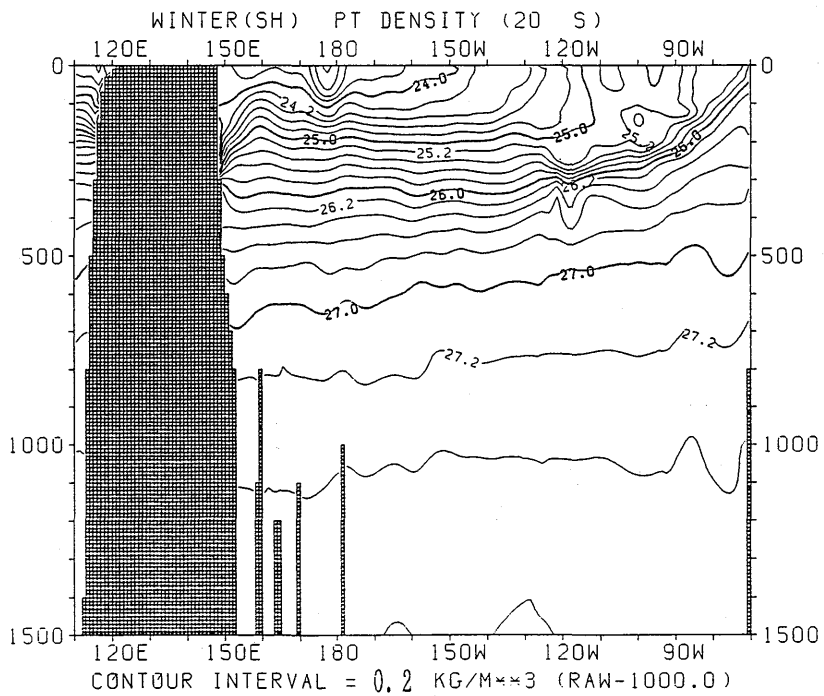
図 3.3.96 冬季 (南半球) におけるポテンシャル密度の東西断面分布 (20°S)
