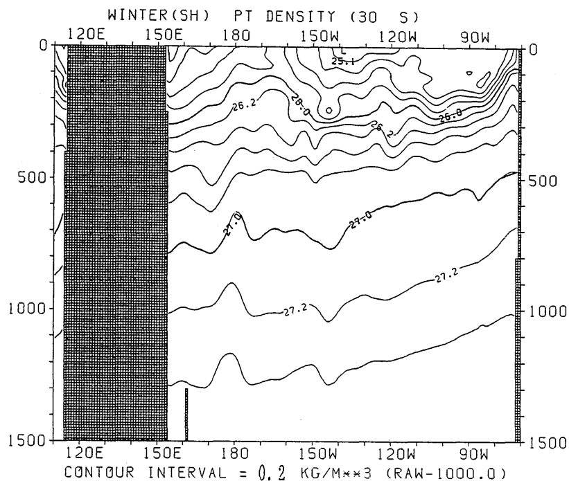
図 3.3.97 冬季 (南半球) におけるポテンシャル密度の東西断面分布 (30°S)
