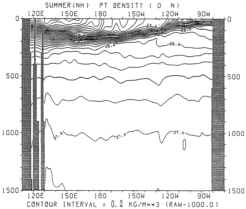
図 3.3.94 夏季におけるポテンシャル密度の東西断面分布 (赤道)
