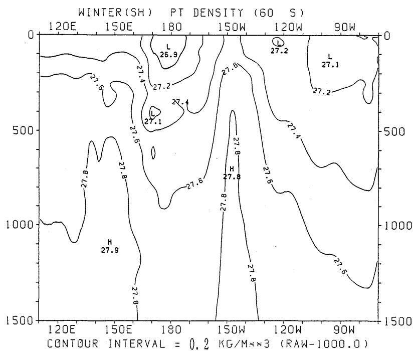
図 3.3.100 冬季 (南半球) におけるポテンシャル密度の東西断面分布 (60°S)
