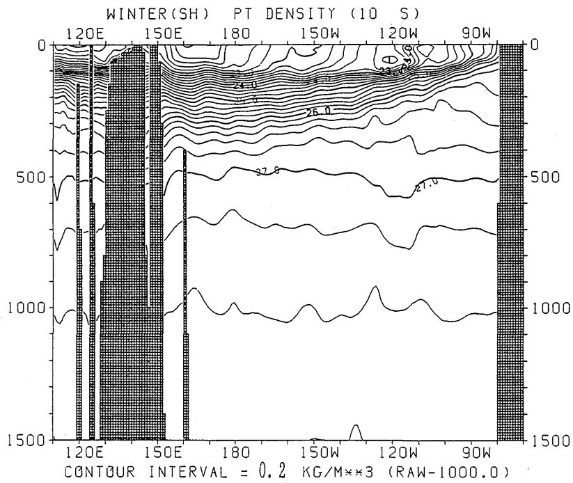
図 3.3.95 冬季 (南半球) におけるポテンシャル密度の東西断面分布 (10°S)
