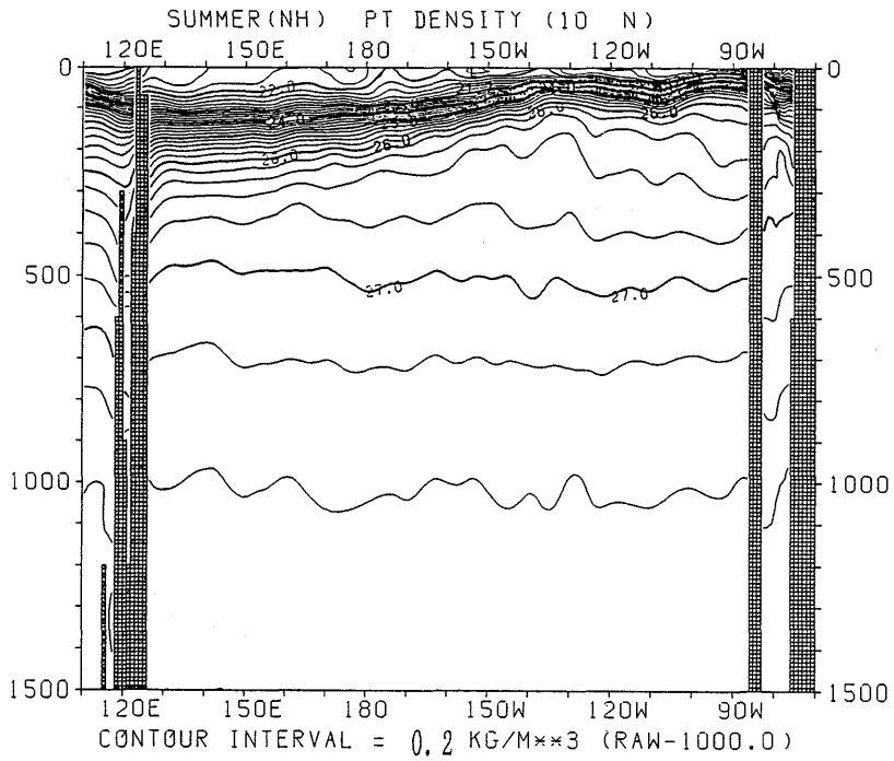
図 3.3.93 夏季におけるポテンシャル密度の東西断面分布 (10°N)
