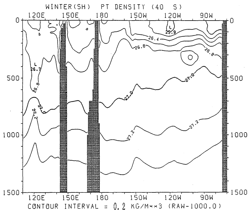
図 3.3.98 冬季 (南半球) におけるポテンシャル密度の東西断面分布 (40°S)
