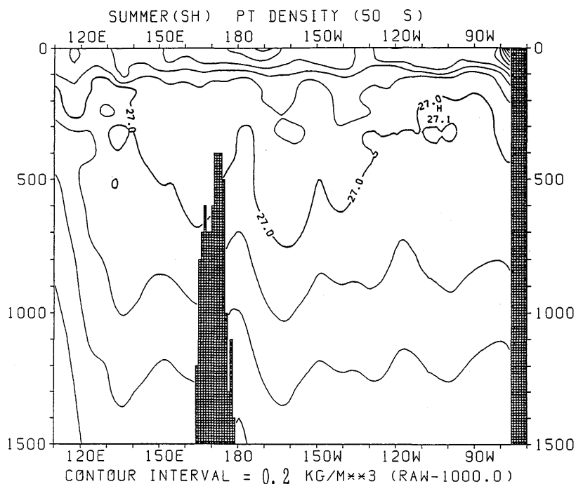
図 3.3.75 夏季 (南半球) におけるポテンシャル密度の東西断面分布 (50°S)
