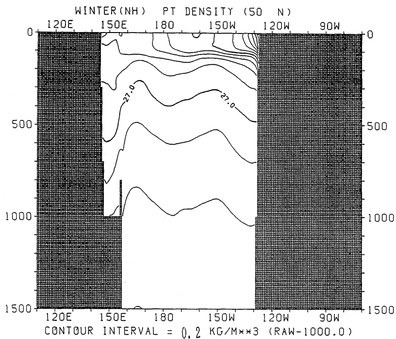
図 3.3.65 冬季におけるポテンシャル密度の東西断面分布 (50°N)
