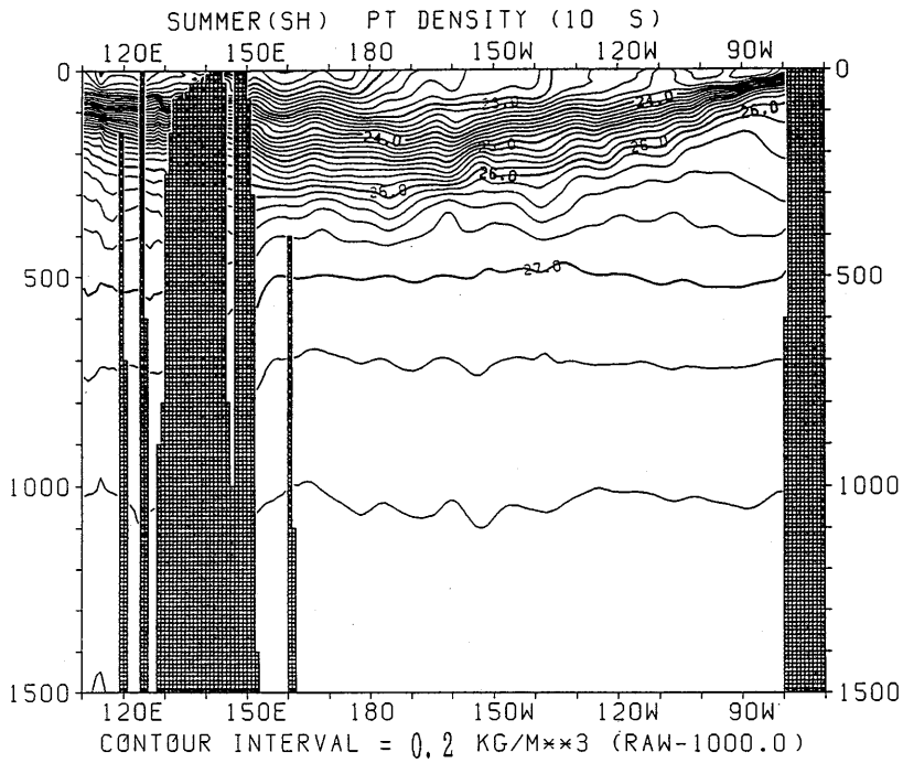
図 3.3.71 夏季（南半球）におけるポテンシャル密度の東西断面分布（10°S）
