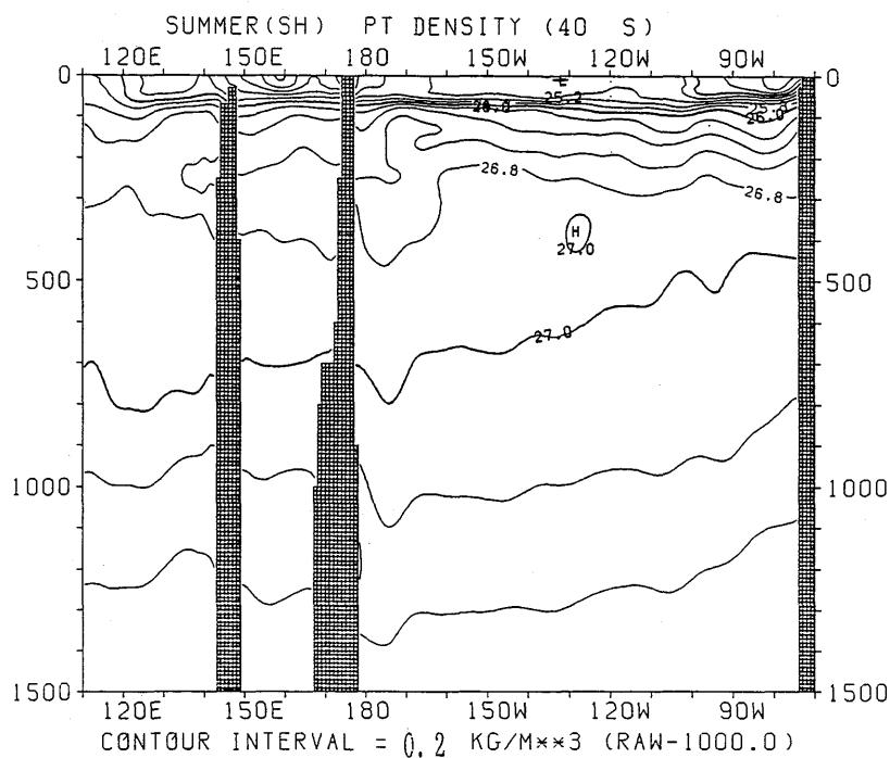
図 3.3.74 夏季 (南半球) におけるポテンシャル密度の東西断面分布 (40°S)
