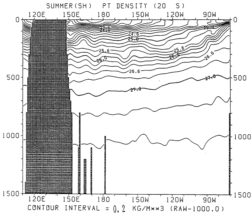
図 3.3.72 夏季（南半球）におけるポテンシャル密度の東西断面分布（20°S）
