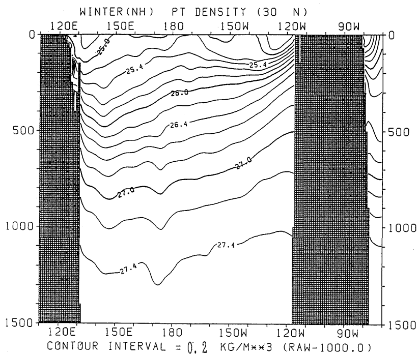
図 3.3.67 冬季におけるポテンシャル密度の東西断面分布 (30°N)
