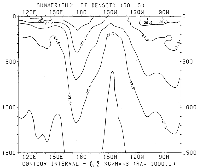
図 3.3.76 夏季 (南半球) におけるポテンシャル密度の東西断面分布 (60°S)
