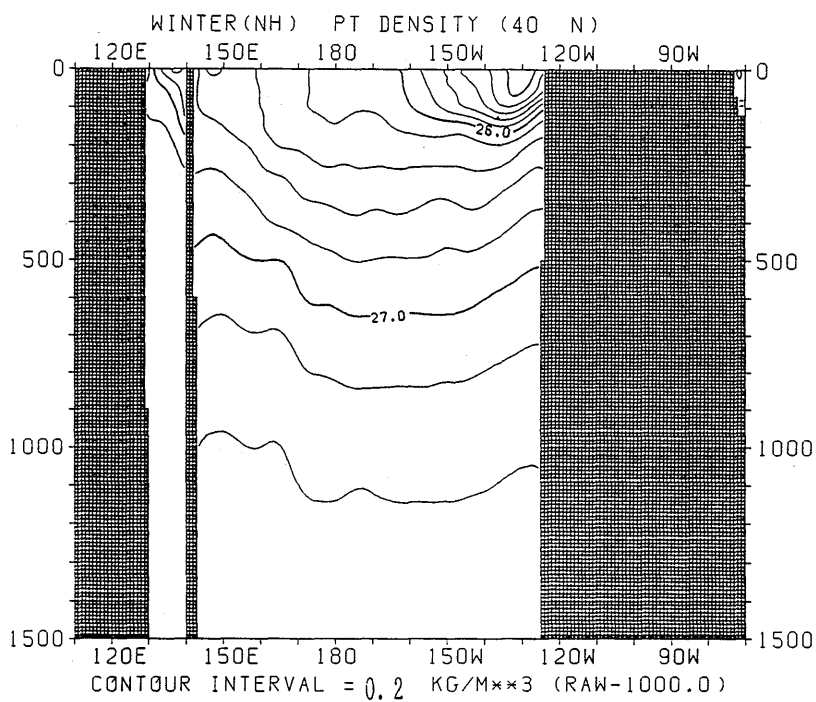
図 3.3.66 冬季におけるポテンシャル密度の東西断面分布 (40°N)
