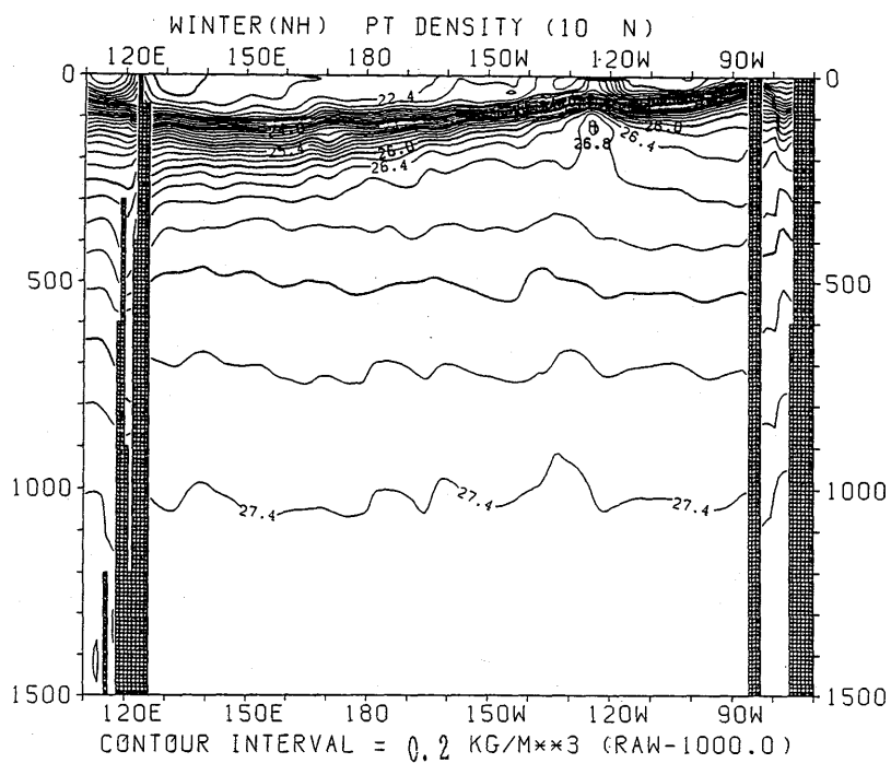
図 3.3.69 冬季におけるポテンシャル密度の東西断面分布 (10°N)
