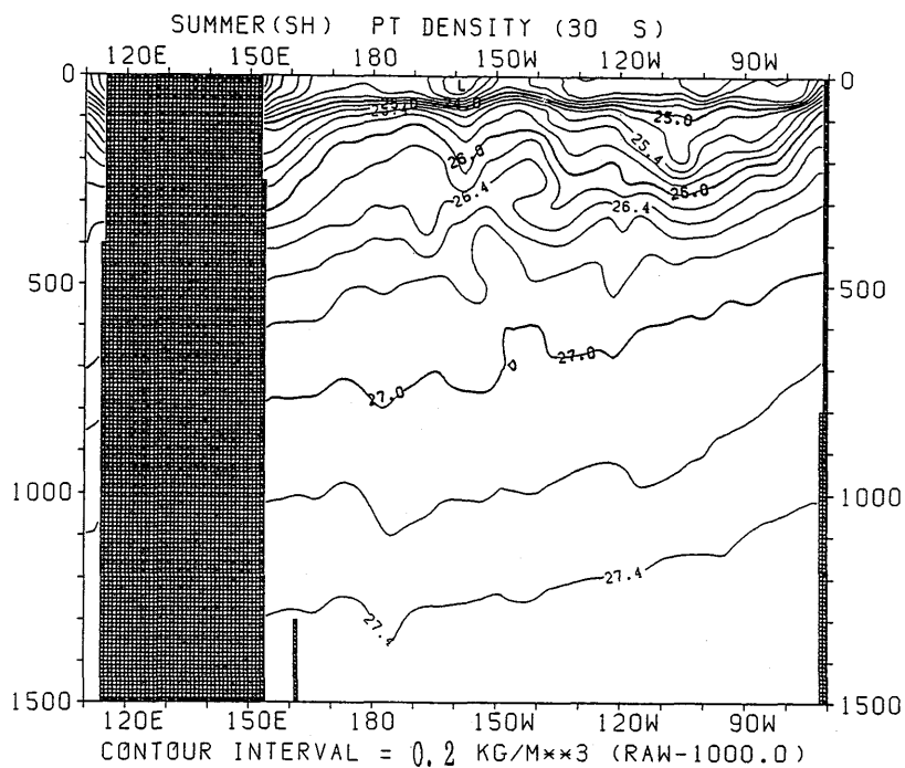
図 3.3.73 夏季 (南半球) におけるポテンシャル密度の東西断面分布 (30°S)
