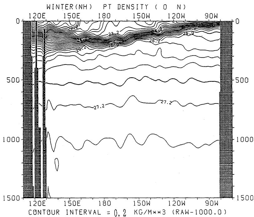
図 3.3.70 冬季におけるポテンシャル密度の東西断面分布 (赤道)
