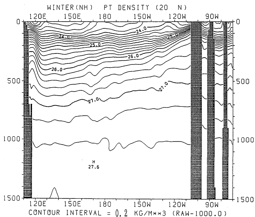
図 3.3.68 冬季におけるポテンシャル密度の東西断面分布 (20°N)
