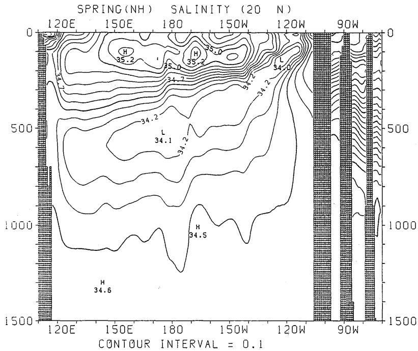
図 3.2.80 春季における塩分の東西断面分布 (20°N)
