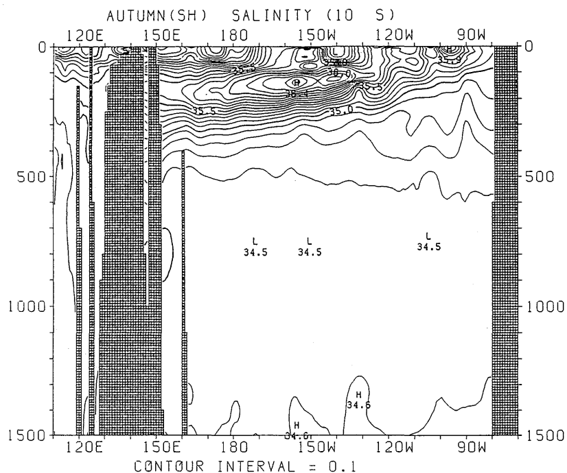
図 3.2.83 秋季（南半球）における塩分の東西断面分布（10°S）
