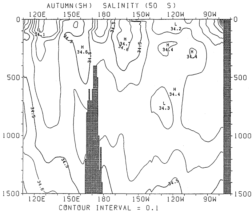
図 3.2.87 秋季 (南半球) における塩分の東西断面分布 (50°S)
