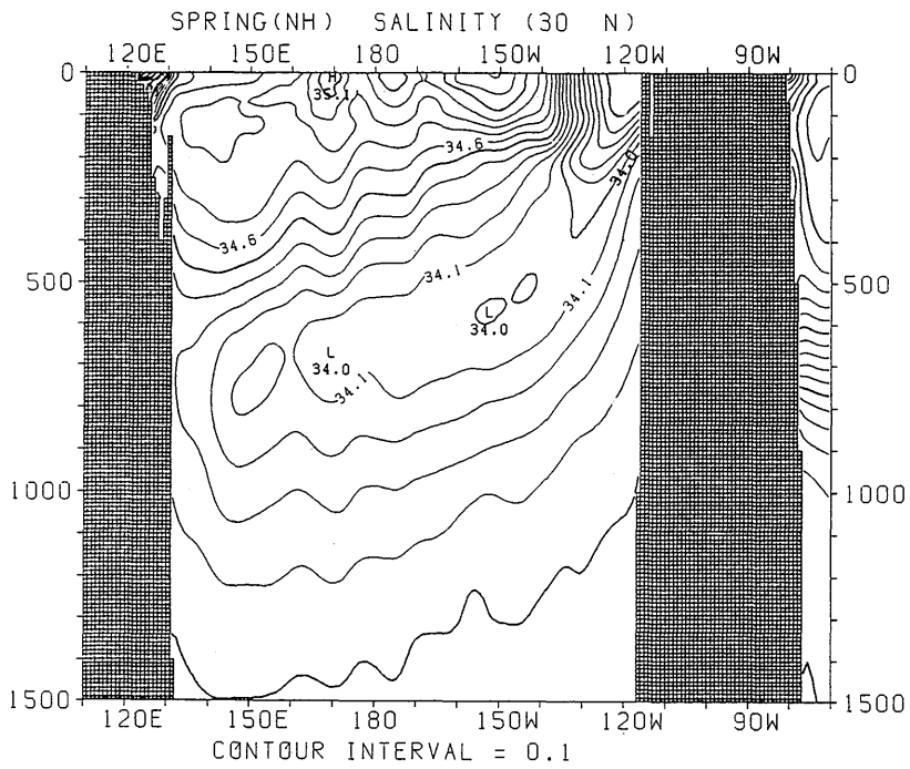
図 3.2.79 春季における塩分の東西断面分布 (30°N)
