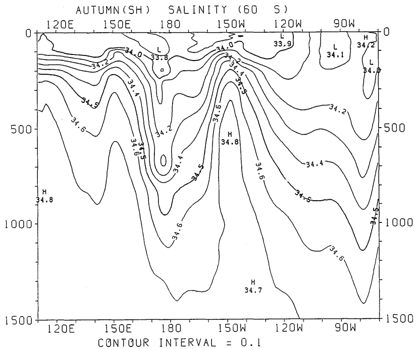
図 3.2.88 秋季 (南半球) における塩分の東西断面分布 (60°S)
