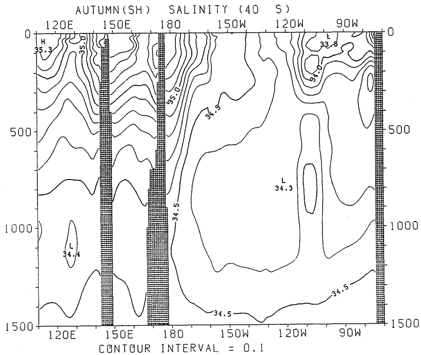
図 3.2.86 秋季 (南半球) における塩分の東西断面分布 (40°S)
