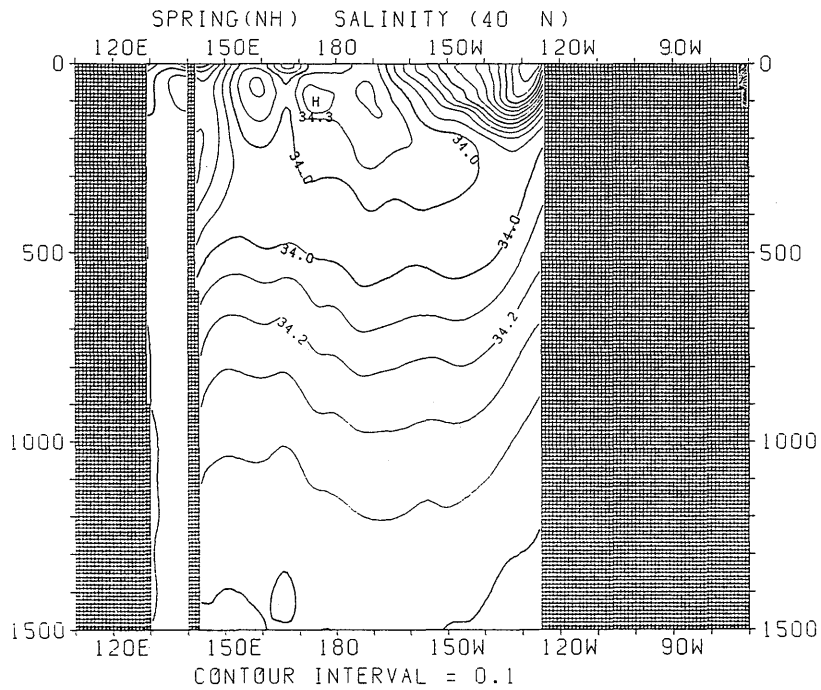
図 3.2.78 春季における塩分の東西断面分布 (40°N)
