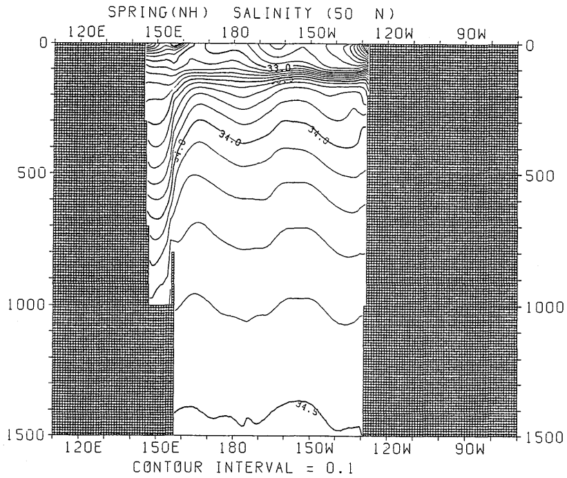
図 3.2.77 春季における塩分の東西断面分布 (50°N)
