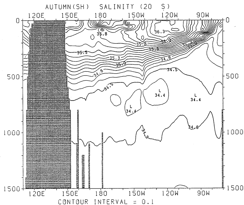
図 3.2.84 秋季（南半球）における塩分の東西断面分布（20°S）
