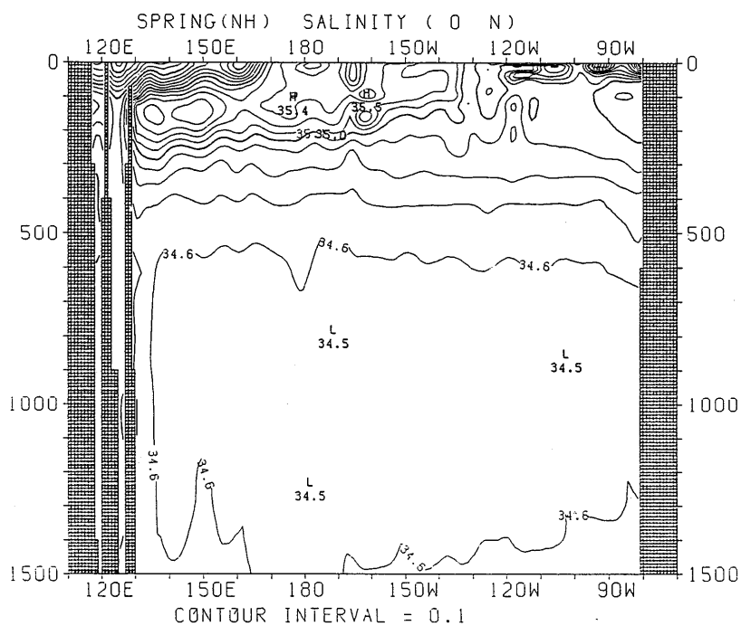
図 3.2.82 春季における塩分の東西断面分布 (赤道)
