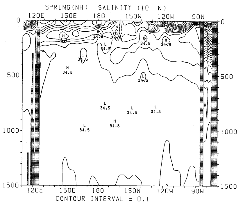
図 3.2.81 春季における塩分の東西断面分布 (10°N)
