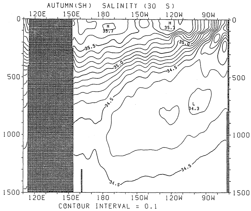
図 3.2.85 秋季 (南半球) における塩分の東西断面分布 (30°S)
