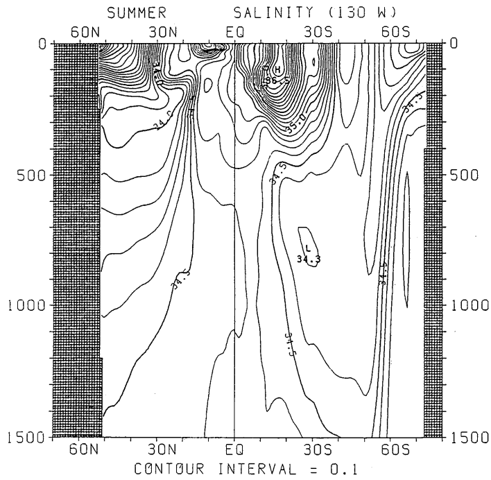
図 3.2.43 夏季における塩分の南北断面分布 (130°W)
