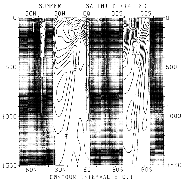
図 3.2.34 夏季における塩分の南北断面分布 (140°E)
