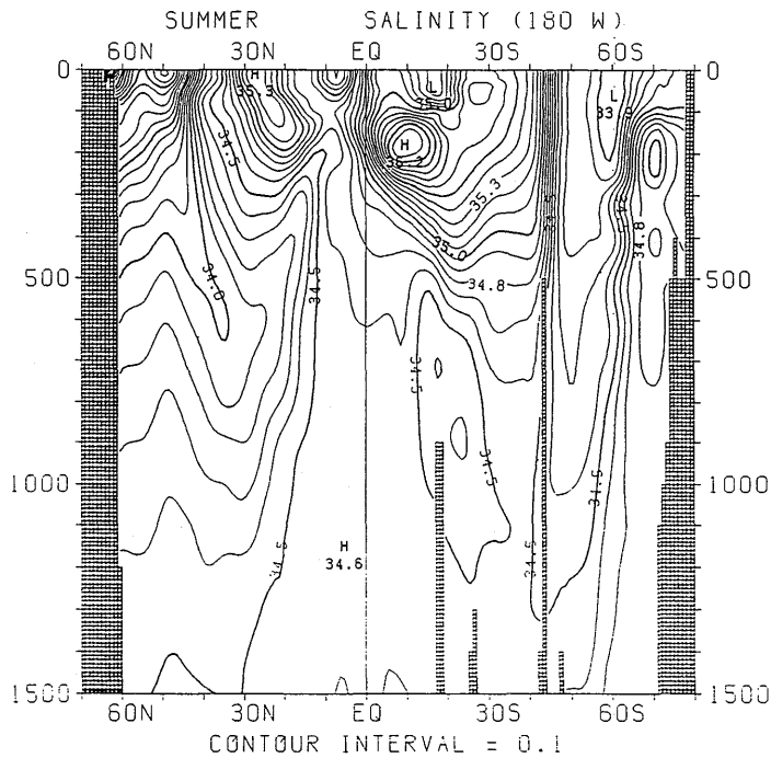
図 3.2.38 夏季における塩分の南北断面分布 (180°)
