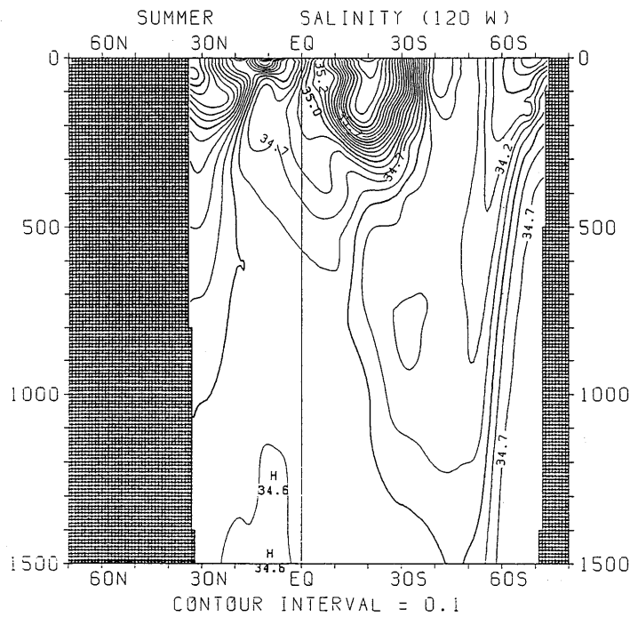
図 3.2.44 夏季における塩分の南北断面分布 (120°W)
