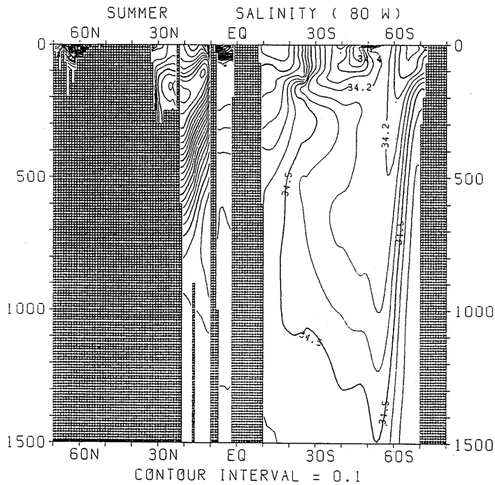
図 3.2.48 夏季における塩分の南北断面分布 (80°W)
