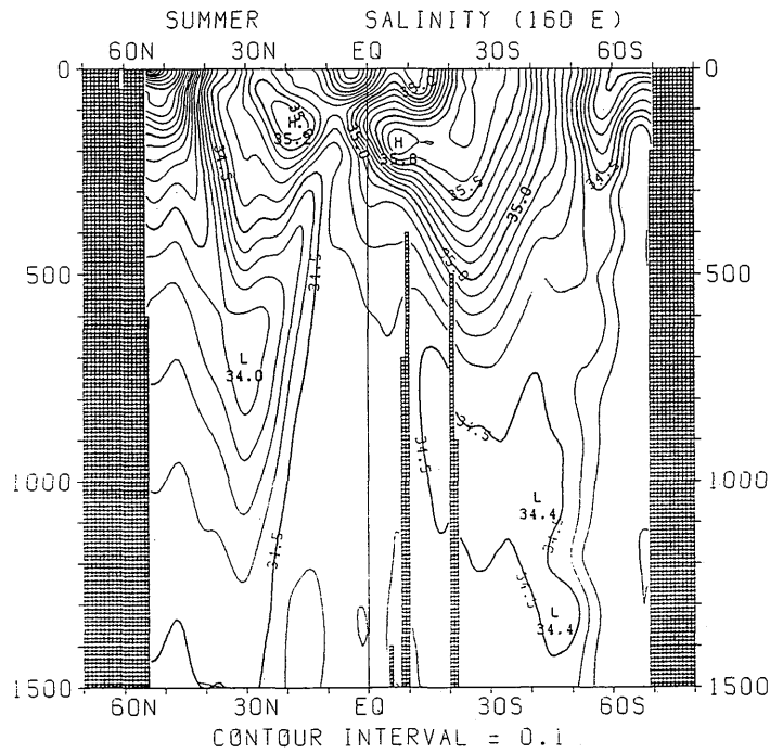
図 3.2.36 夏季における塩分の南北断面分布 (160°E)
