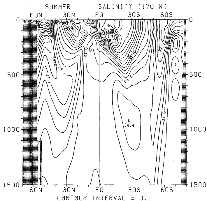
図 3.2.39 夏季における塩分の南北断面分布 (170°W)
