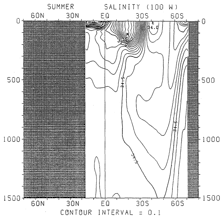
図 3.2.46 夏季における塩分の南北断面分布 (100°W)
