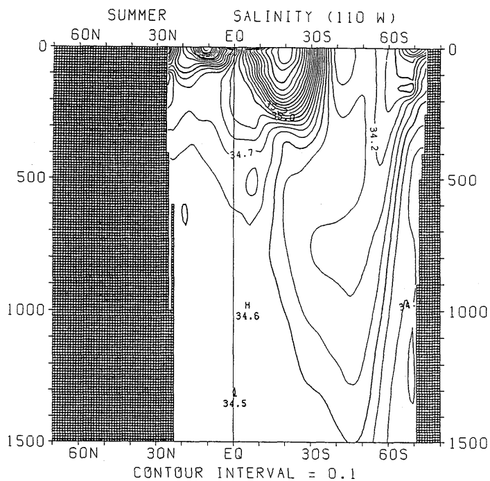
図 3.2.45 夏季における塩分の南北断面分布 (110°W)
