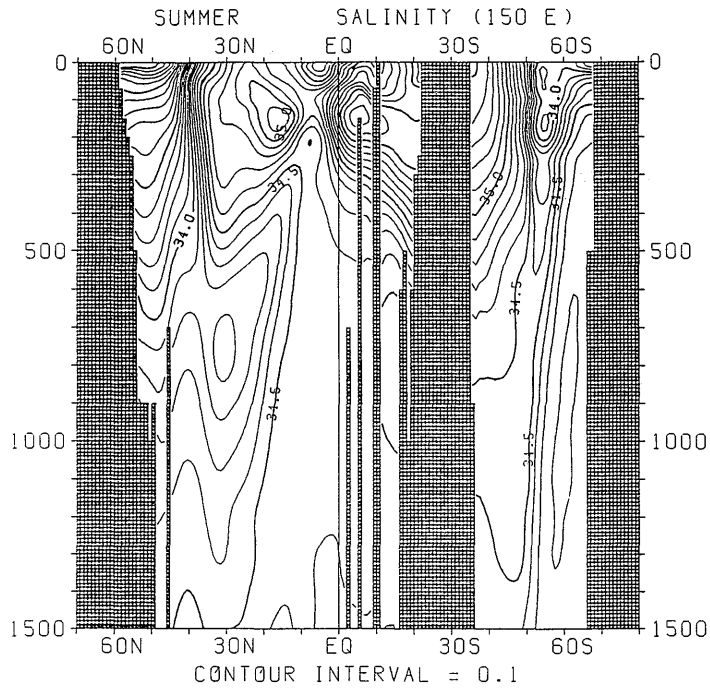
図 3.2.35 夏季における塩分の南北断面分布 (150°E)
