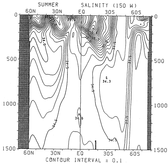
図 3.2.41 夏季における塩分の南北断面分布 (150°W)
