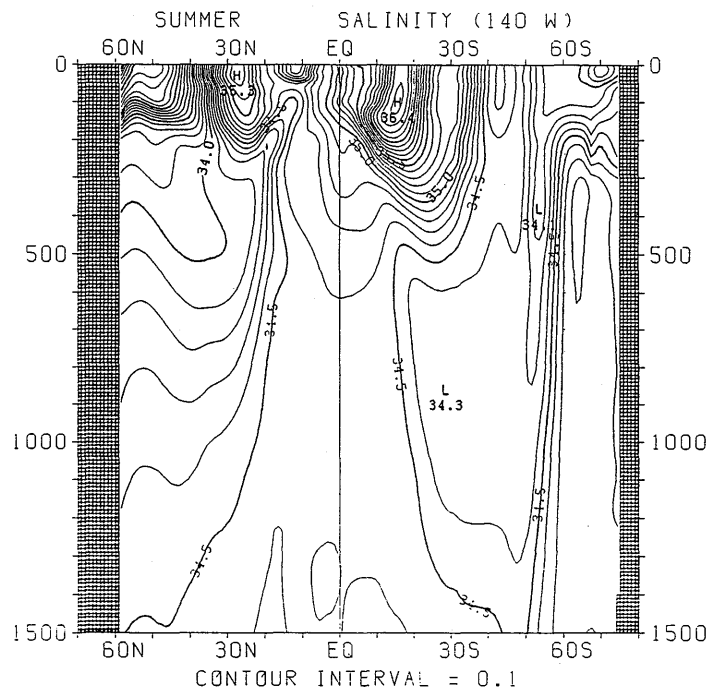
図 3.2.42 夏季における塩分の南北断面分布 (140°W)
