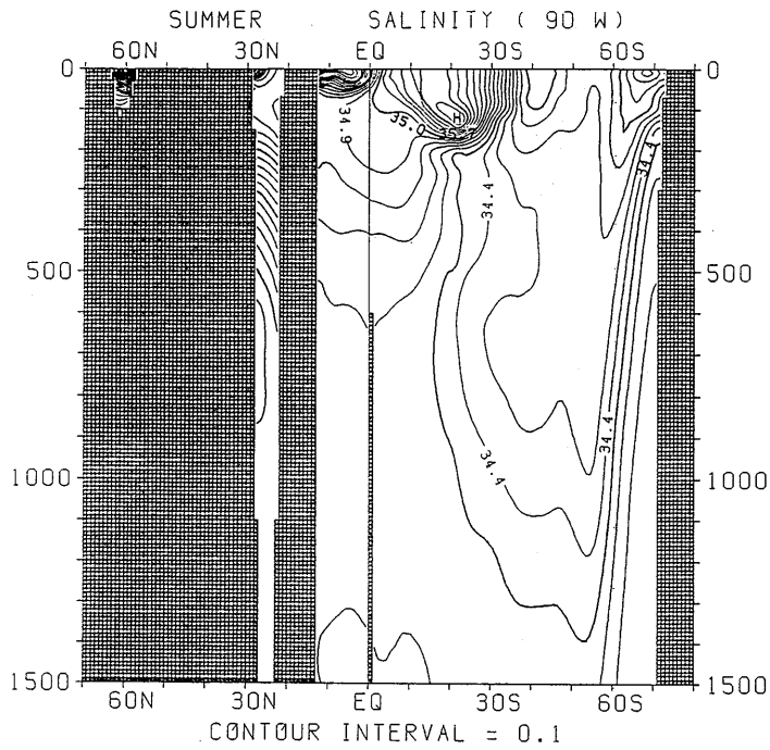
図 3.2.47 夏季における塩分の南北断面分布 (90°W)
