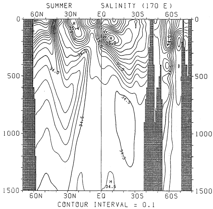
図 3.2.37 夏季における塩分の南北断面分布 (170°E)
