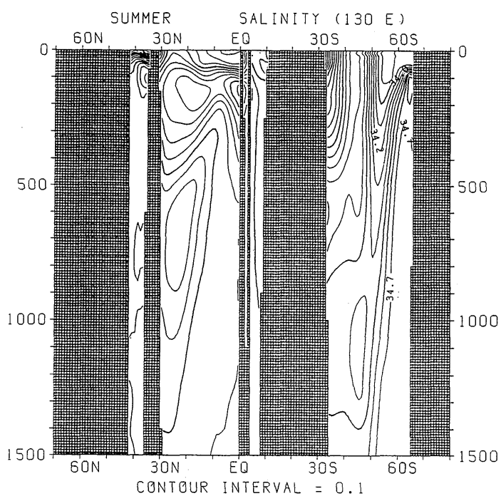
図 3.2.33 夏季における塩分の南北断面分布 (130°E)
