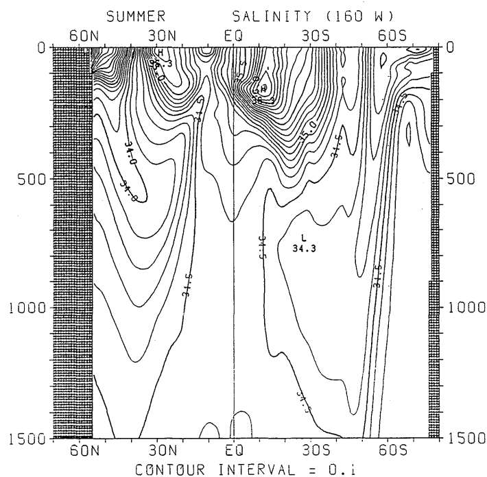
図 3.2.40 夏季における塩分の南北断面分布 (160°W)
