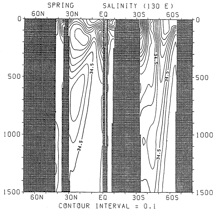
図 3.2.17 春季における塩分の南北断面分布 (130°E)
