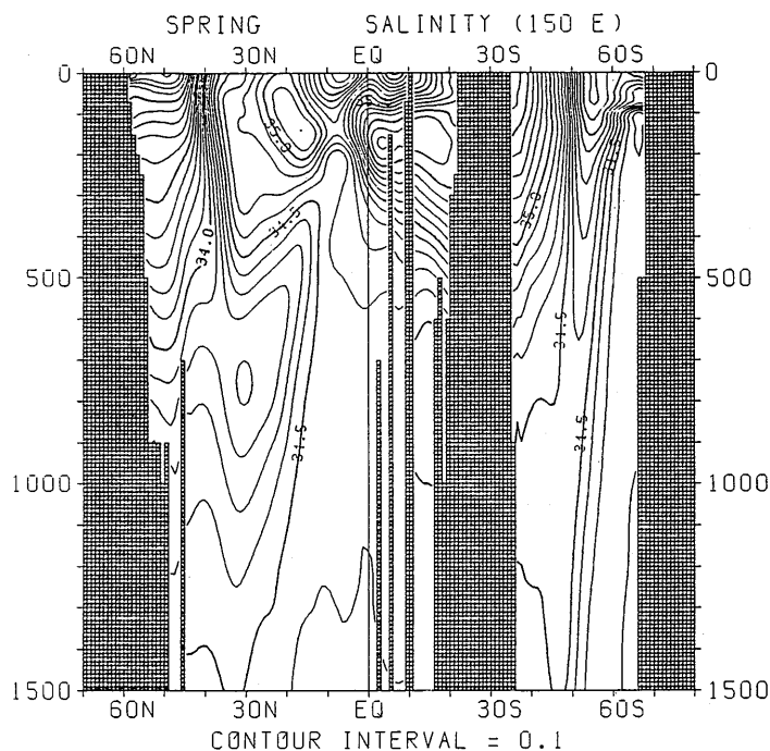
図 3.2.19 春季における塩分の南北断面分布 (150°E)
