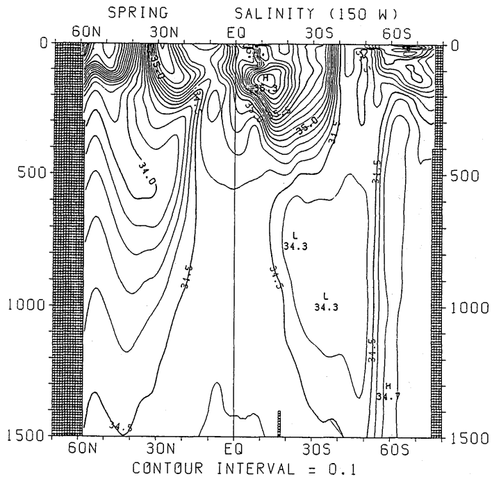
図 3.2.25 春季における塩分の南北断面分布 (150°W)
