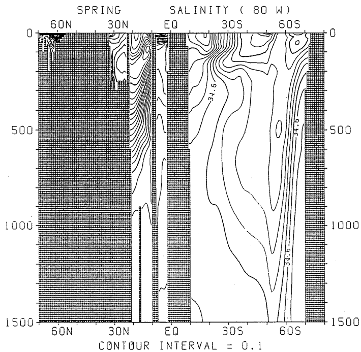
図 3.2.32 春季における塩分の南北断面分布 (80°W)
