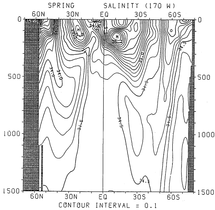
図 3.2.23 春季における塩分の南北断面分布 (170°W)
