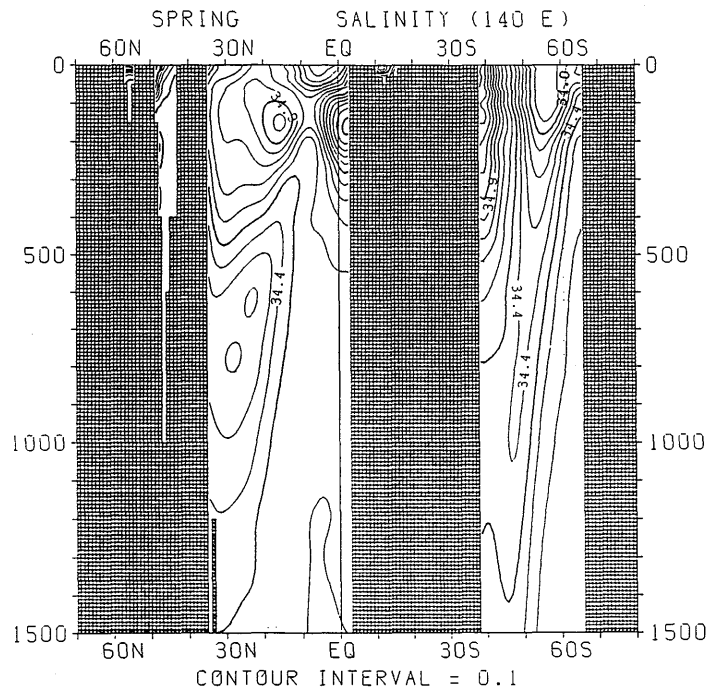
図 3.2.18 春季における塩分の南北断面分布 (140°E)
