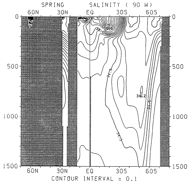
図 3.2.31 春季における塩分の南北断面分布 (90°W)
