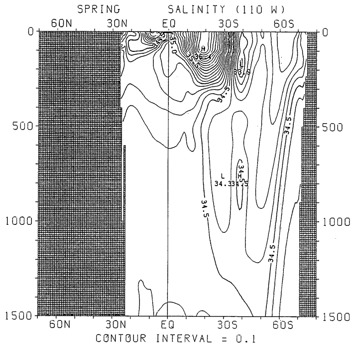
図 3.2.29 春季における塩分の南北断面分布 (110°W)
