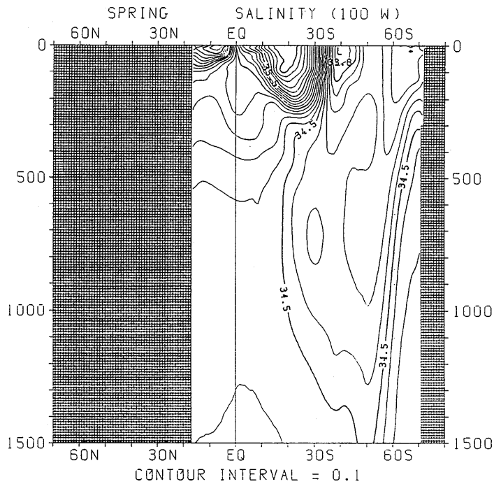
図 3.2.30 春季における塩分の南北断面分布 (100°W)
