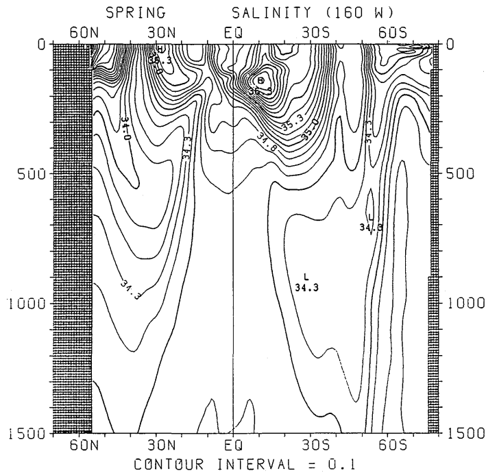
図 3.2.24 春季における塩分の南北断面分布 (160°W)
