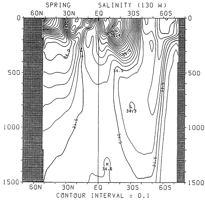
図 3.2.27 春季における塩分の南北断面分布 (130°W)
