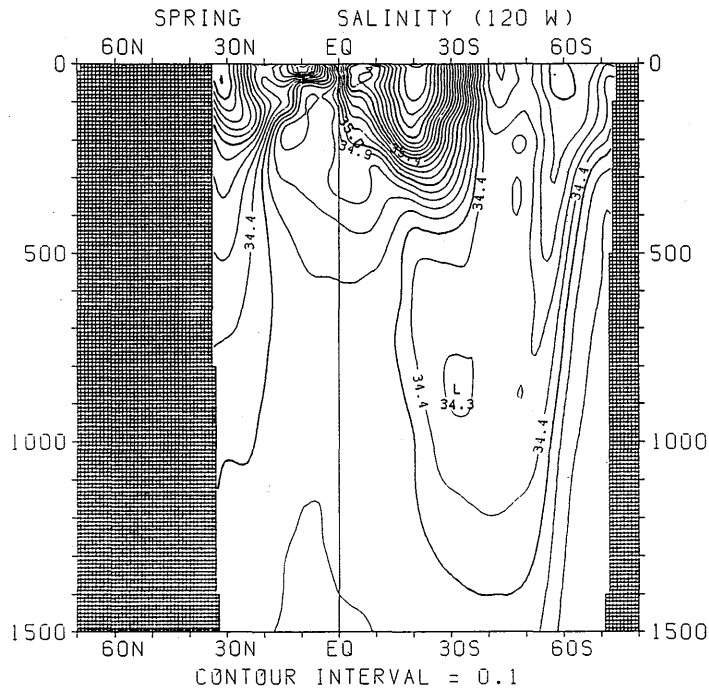
図 3.2.28 春季における塩分の南北断面分布 (120°W)
