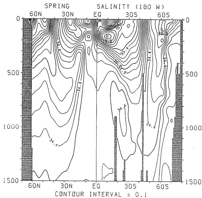
図 3.2.22 春季における塩分の南北断面分布 (180°)
