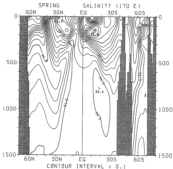
図 3.2.21 春季における塩分の南北断面分布 (170°E)
