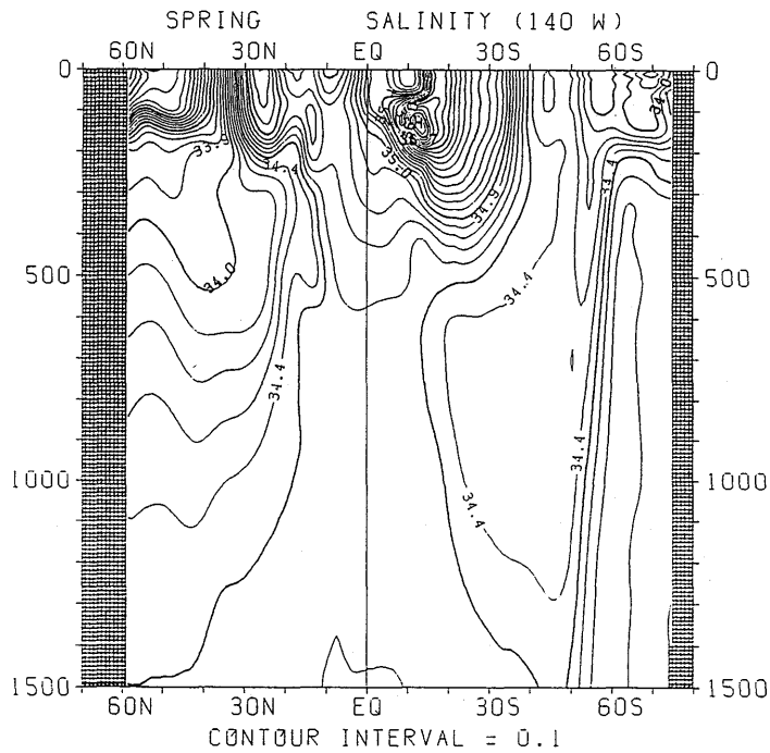
図 3.2.26 春季における塩分の南北断面分布 (140°W)
