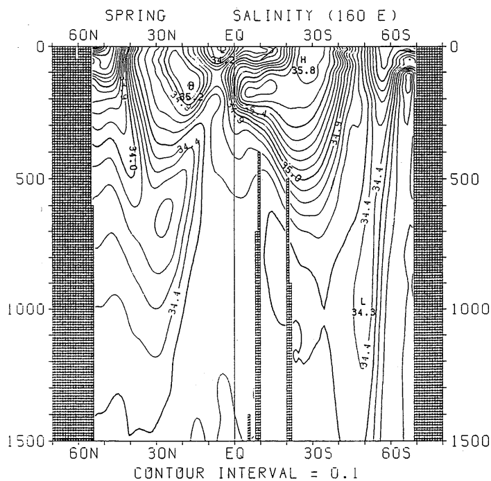
図 3.2.20 春季における塩分の南北断面分布 (160°E)
