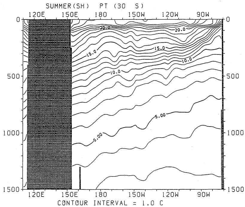
図 3.1.73 夏季 (南半球) におけるポテンシャル水温の東西断面分布 (30°S)
