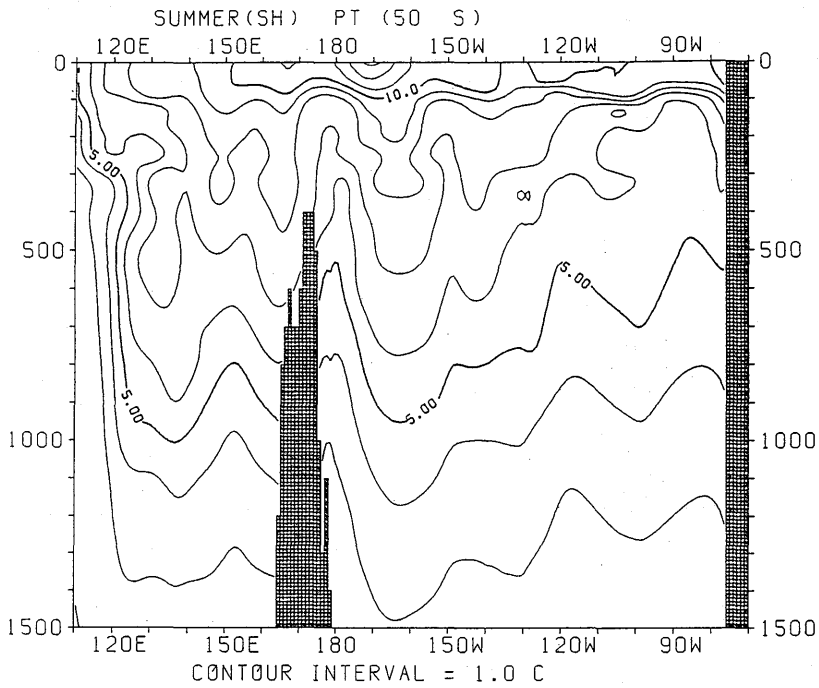
図 3.1.75 夏季(南半球)におけるポテンシャル水温の東西断面分布 (50°S)
