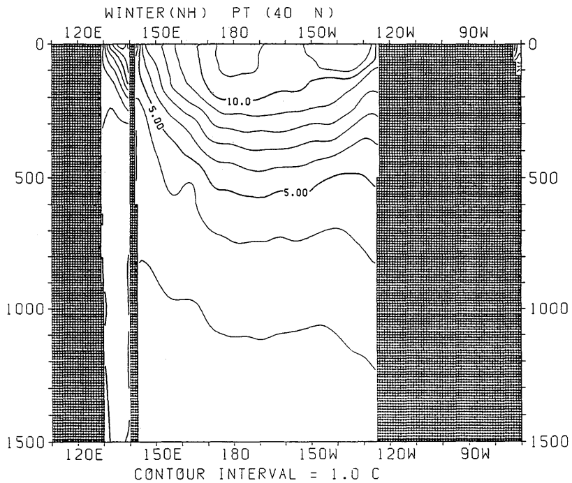
図 3.1.66 冬季におけるポテンシャル水温の東西断面分布 (40°N)
