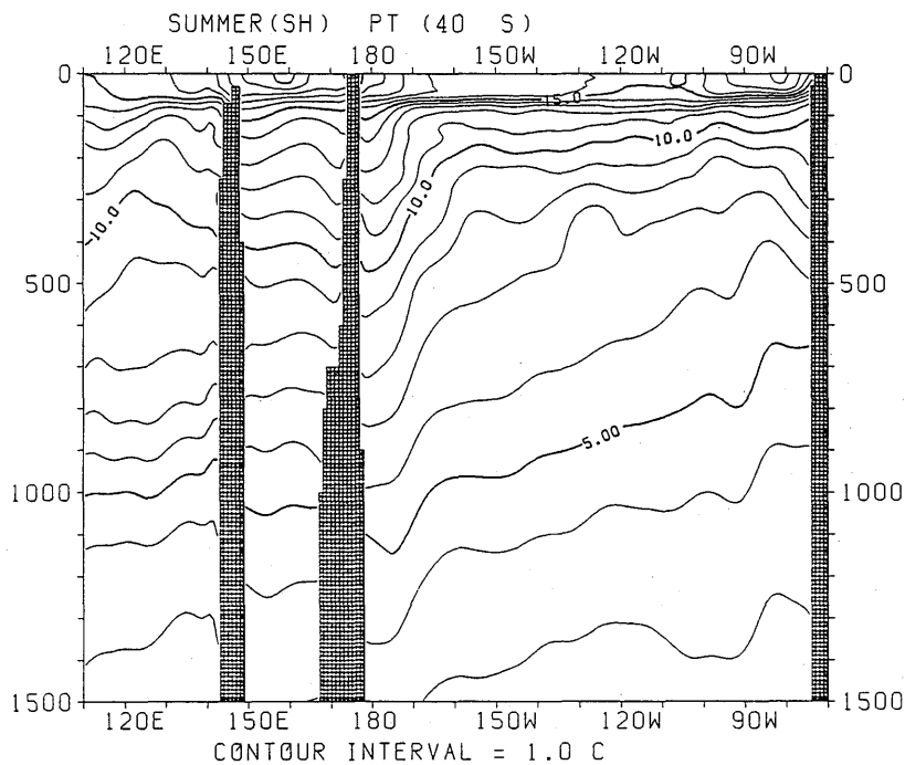
図 3.1.74 夏季 (南半球) におけるポテンシャル水温の東西断面分布 (40°S)
