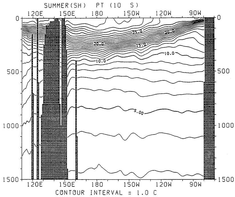
図 3.1.71 夏季 (南半球) におけるポテンシャル水温の東西断面分布 (10°S)
