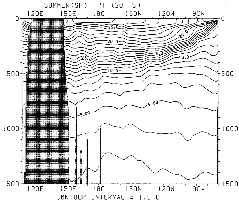
図 3.1.72 夏季 (南半球) におけるポテンシャル水温の東西断面分布 (20°S)
