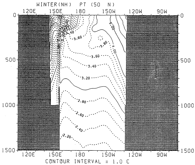
図 3.1.65 冬季におけるポテンシャル水温の東西断面分布 (50°N)
