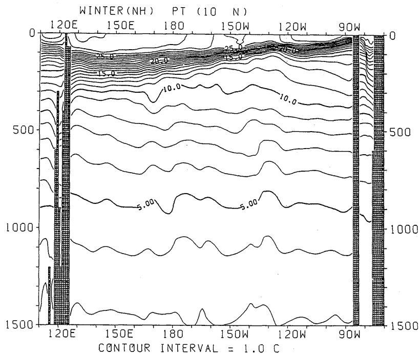
図 3.1.69 冬季におけるポテンシャル水温の東西断面分布 (10°N)
