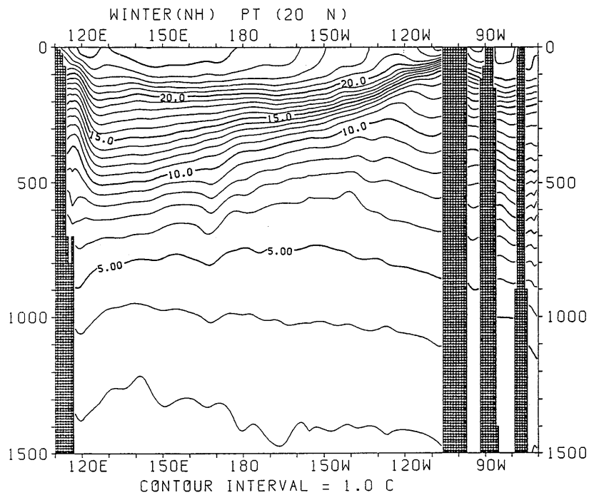
図 3.1.68 冬季におけるポテンシャル水温の東西断面分布 (20°N)
