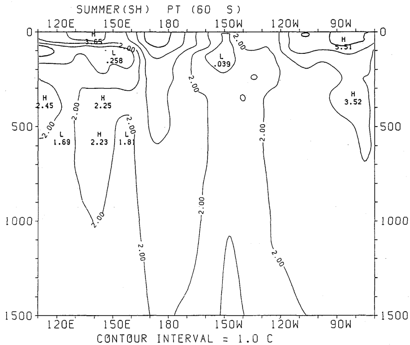
図 3.1.76 夏季(南半球)におけるポテンシャル水温の東西断面分布 (60°S)
