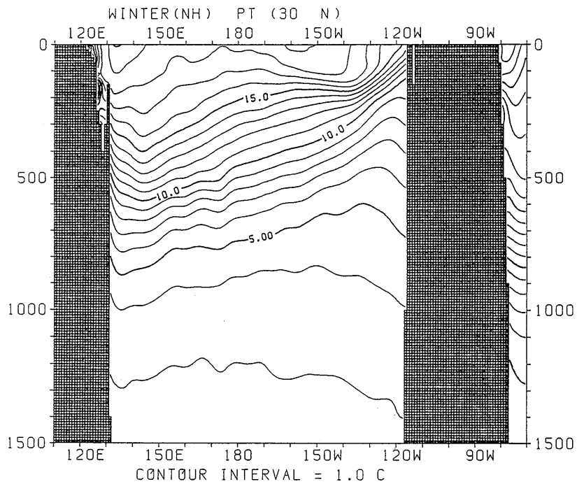
図 3.1.67 冬季におけるポテンシャル水温の東西断面分布 (30°N)
