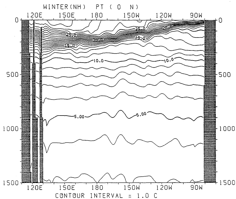
図 3.1.70 冬季におけるポテンシャル水温の東西断面分布 (赤道)
