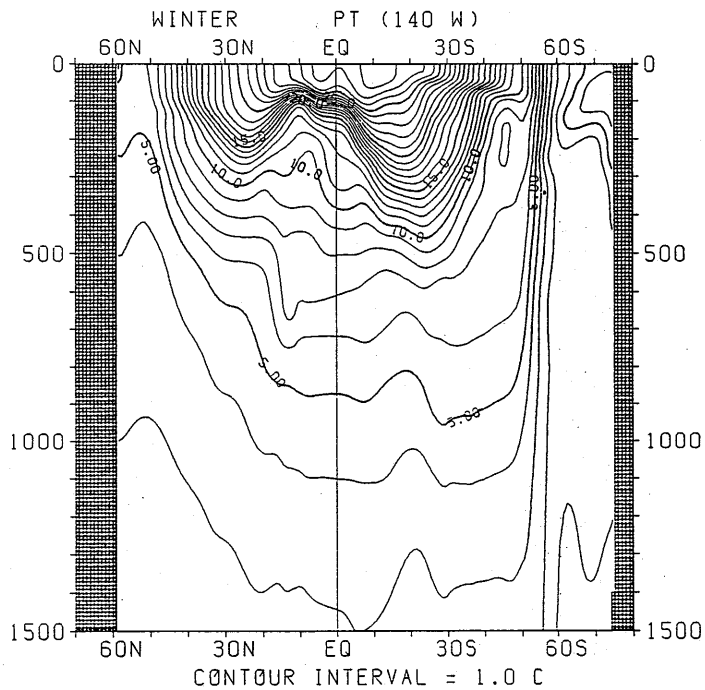
図 3.1.10 冬季におけるポテンシャル水温の南北断面分布 (140°W)
