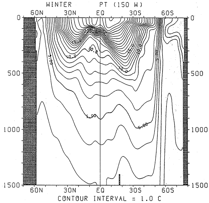
図 3.1.9 冬季におけるポテンシャル水温の南北断面分布 (150°W)
