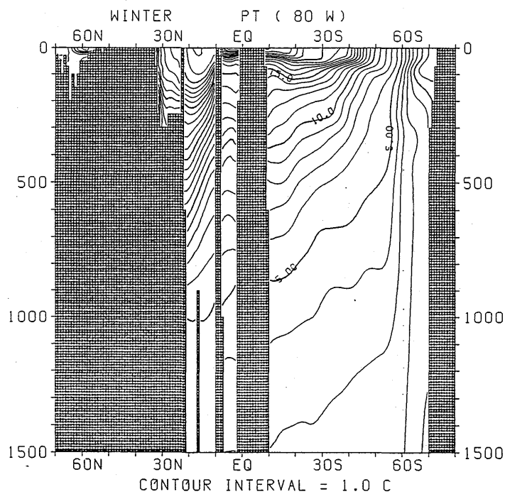
図 3.1.16 冬季におけるポテンシャル水温の南北断面分布 (80°W)
