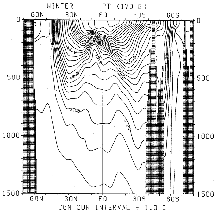
図 3.1.5 冬季におけるポテンシャル水温の南北断面分布 (170°E)
