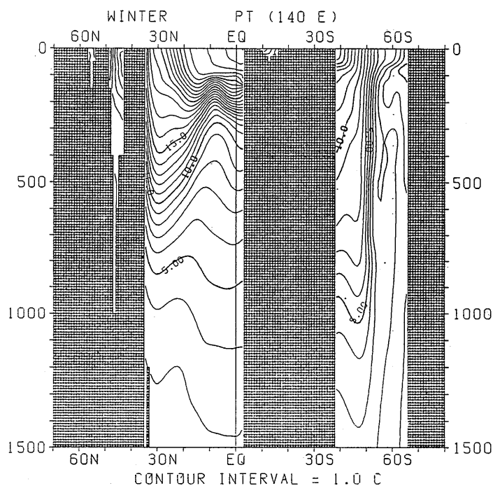
図 3.1.2 冬季におけるポテンシャル水温の南北断面分布 (140°E)
