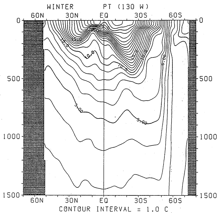
図 3.1.11 冬季におけるポテンシャル水温の南北断面分布 (130°W)
