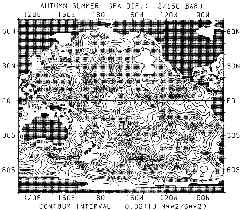
図 2.4.18 GPA の差の水平分布 (秋季—夏季) (20m)
