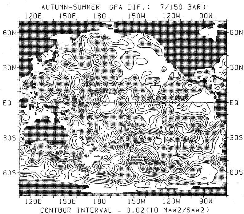
図 2.4.20 GPA の差の水平分布 (秋季—夏季) (75m)
