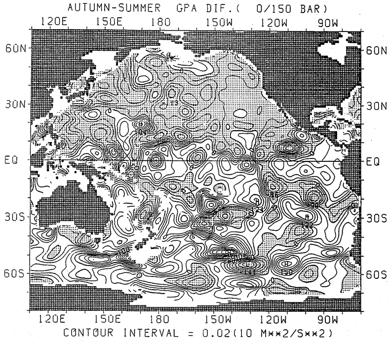
図 2.4.17 GPA の差の水平分布 (秋季—夏季) (海面)
