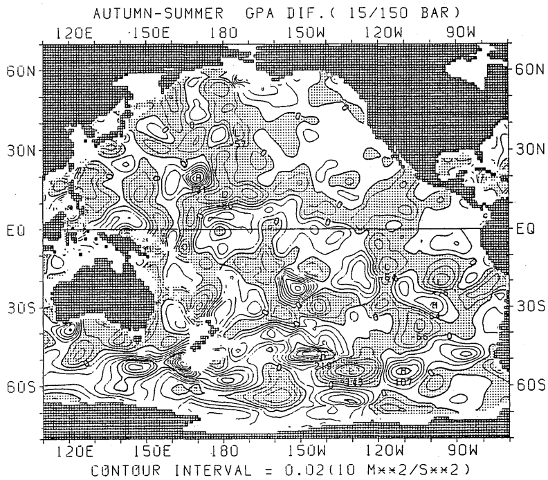
図 2.4.22 GPA の差の水平分布 (秋季—夏季) (150m)
