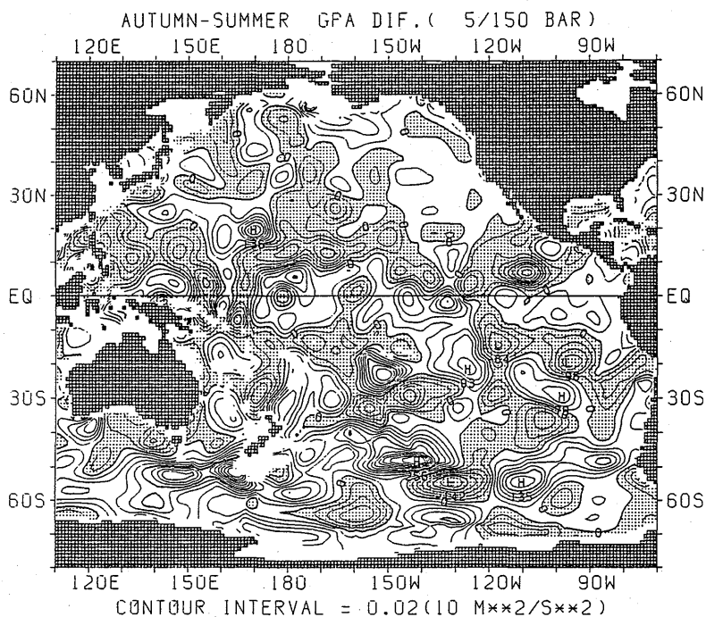
図 2.4.19 GPA の差の水平分布 (秋季—夏季) (50m)
