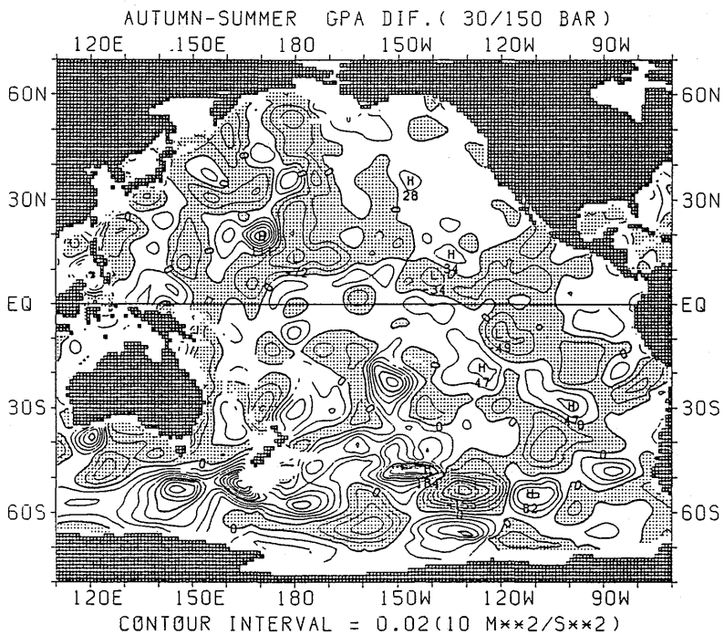
図 2.4.24 GPA の差の水平分布 (秋季—夏季) (300m)
