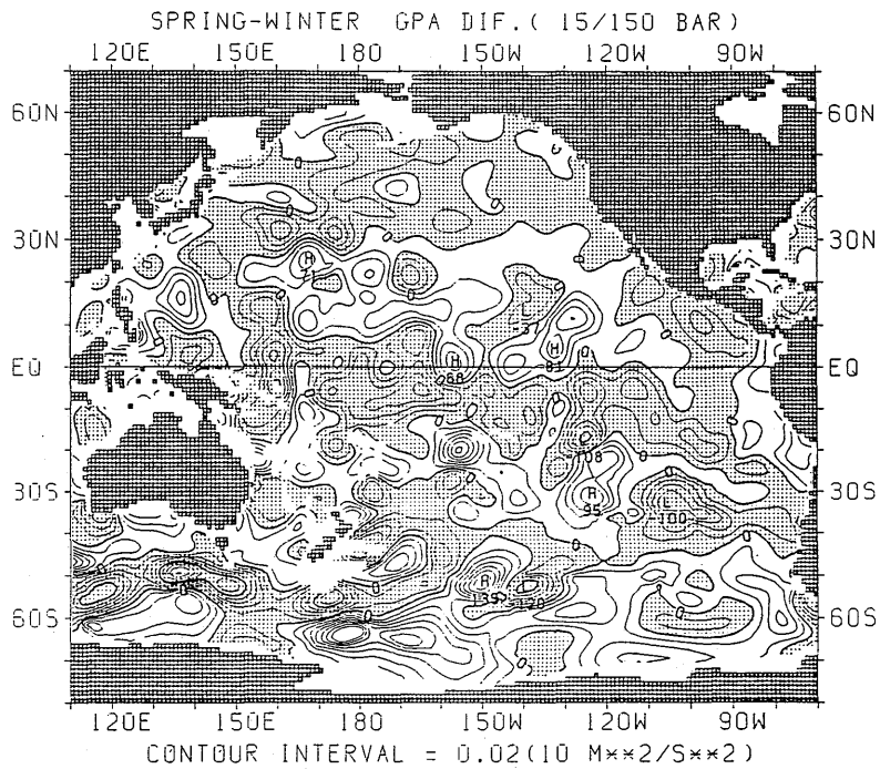
図 2.4.6 GPA の差の水平分布 (春季－冬季) (150m)
