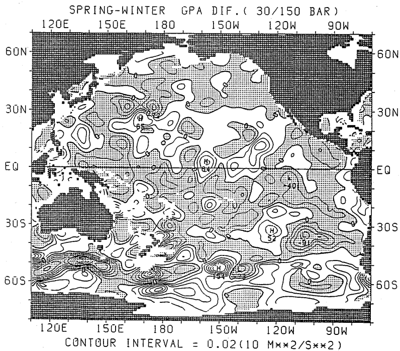
図 2.4.8 GPA の差の水平分布 (春季—冬季) (300m)
