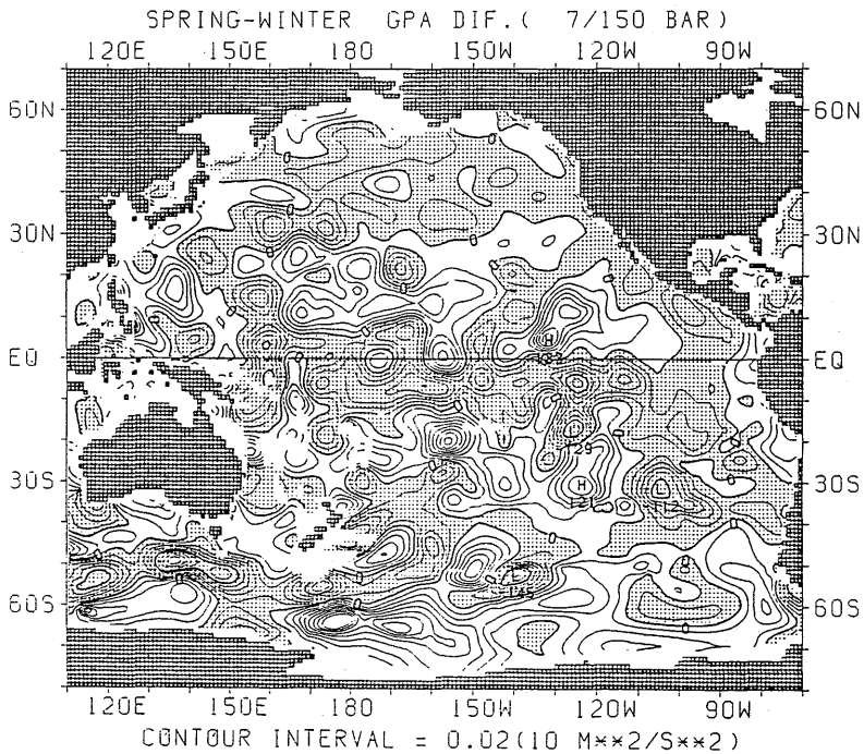
図 2.4.4 GPA の差の水平分布 (春季—冬季) (75m)
