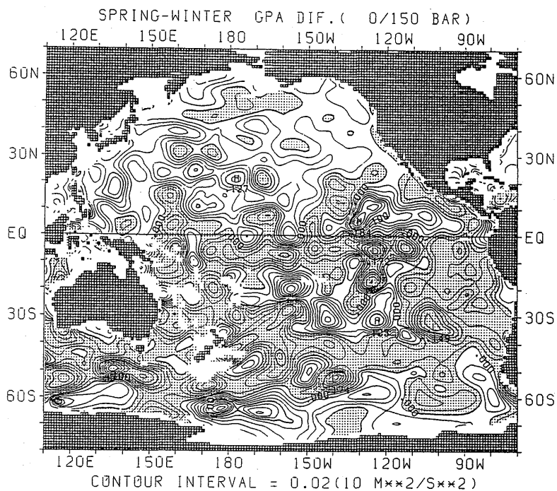
図 2.4.1 GPA の差の水平分布 (春季—冬季) (海面)
