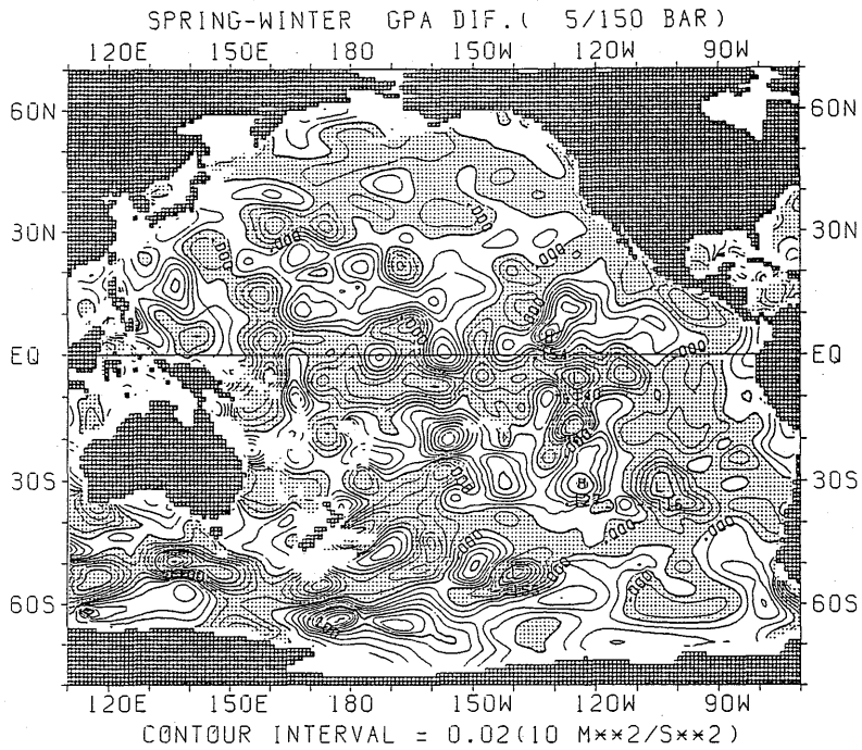
図 2.4.3 GPA の差の水平分布 (春季—冬季) (50m)
