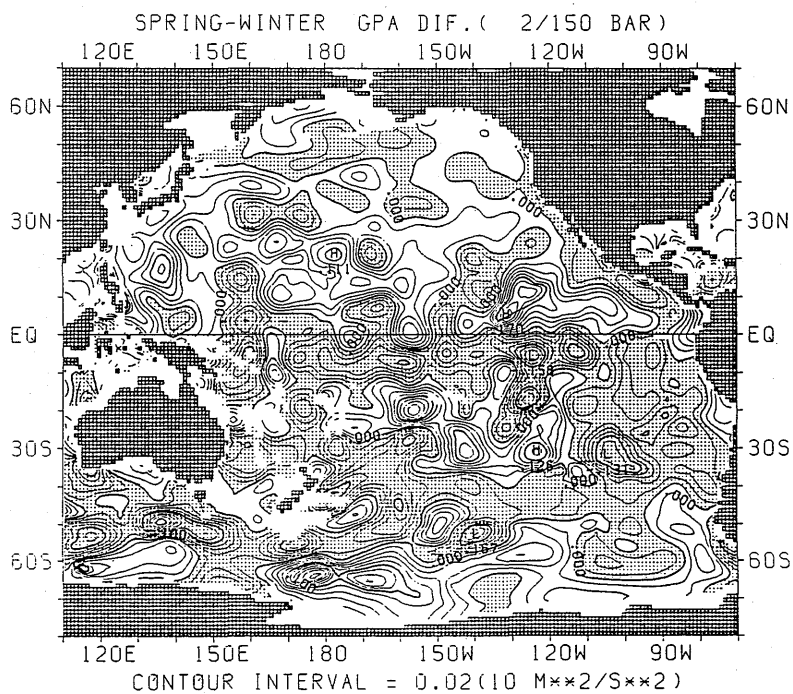
図 2.4.2 GPA の差の水平分布 (春季—冬季) (20m)
