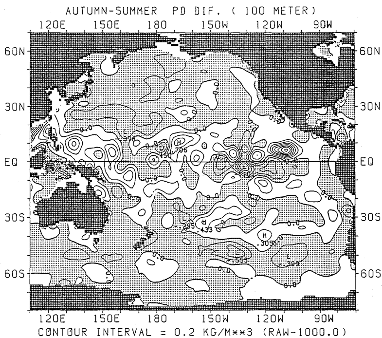
図 2.3.21 ポテンシャル密度の差の水平分布 (秋季—夏季) (100m)
