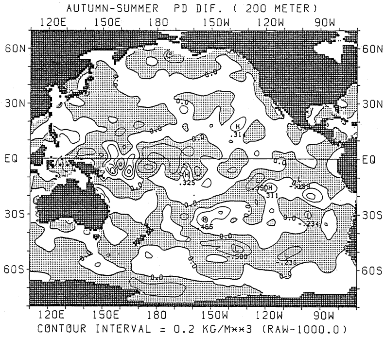
図 2.3.23 ポテンシャル密度の差の水平分布 (秋季—夏季) (200m)
