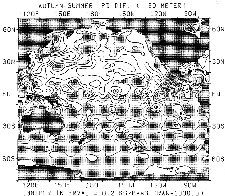
図 2.3.19 ポテンシャル密度の差の水平分布 (秋季—夏季) (50m)
