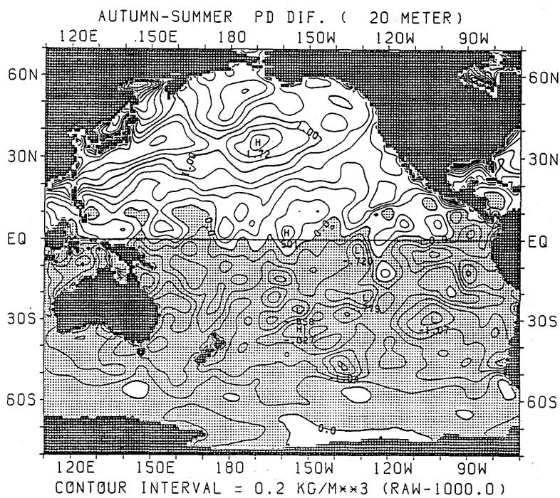
図 2.3.18 ポテンシャル密度の差の水平分布 (秋季—夏季) (20m)
