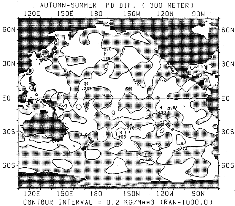
図 2.3.24 ポテンシャル密度の差の水平分布 (秋季—夏季) (300m)
