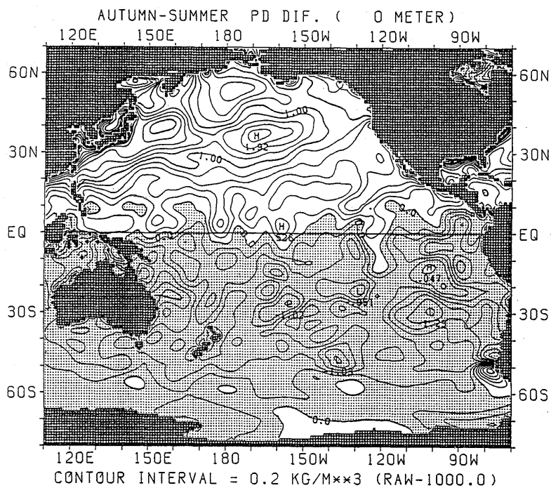
図 2.3.17 ポテンシャル密度の差の水平分布 (秋季—夏季) (海面)
