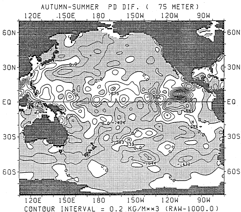
図 2.3.20 ポテンシャル密度の差の水平分布 (秋季—夏季) (75m)
