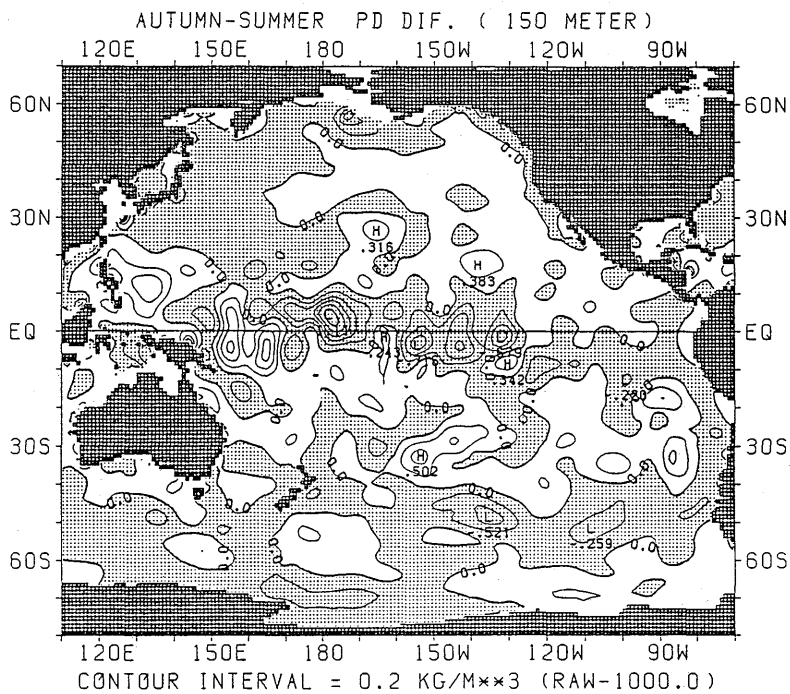
図 2.3.22 ポテンシャル密度の差の水平分布 (秋季—夏季) (150m)
