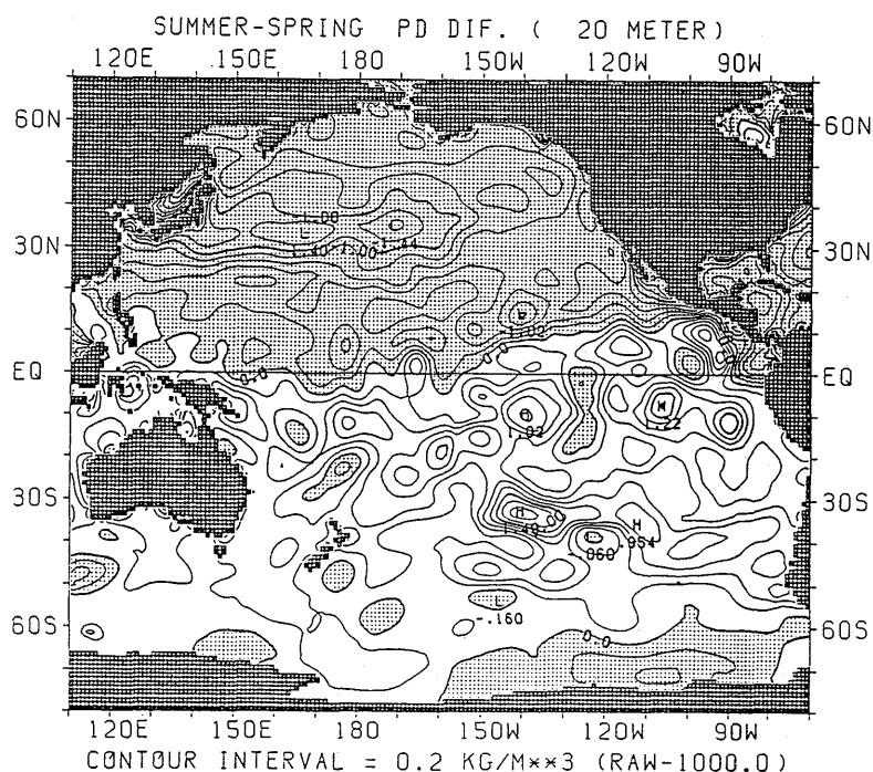
図 2.3.10 ポテンシャル密度の差の水平分布 (夏季—春季) (20m)
