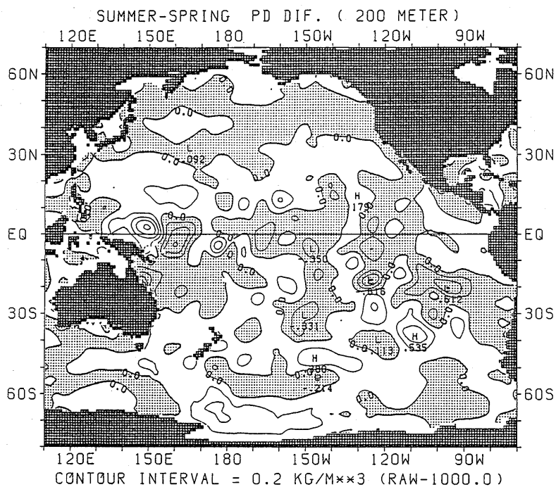
図 2.3.15 ポテンシャル密度の差の水平分布 (夏季—春季) (200m)
