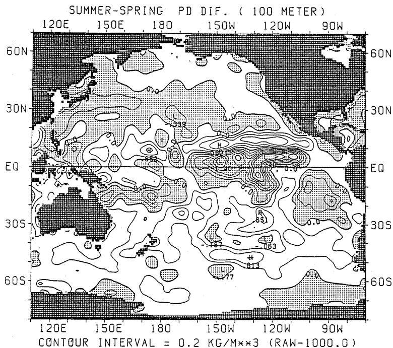
図 2.3.13 ポテンシャル密度の差の水平分布 (夏季—春季) (100m)
