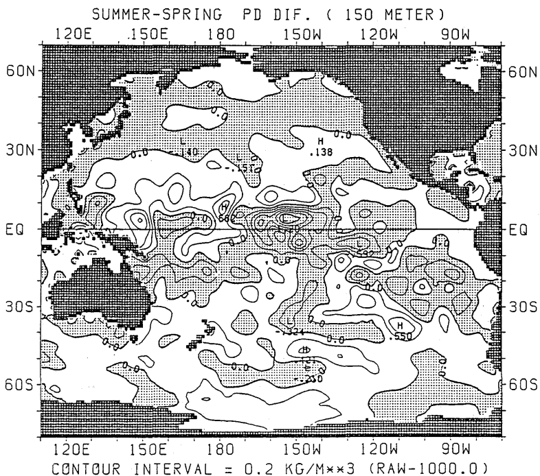
図 2.3.14 ポテンシャル密度の差の水平分布 (夏季－春季) (150m)
