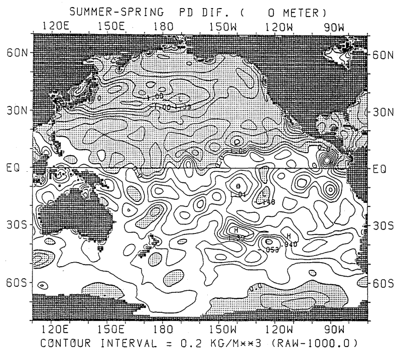
図 2.3.9 ポテンシャル密度の差の水平分布 (夏季—春季) (海面)
