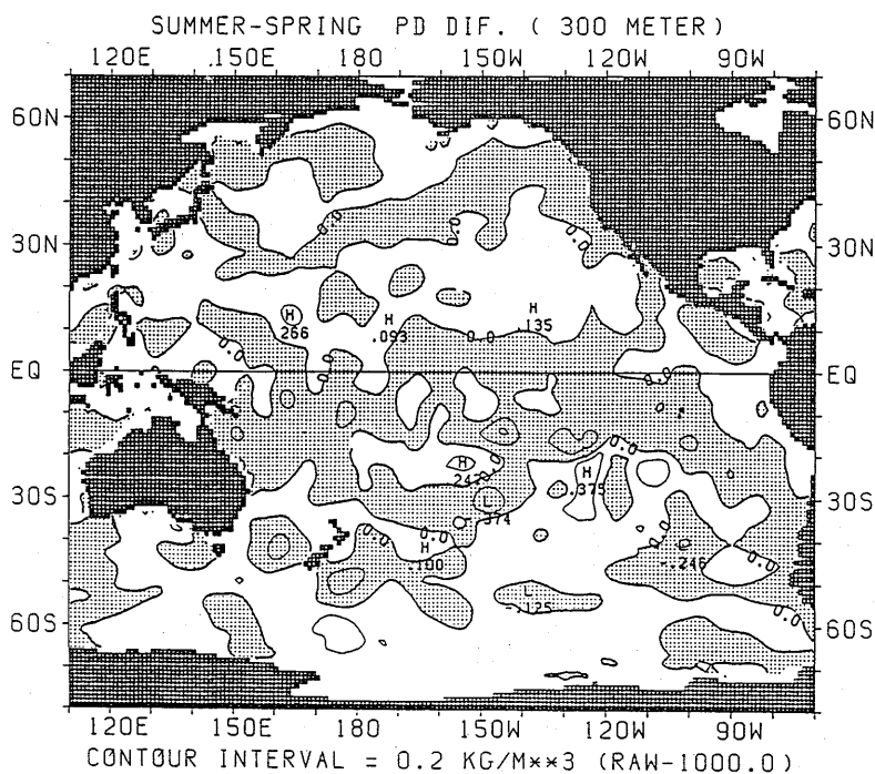
図 2.3.16 ポテンシャル密度の差の水平分布 (夏季—春季) (300m)
