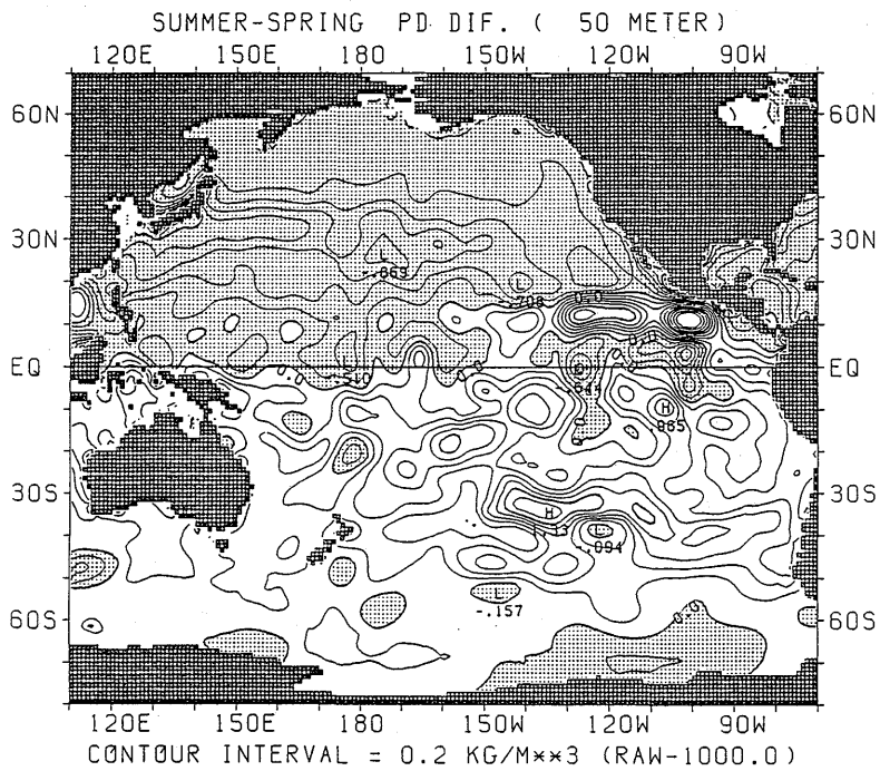
図 2.3.11 ポテンシャル密度の差の水平分布 (夏季－春季) (50m)
