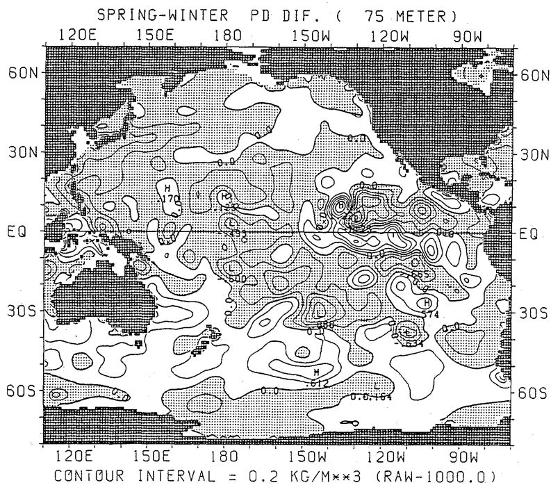
図 2.3.4 ポテンシャル密度の差の水平分布 (春季—冬季) (75m)
