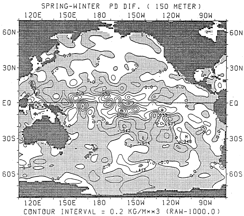
図 2.3.6 ポテンシャル密度の差の水平分布 (春季—冬季) (150m)
