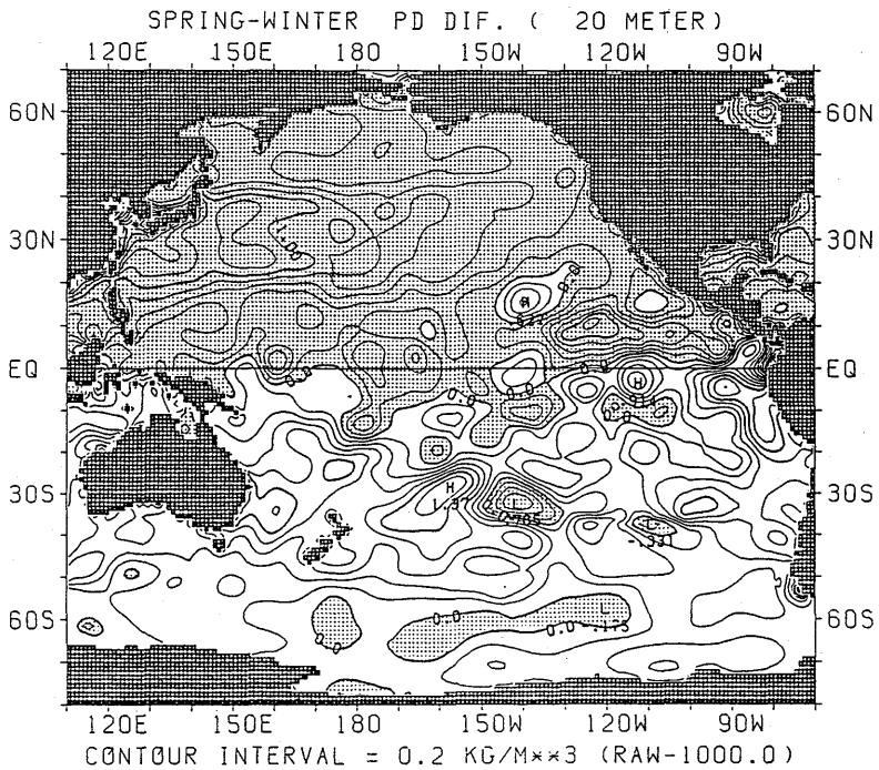
図 2.3.2 ポテンシャル密度の差の水平分布 (春季—冬季) (20m)
