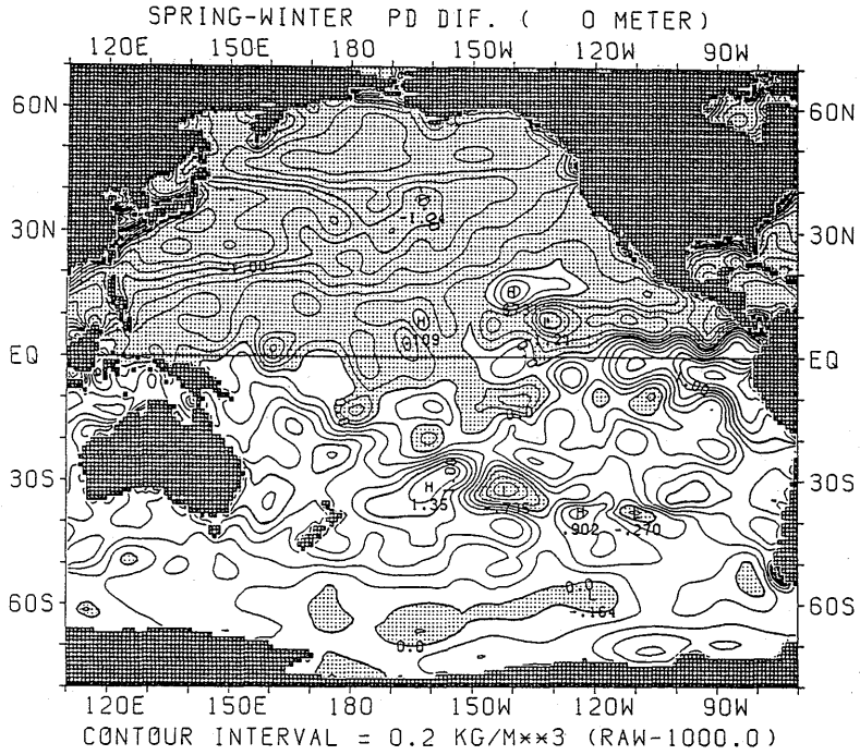
図 2.3.1 ポテンシャル密度の差の水平分布 (春季—冬季) (海面)
