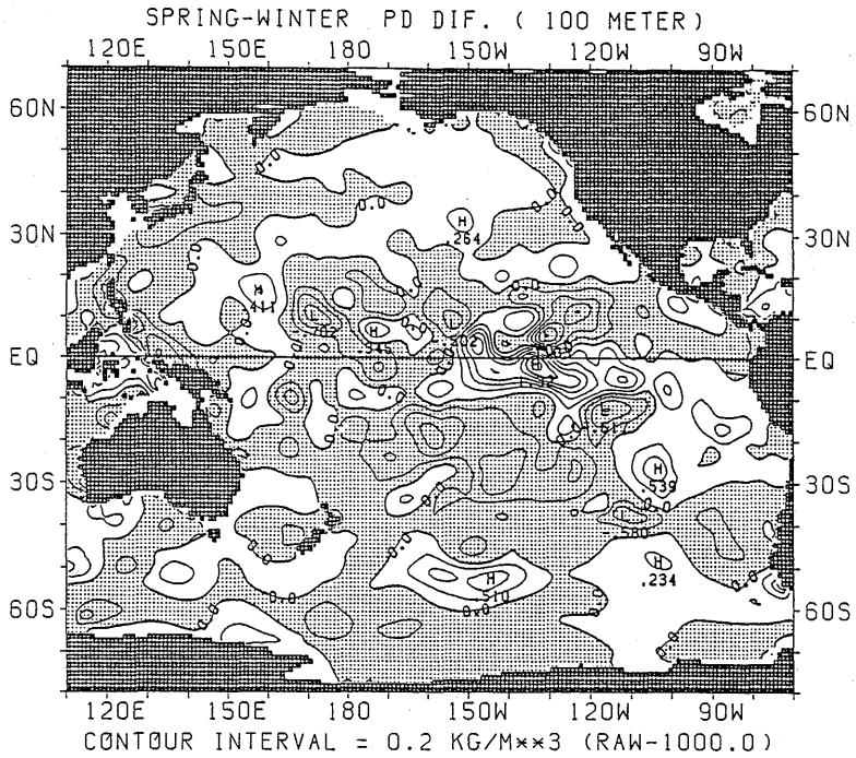
図 2.3.5 ポテンシャル密度の差の水平分布 (春季—冬季) (100m)
