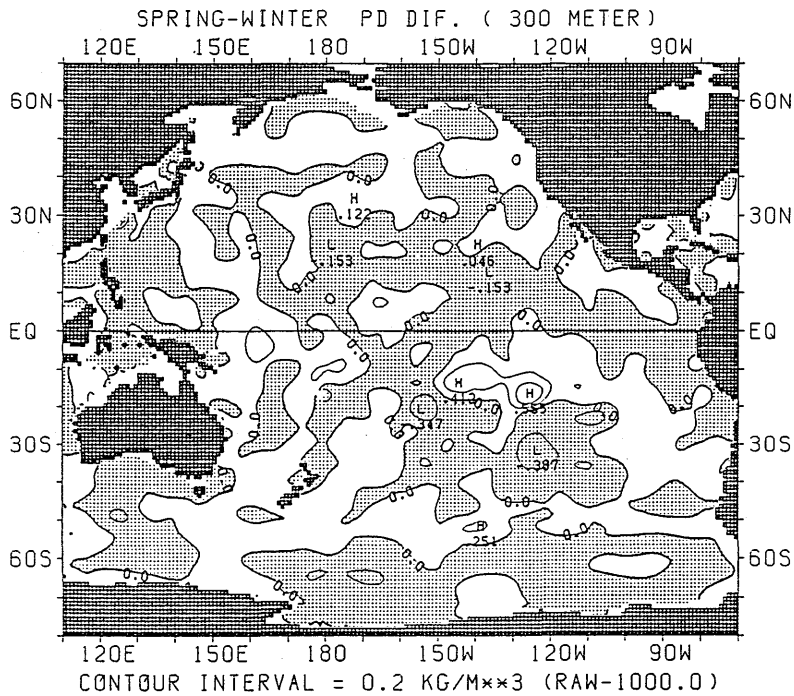
図 2.3.8 ポテンシャル密度の差の水平分布 (春季—冬季) (300m)
