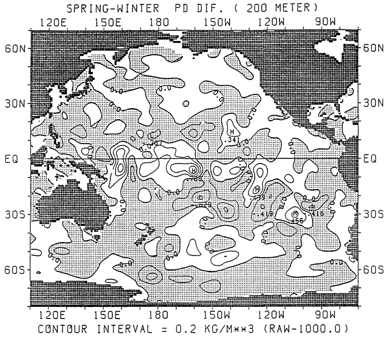
図 2.3.7 ポテンシャル密度の差の水平分布 (春季—冬季) (200m)
