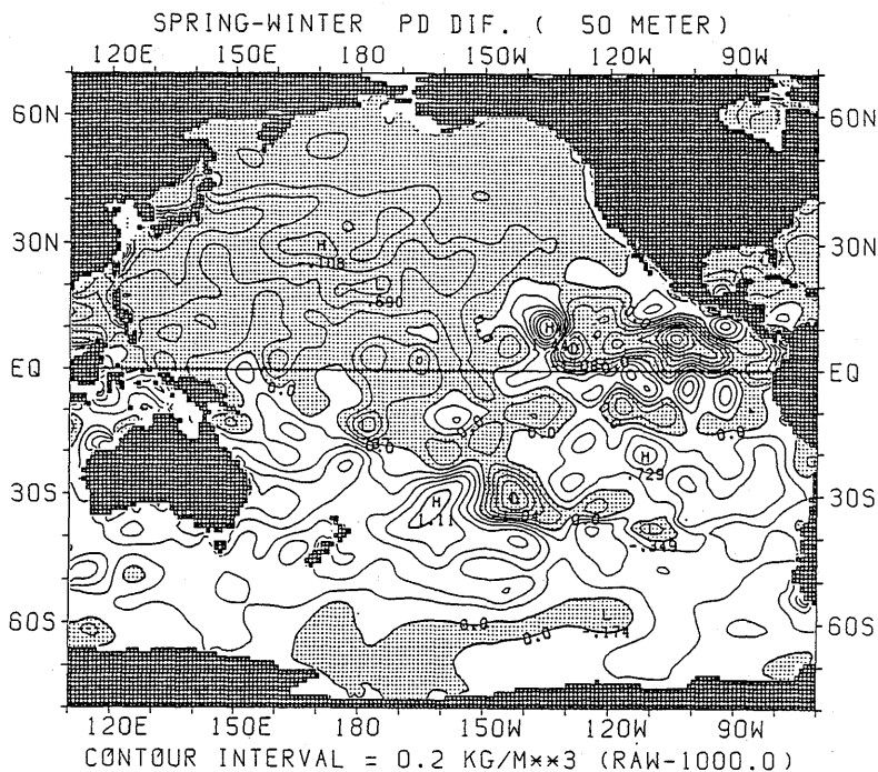
図 2.3.3 ポテンシャル密度の差の水平分布 (春季—冬季) (50m)
