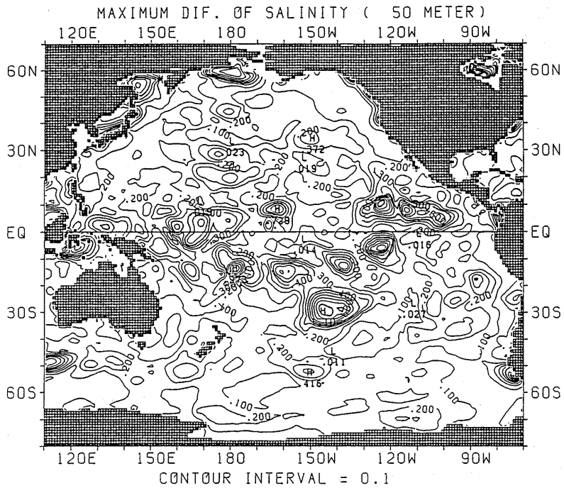
図 2.2.35 塩分年較差の水平分布 (50m)
