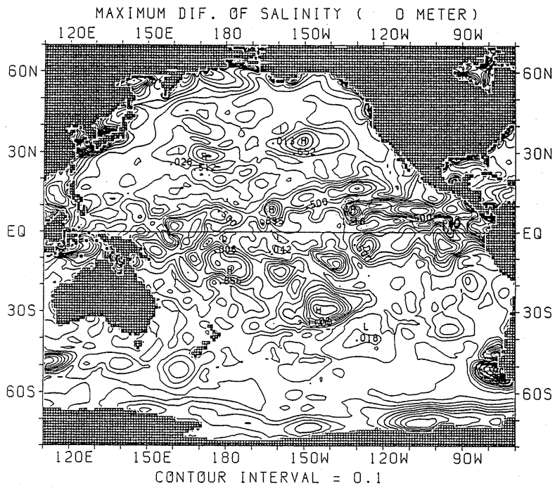
図 2.2.33 塩分年較差の水平分布 (海面)
