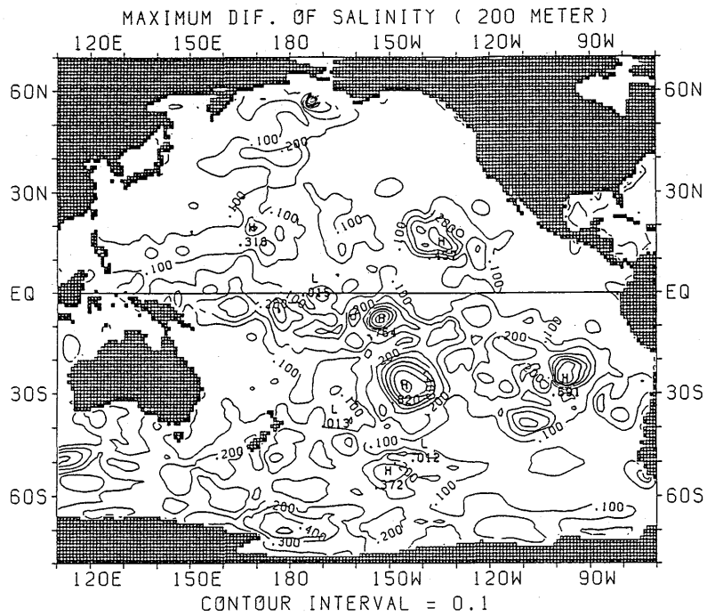
図 2.2.39 塩分年較差の水平分布 (200m)
