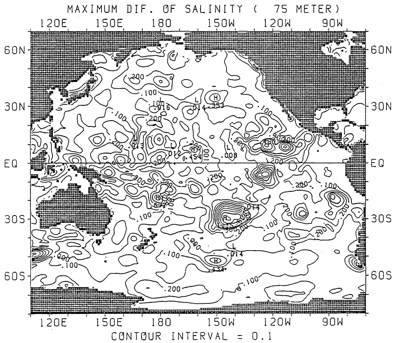
図 2.2.36 塩分年較差の水平分布 (75m)
