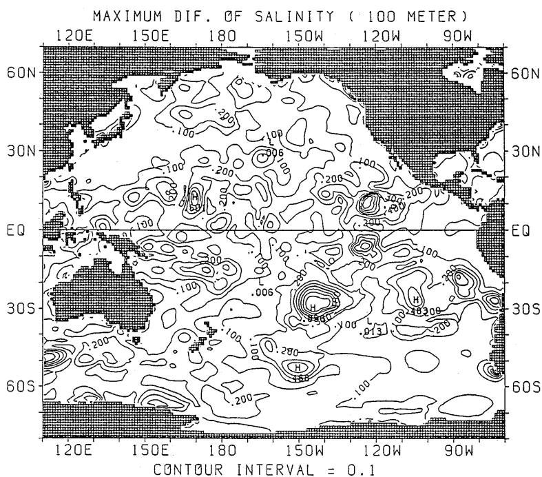
図 2.2.37 塩分年較差の水平分布 (100m)
