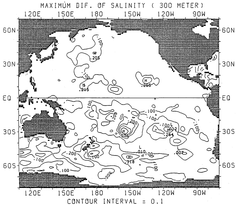
図 2.2.40 塩分年較差の水平分布 (300m)
