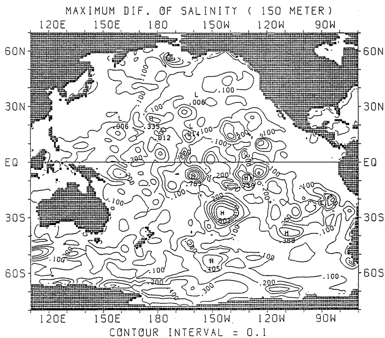
図 2.2.38 塩分年較差の水平分布 (150m)
