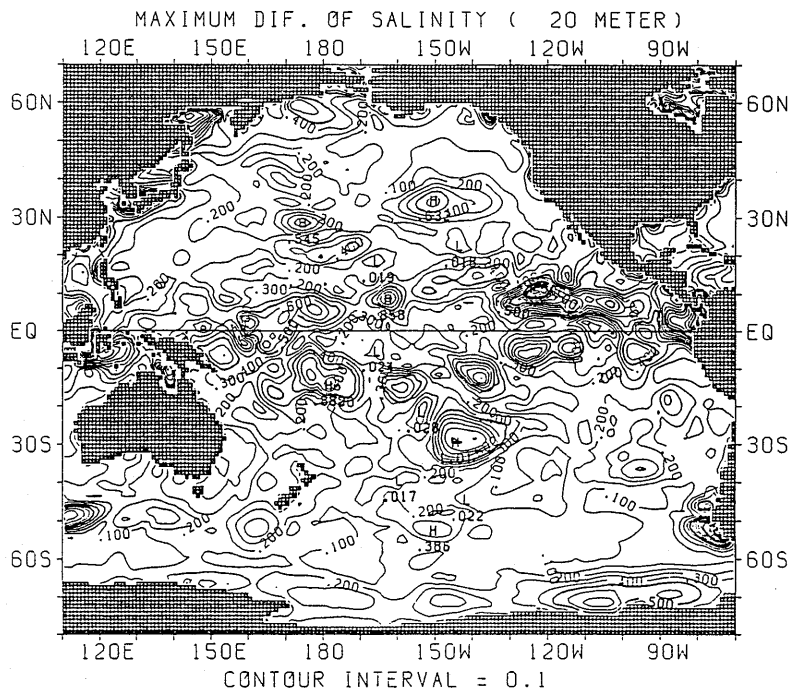
図 2.2.34 塩分年較差の水平分布 (20m)
