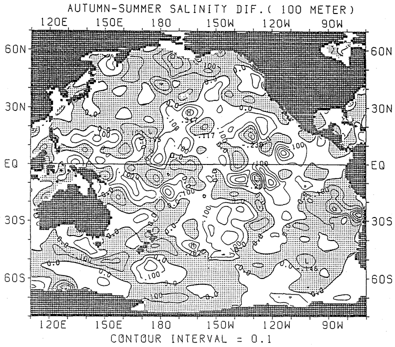
図 2.2.21 塩分の差の水平分布 (秋季—夏季) (100m)
