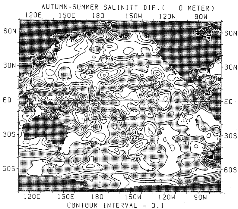
図 2.2.17 塩分の差の水平分布 (秋季—夏季) (海面)
