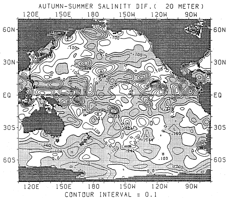
図 2.2.18 塩分の差の水平分布 (秋季—夏季) (20m)
