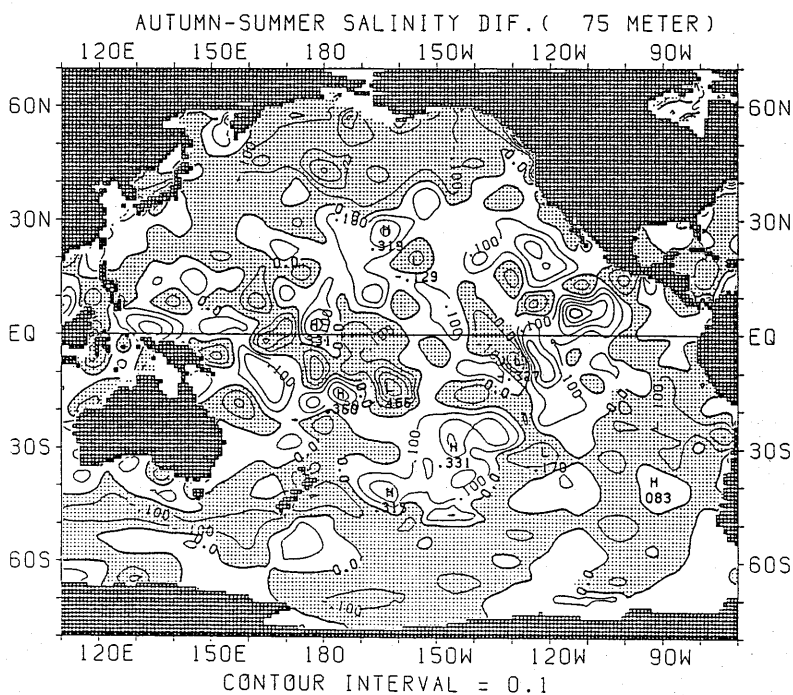
図 2.2.20 塩分の差の水平分布 (秋季—夏季) (75m)
