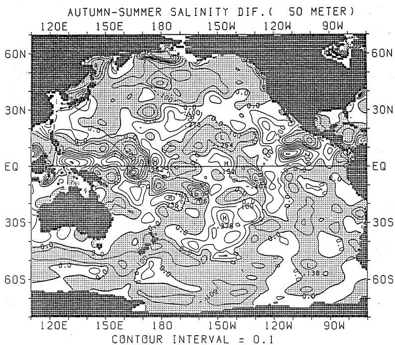
図 2.2.19 塩分の差の水平分布 (秋季—夏季) (50m)
