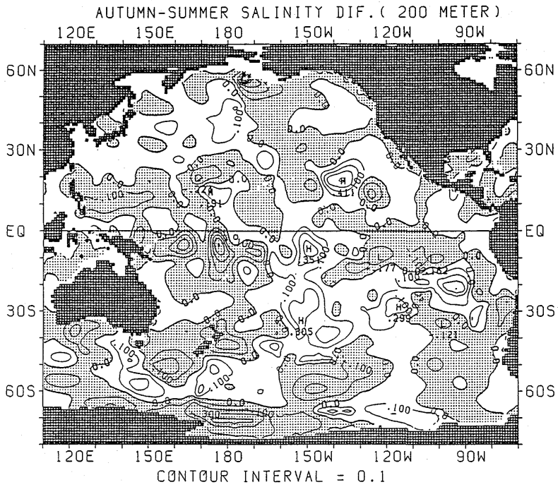
図 2.2.23 塩分の差の水平分布 (秋季—夏季) (200m)
