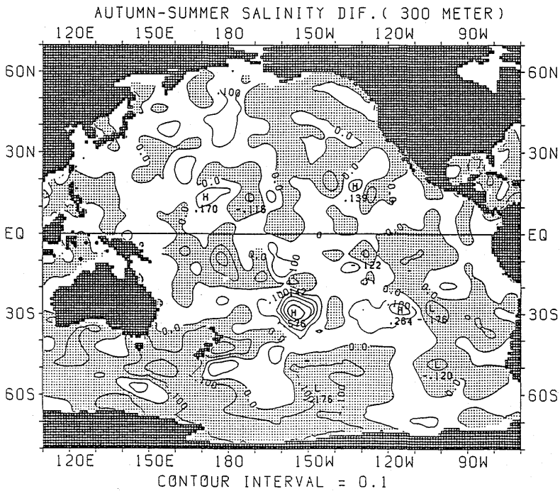
図 2.2.24 塩分の差の水平分布 (秋季—夏季) (300m)
