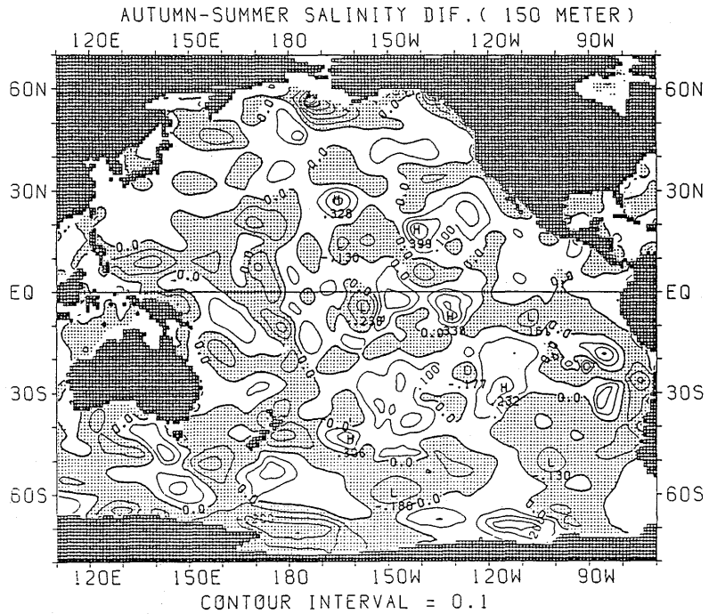
図 2.2.22 塩分の差の水平分布 (秋季—夏季) (150m)
