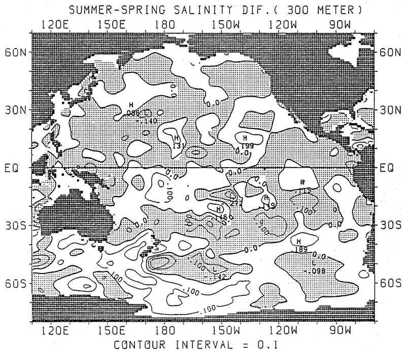
図 2.2.16 塩分の差の水平分布 (夏季—春季) (300m)
