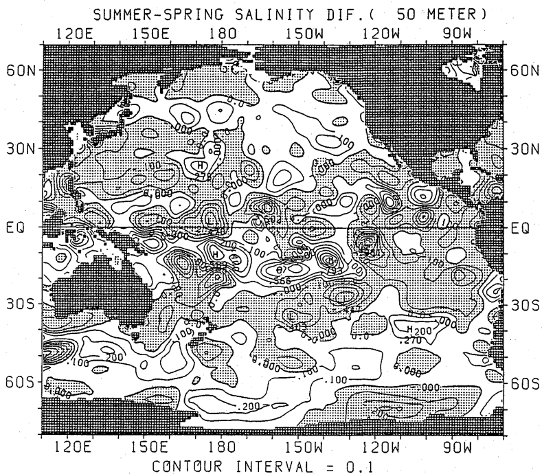
図 2.2.11 塩分の差の水平分布 (夏季—春季) (50m)
