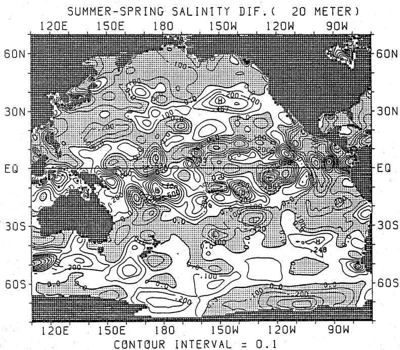
図 2.2.10 塩分の差の水平分布 (夏季－春季) (20m)
