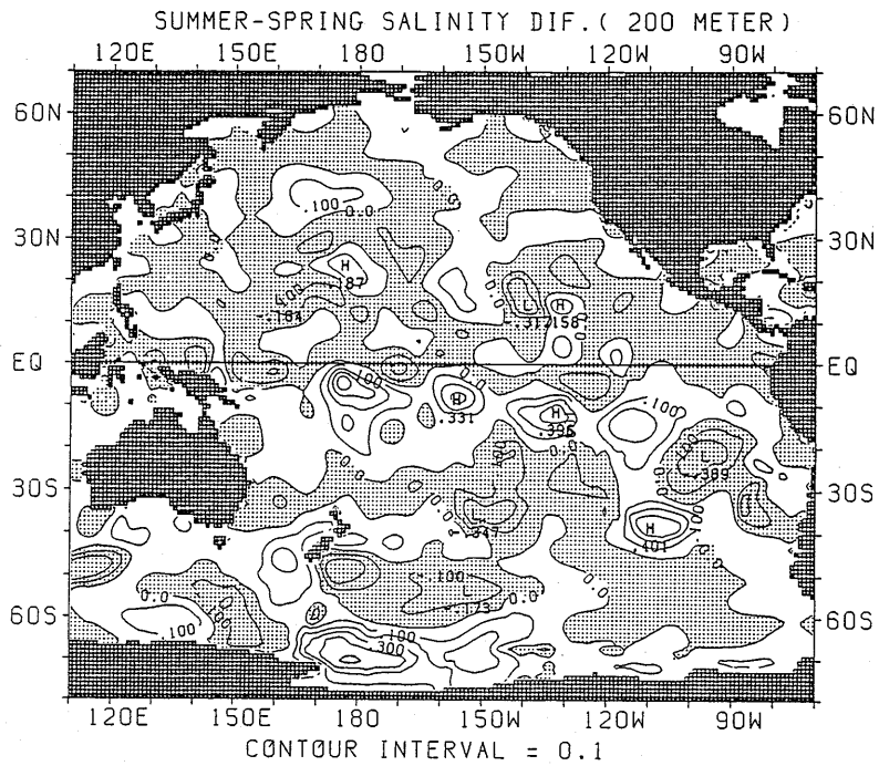
図 2.2.15 塩分の差の水平分布 (夏季—春季) (200m)
