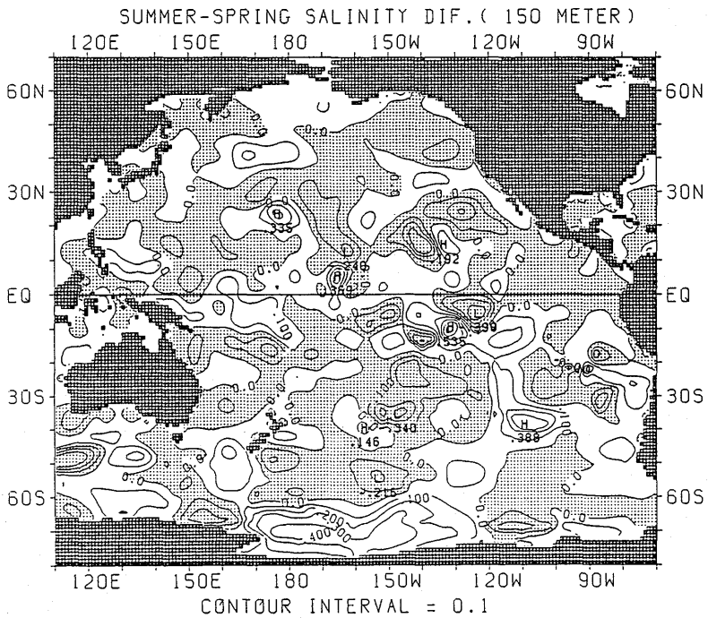
図 2.2.14 塩分の差の水平分布 (夏季—春季) (150m)
