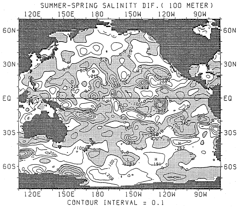
図 2.2.13 塩分の差の水平分布 (夏季—春季) (100m)
