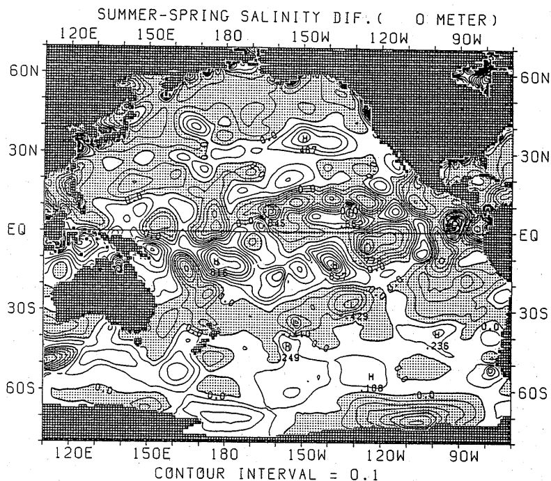
図 2.2.9 塩分の差の水平分布 (夏季－春季) (海面)
