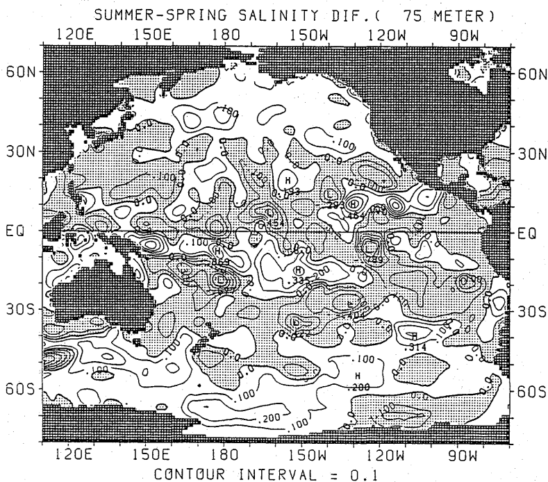
図 2.2.12 塩分の差の水平分布 (夏季—春季) (75m)
