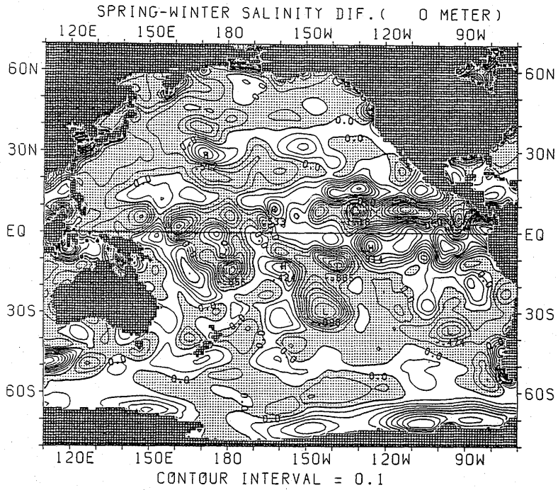
図 2.2.1 塩分の差の水平分布 (春季－冬季) (海面)
