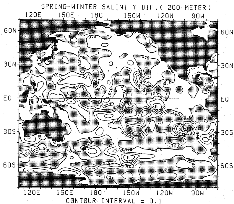
図 2.2.7 塩分の差の水平分布 (春季 - 冬季) (200m)
