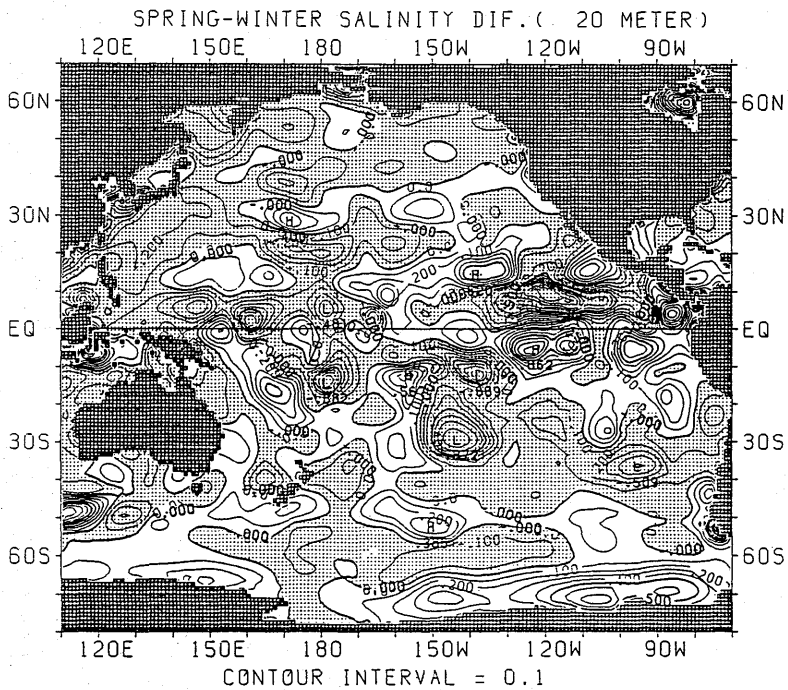
図 2.2.2 塩分の差の水平分布 (春季－冬季) (20m)
