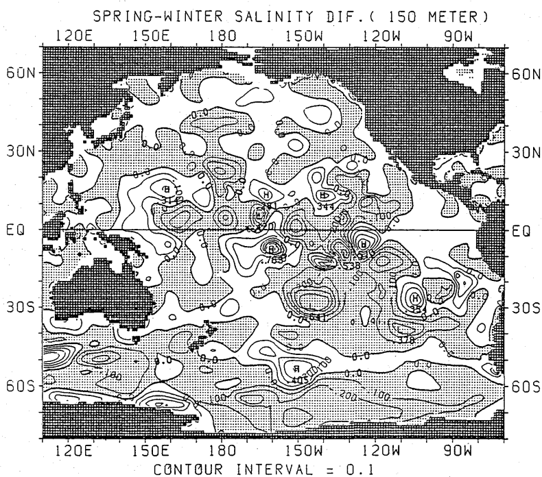
図 2.2.6 塩分の差の水平分布 (春季－冬季) (150m)
