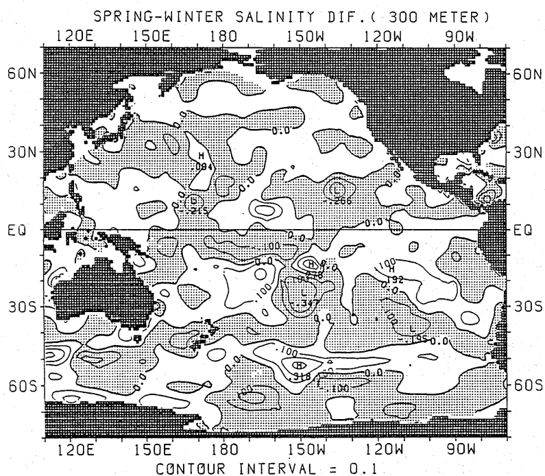
図 2.2.8 塩分の差の水平分布 (春季 - 冬季) (300m)
