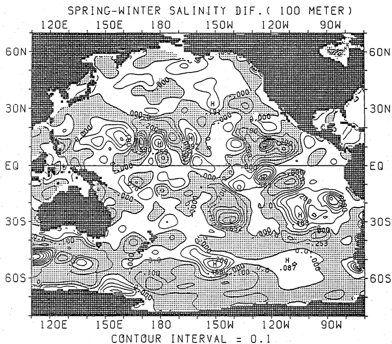
図 2.2.5 塩分の差の水平分布 (春季－冬季) (100m)
