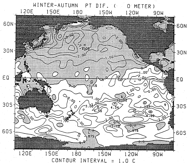
図 2.1.25 ポテンシャル水温の差の水平分布 (冬季—秋季) (海面)
