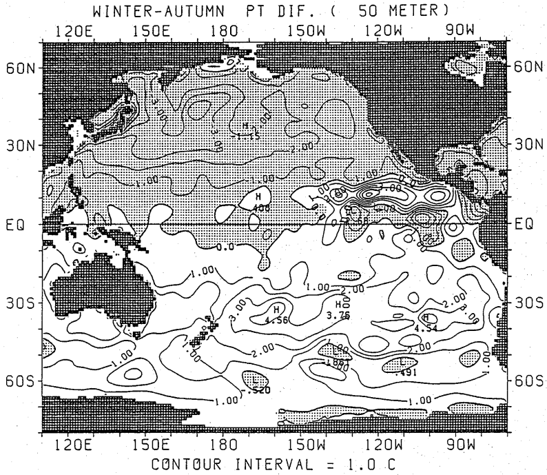
図 2.1.27 ポテンシャル水温の差の水平分布 (冬季—秋季) (50m)
