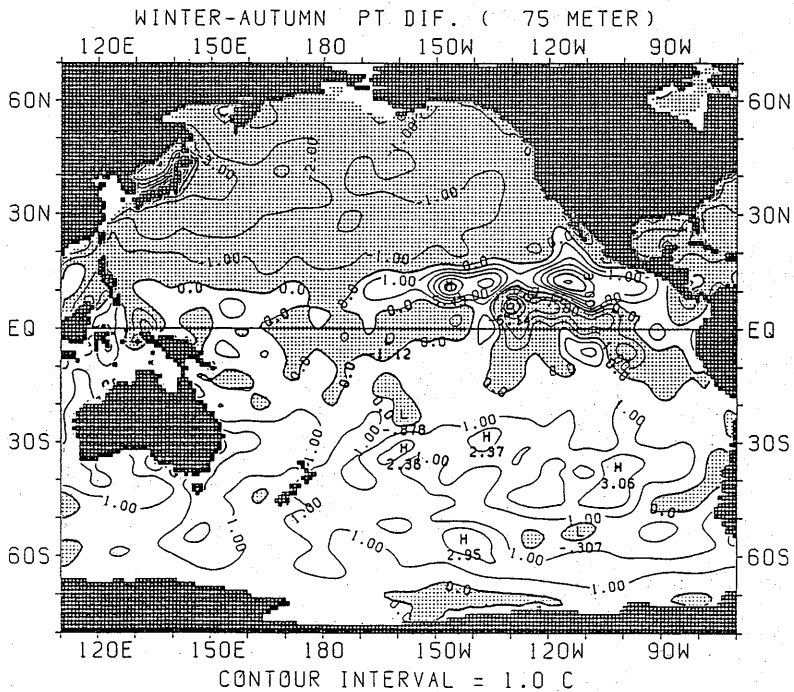
図 2.1.28 ポテンシャル水温の差の水平分布 (冬季—秋季) (75m)
