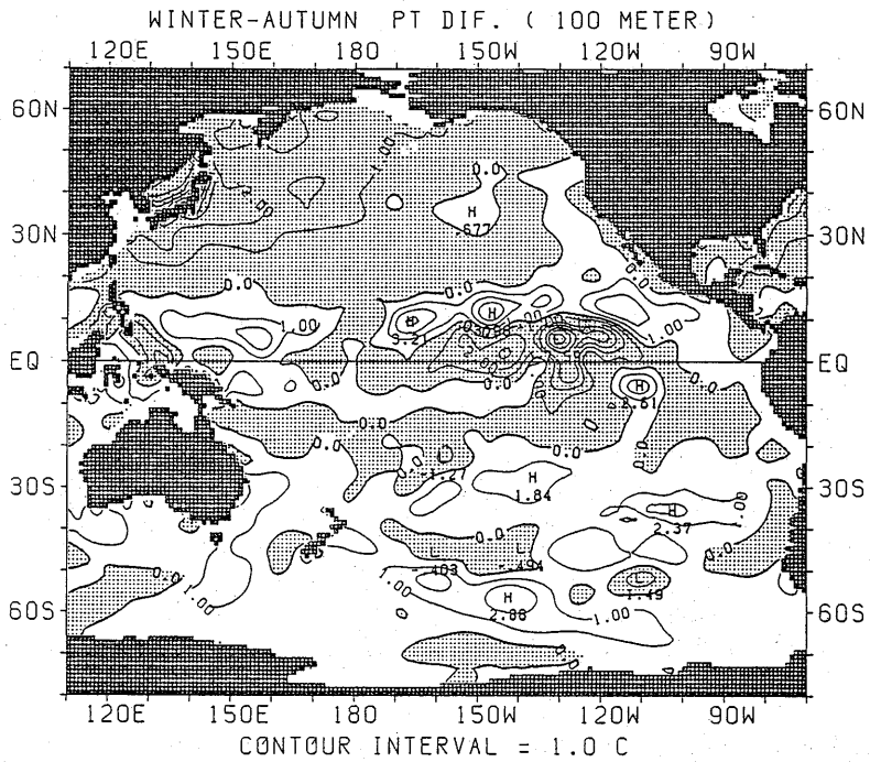
図 2.1.29 ポテンシャル水温の差の水平分布 (冬季—秋季) (100m)
