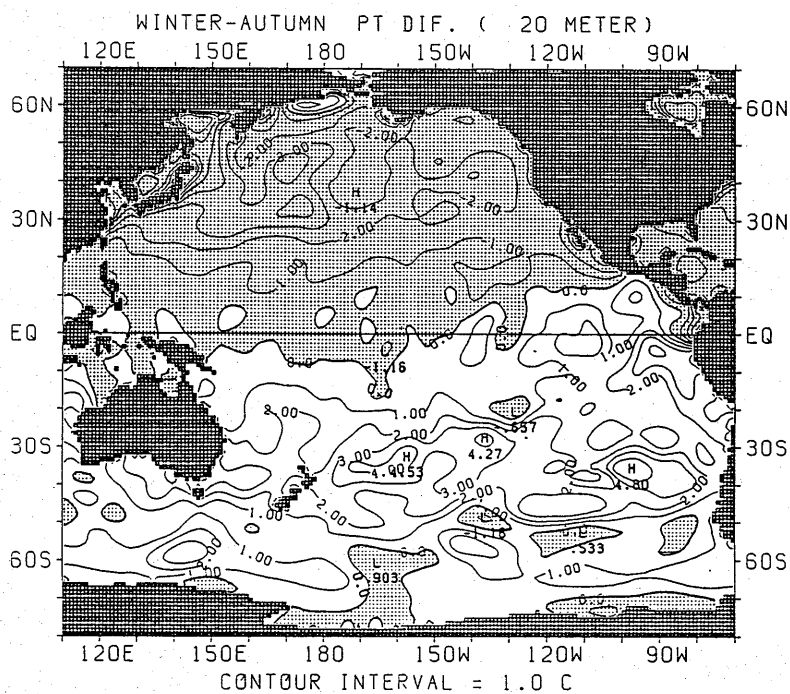
図 2.1.26 ポテンシャル水温の差の水平分布 (冬季—秋季) (20m)
