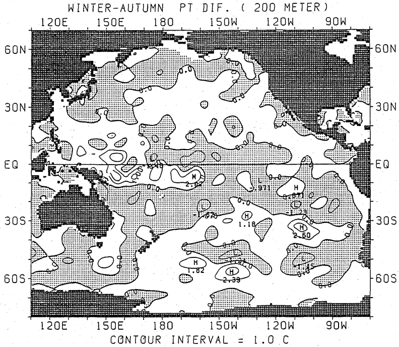
図 2.1.31 ポテンシャル水温の差の水平分布 (冬季—秋季) (200m)
