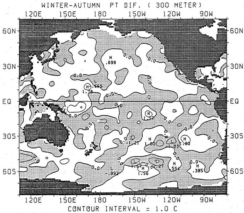
図 2.1.32 ポテンシャル水温の差の水平分布 (冬季—秋季) (300m)
