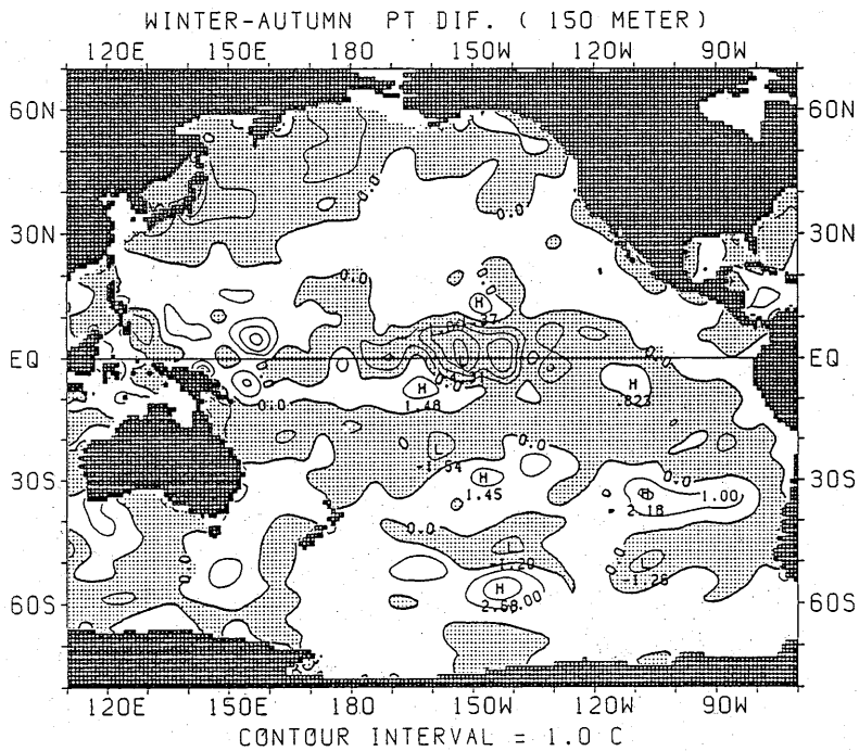
図 2.1.30 ポテンシャル水温の差の水平分布 (冬季—秋季) (150m)
