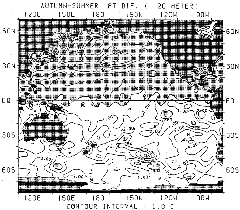
図 2.1.18 ポテンシャル水温の差の水平分布 (秋季－夏季) (20m)
