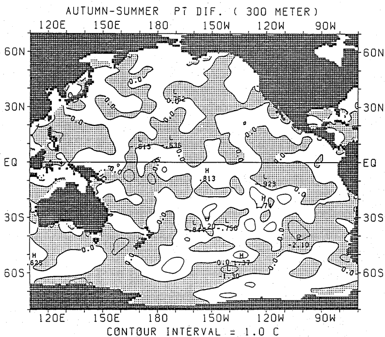
図 2.1.24 ポテンシャル水温の差の水平分布 (秋季—夏季) (300m)
