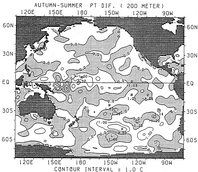
図 2.1.23 ポテンシャル水温の差の水平分布 (秋季—夏季) (200m)
