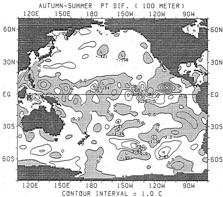
図 2.1.21 ポテンシャル水温の差の水平分布 (秋季—夏季) (100m)
