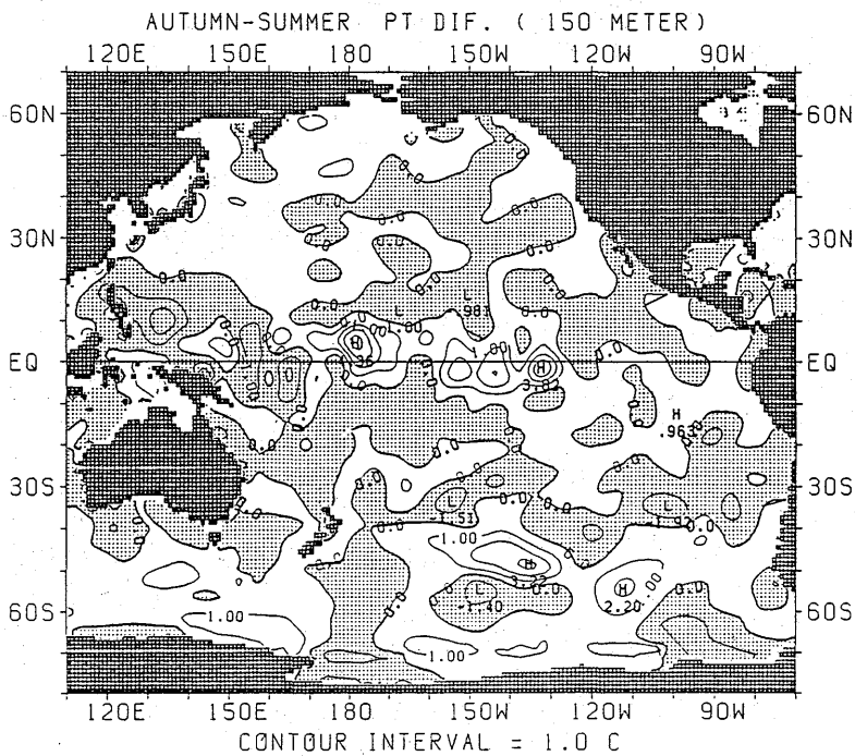
図 2.1.22 ポテンシャル水温の差の水平分布 (秋季—夏季) (150m)
