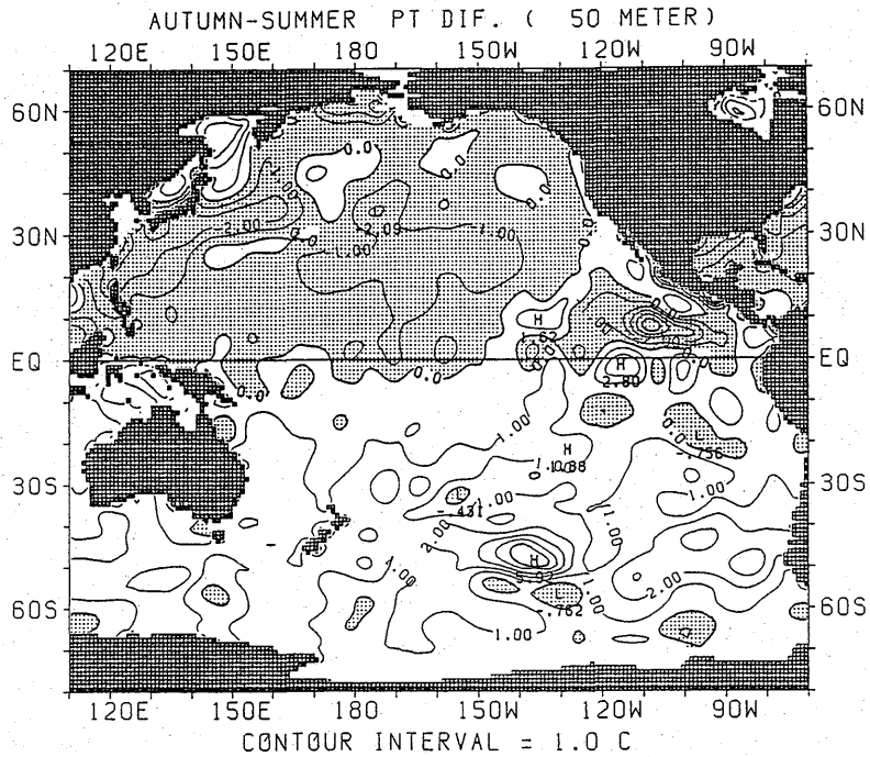
図 2.1.19 ポテンシャル水温の差の水平分布 (秋季—夏季) (50m)
