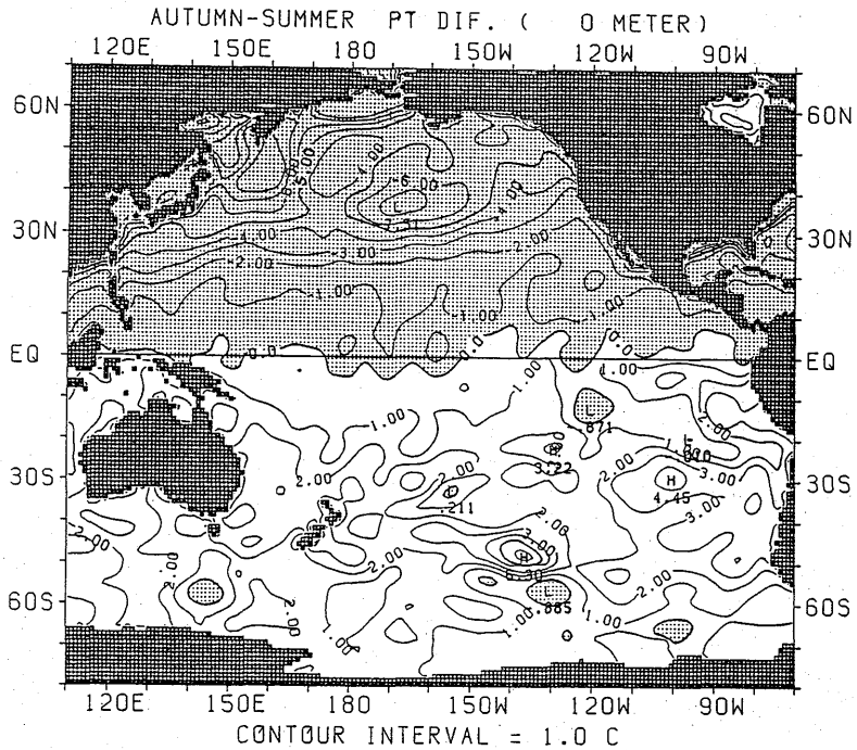
図 2.1.17 ポテンシャル水温の差の水平分布 (秋季－夏季) (海面)
