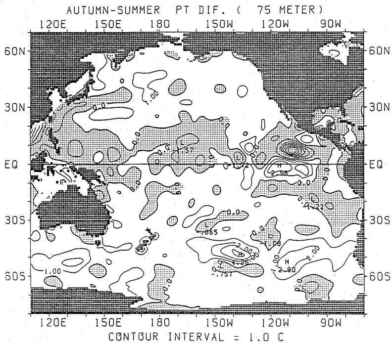
図 2.1.20 ポテンシャル水温の差の水平分布 (秋季—夏季) (75m)
