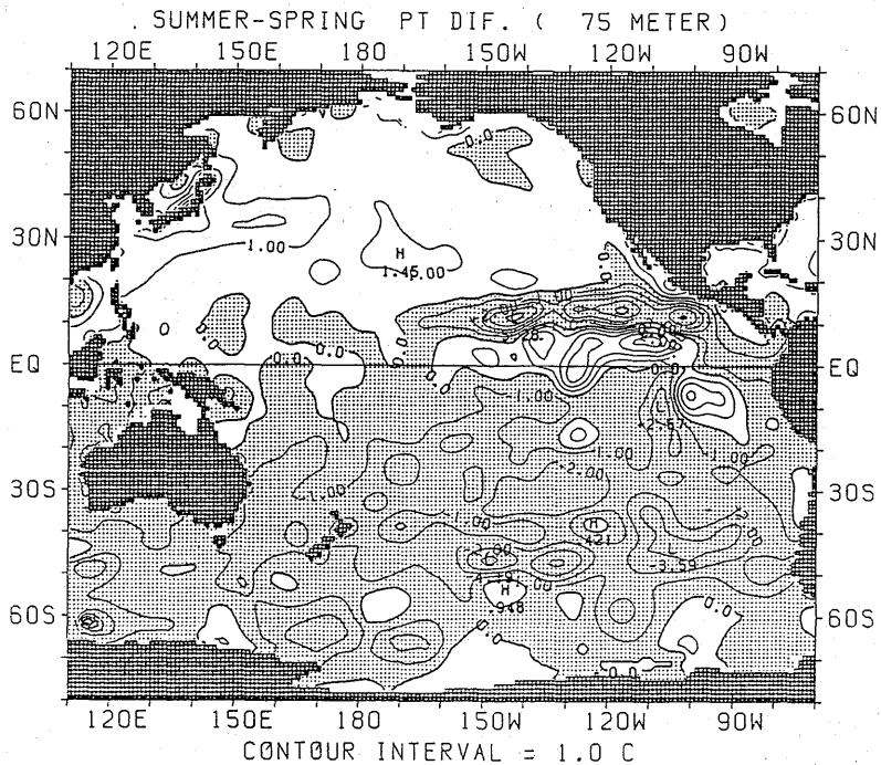
図 2.1.12 ポテンシャル水温の差の水平分布 (夏季—春季) (75m)
