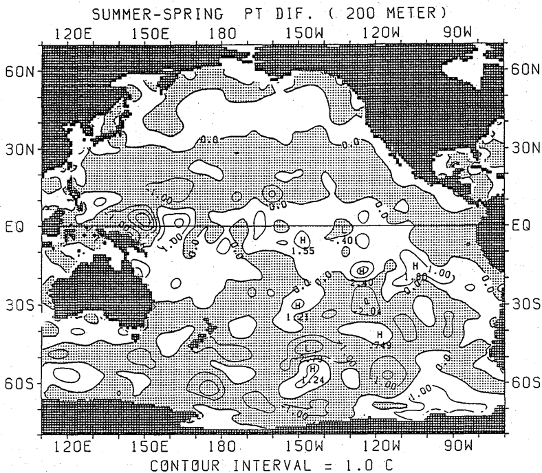
図 2.1.15 ポテンシャル水温の差の水平分布 (夏季—春季) (200m)
