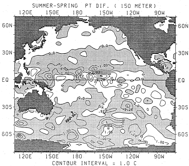
図 2.1.14 ポテンシャル水温の差の水平分布 (夏季－春季) (150m)
