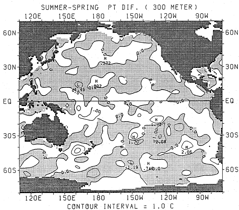
図 2.1.16 ポテンシャル水温の差の水平分布 (夏季—春季) (300m)
