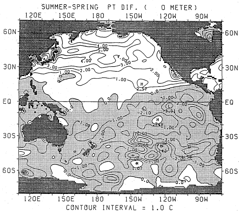
図 2.1.9 ポテンシャル水温の差の水平分布 (夏季—春季) (海面)
