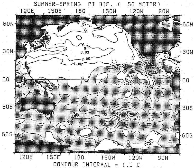
図 2.1.11 ポテンシャル水温の差の水平分布 (夏季—春季) (50m)
