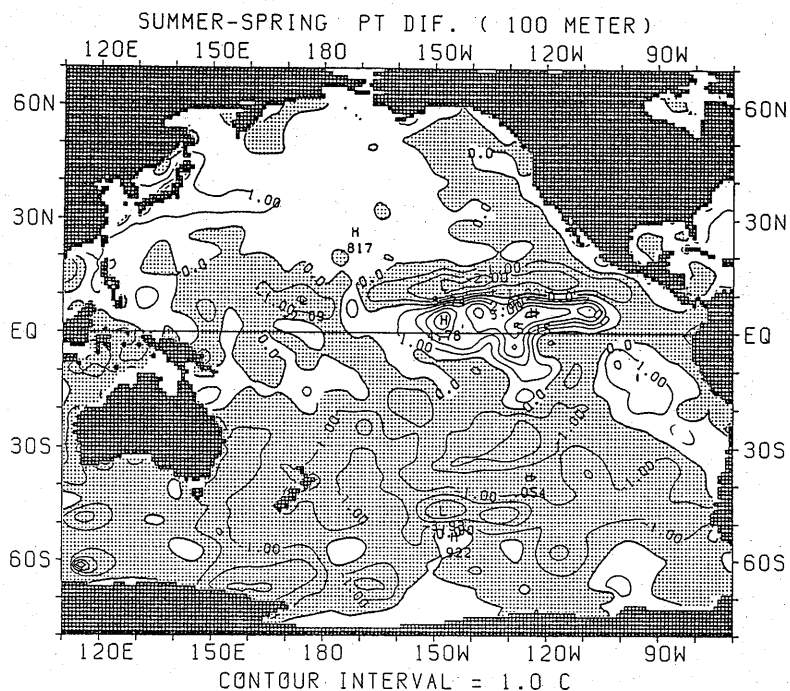
図 2.1.13 ポテンシャル水温の差の水平分布 (夏季－春季) (100m)
