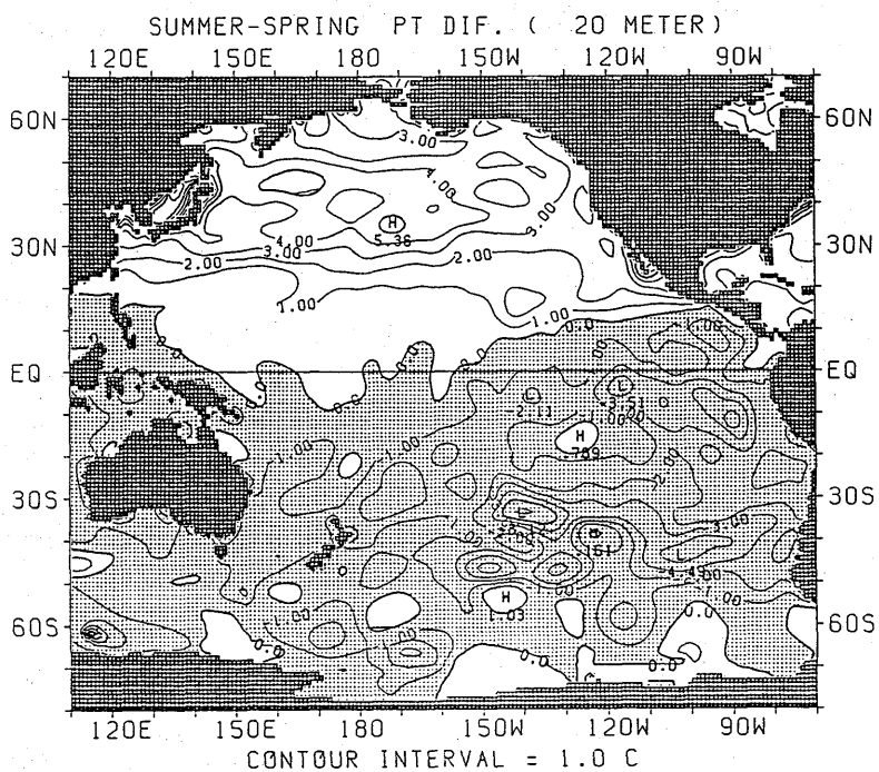
図 2.1.10 ポテンシャル水温の差の水平分布 (夏季—春季) (20m)
