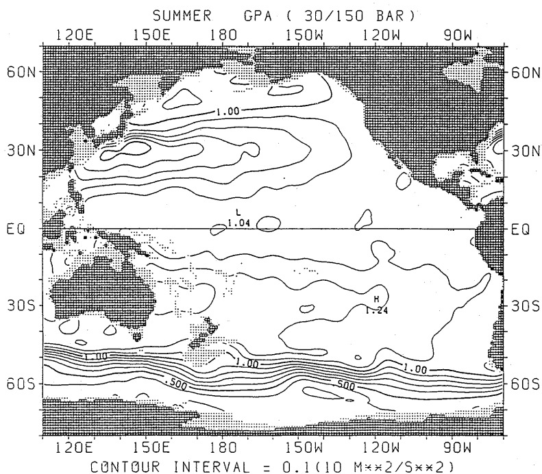
図 1.4.28 夏季における GPA の水平分布 (300m)
