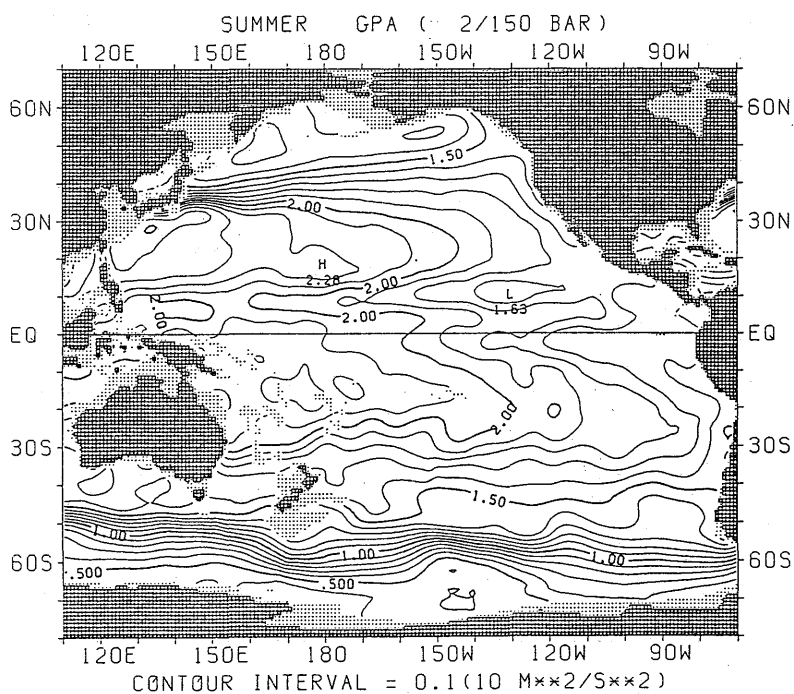
図 1.4.22 夏季における GPA の水平分布 (20m)
