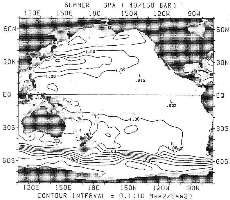
図 1.4.29 夏季における GPA の水平分布 (400m)
