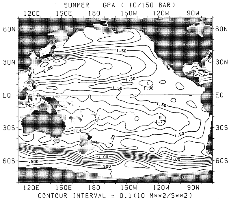
図 1.4.25 夏季における GPA の水平分布 (100m)
