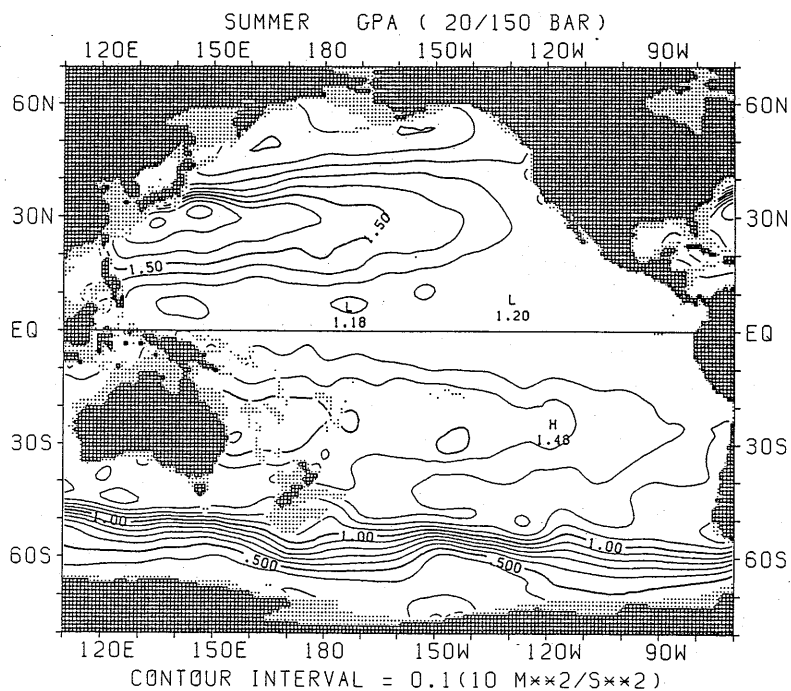
図 1.4.27 夏季における GPA の水平分布 (200m)
