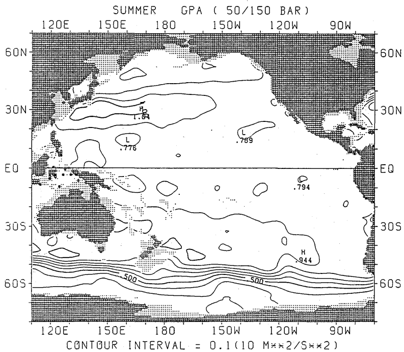
図 1.4.30 夏季における GPA の水平分布 (500m)
