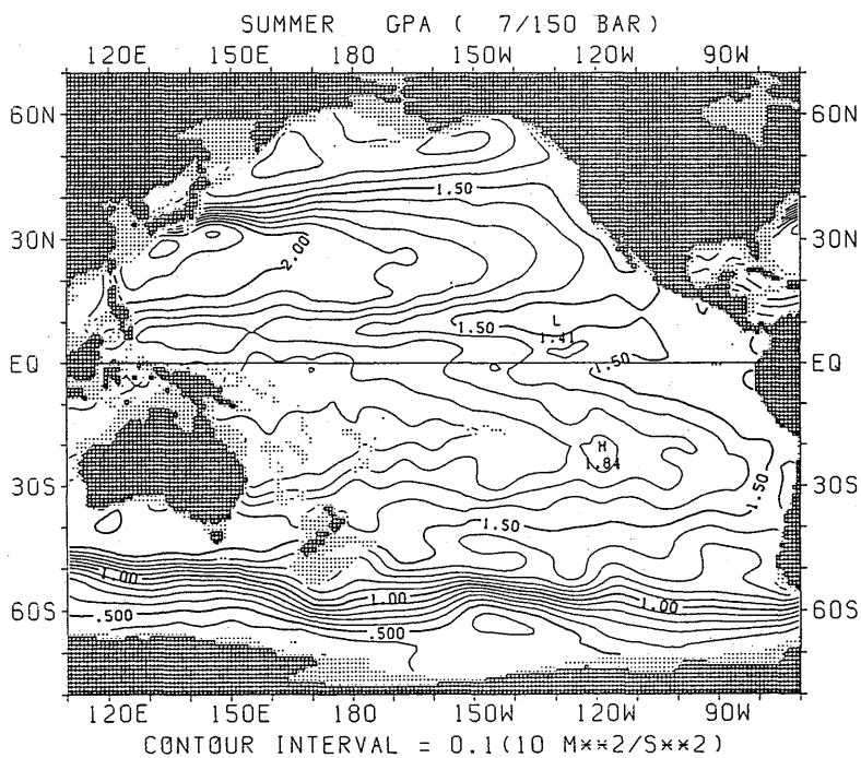
図 1.4.24 夏季における GPA の水平分布 (75m)
