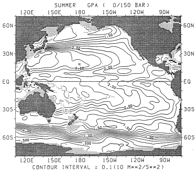
図 1.4.21 夏季における GPA の水平分布 (海面)
