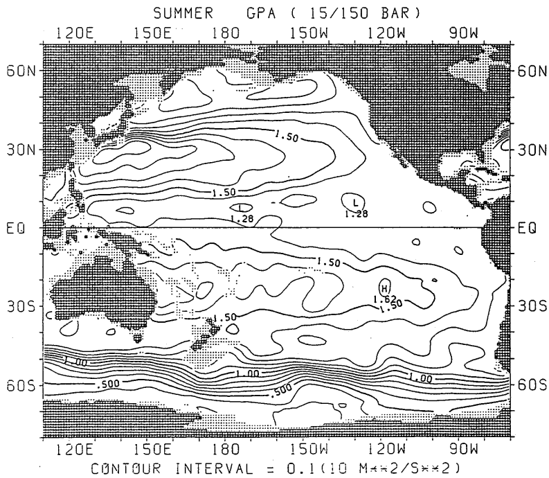
図 1.4.26 夏季における GPA の水平分布 (150m)
