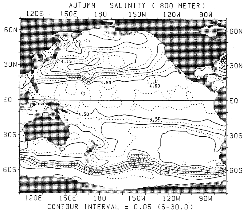
図 1.2.61 秋季における塩分水平分布 (800m)
