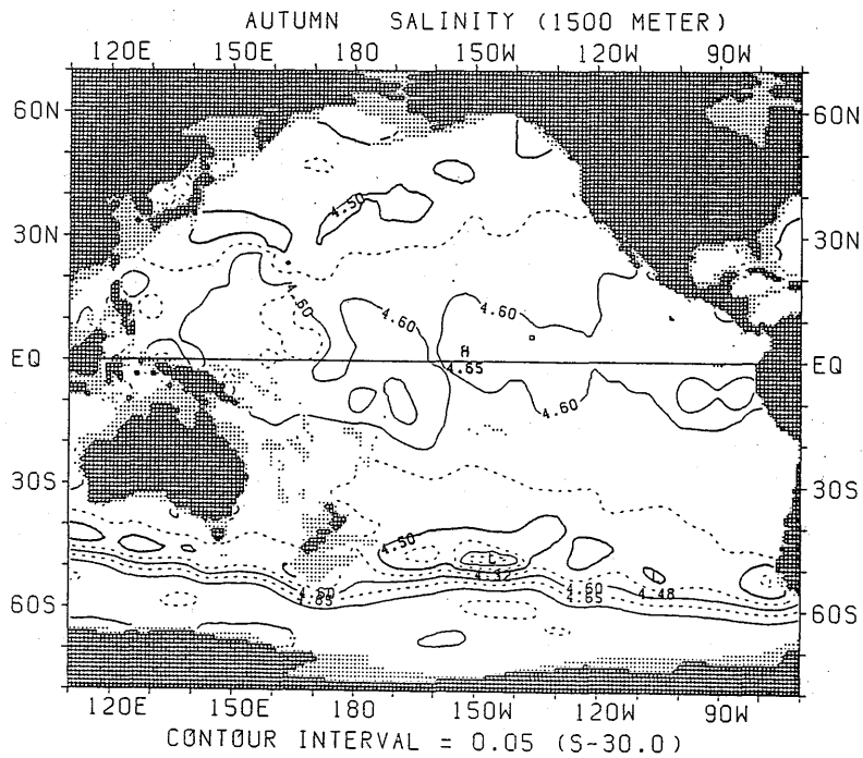
図 1.2.64 秋季における塩分水平分布 (1500m)
