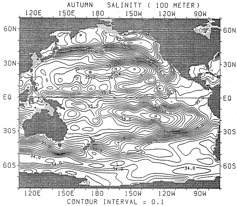
図 1.2.53 秋季における塩分水平分布 (100m)
