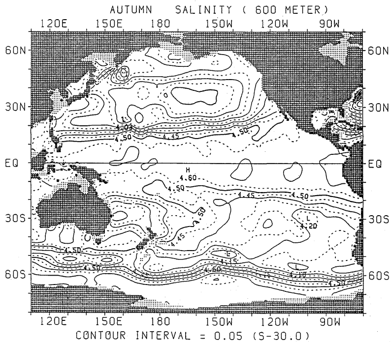
図 1.2.60 秋季における塩分水平分布 (600m)
