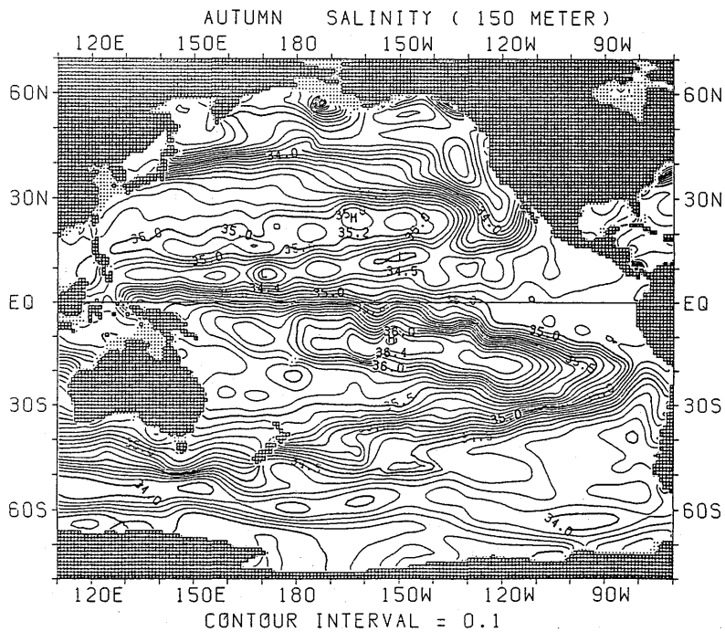
図 1.2.54 秋季における塩分水平分布 (150m)
