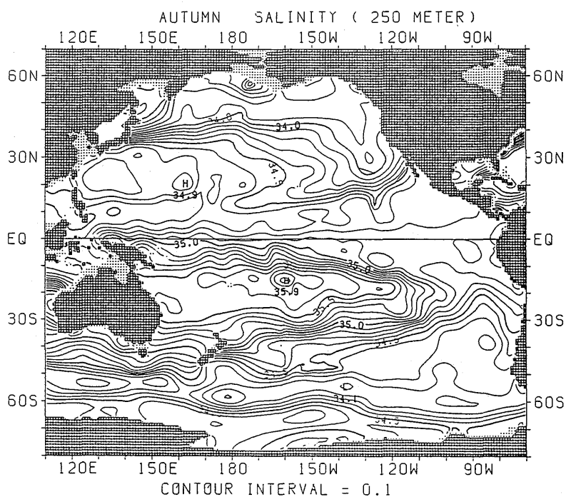
図 1.2.56 秋季における塩分水平分布 (250m)
