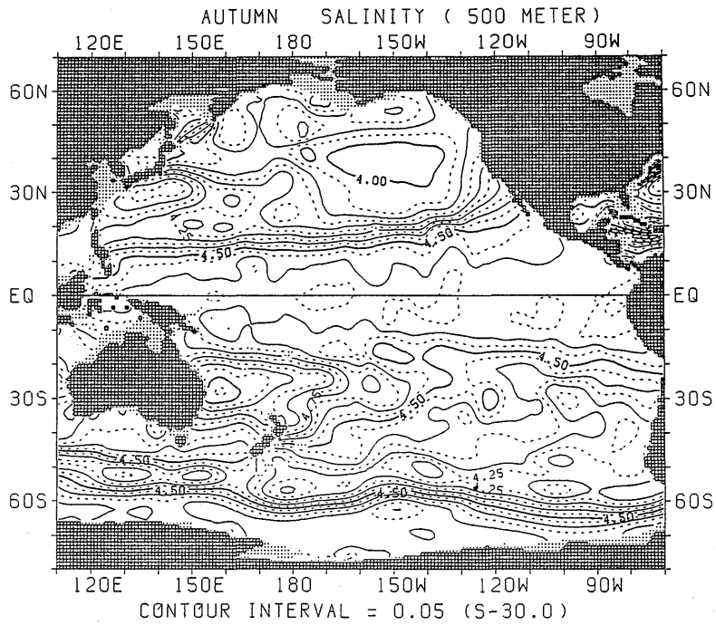
図 1.2.59 秋季における塩分水平分布 (500m)
