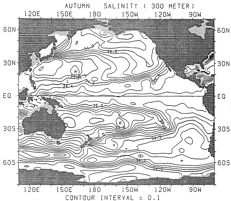
図 1.2.57 秋季における塩分水平分布 (300m)
