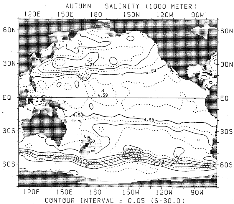
図 1.2.62 秋季における塩分水平分布 (1000m)
