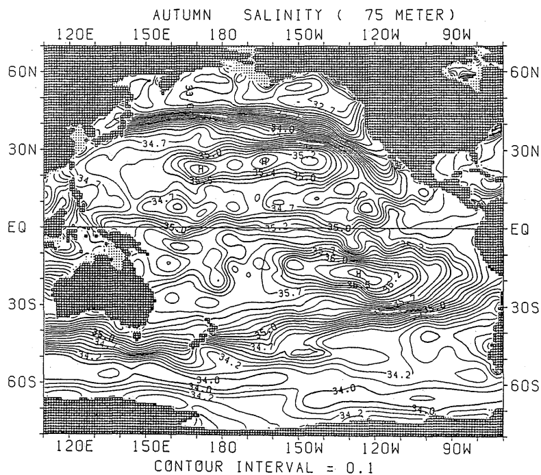
図 1.2.52 秋季における塩分水平分布 (75m)
