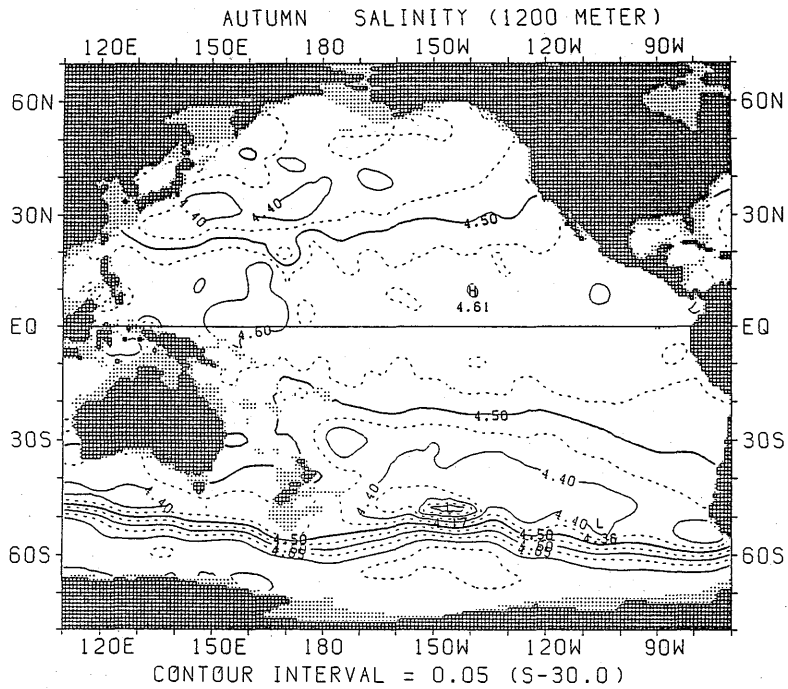
図 1.2.63 秋季における塩分水平分布 (1200m)
