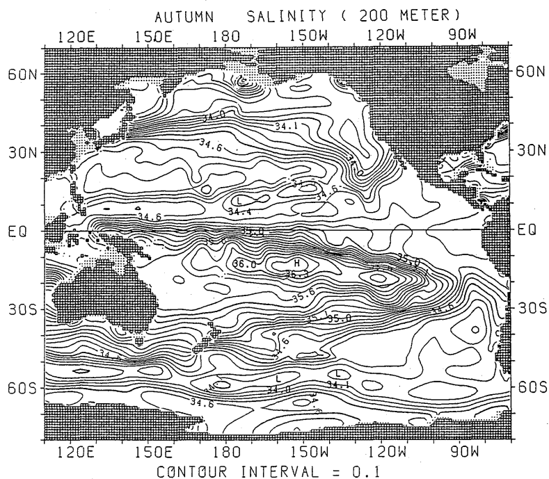
図 1.2.55 秋季における塩分水平分布 (200m)
