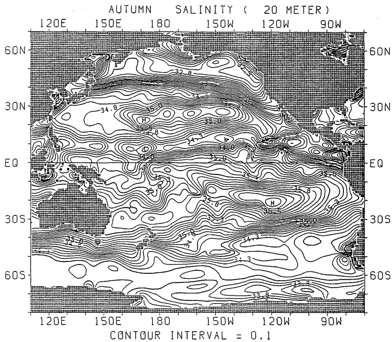
図 1.2.50 秋季における塩分水平分布 (20m)
