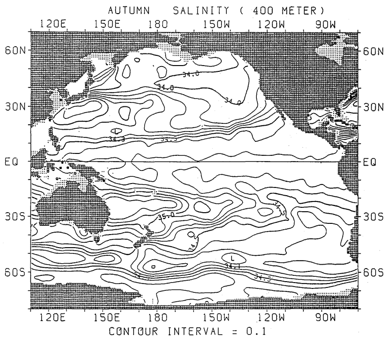
図 1.2.58 秋季における塩分水平分布 (400m)
