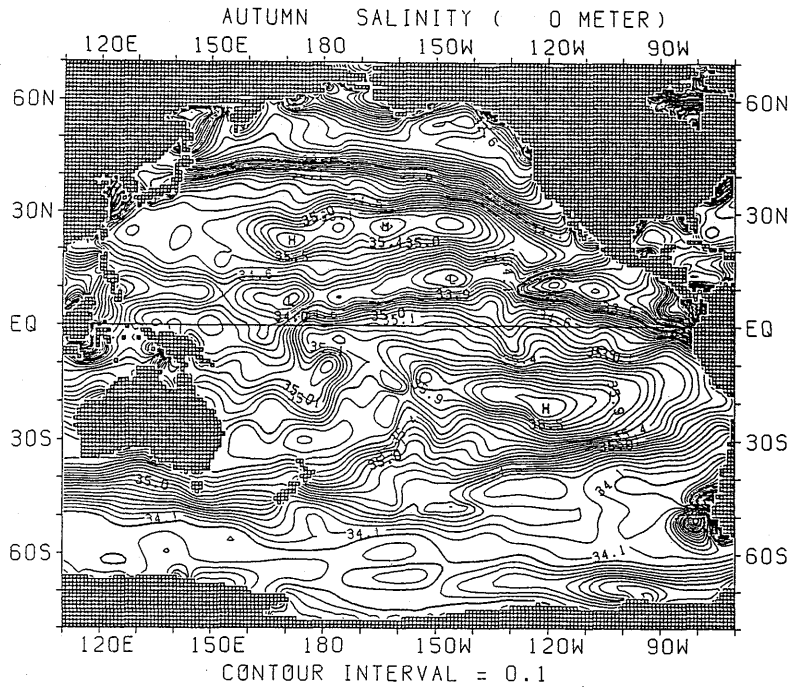
図 1.2.49 秋季における塩分水平分布 (海面)
