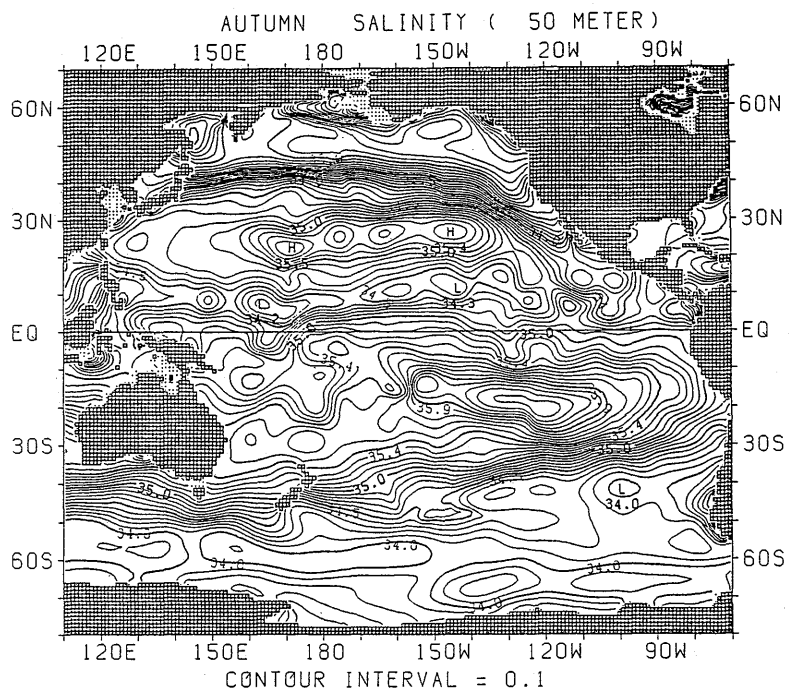
図 1.2.51 秋季における塩分水平分布 (50m)
