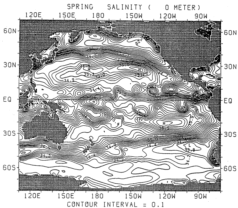
図 1.2.17 春季における塩分水平分布 (海面)
