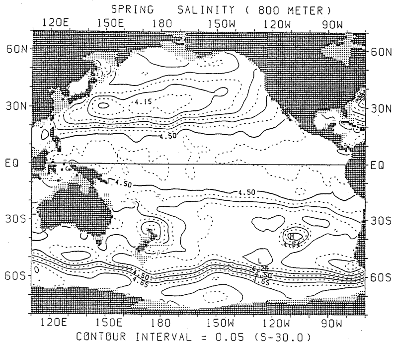
図 1.2.29 春季における塩分水平分布 (800m)
