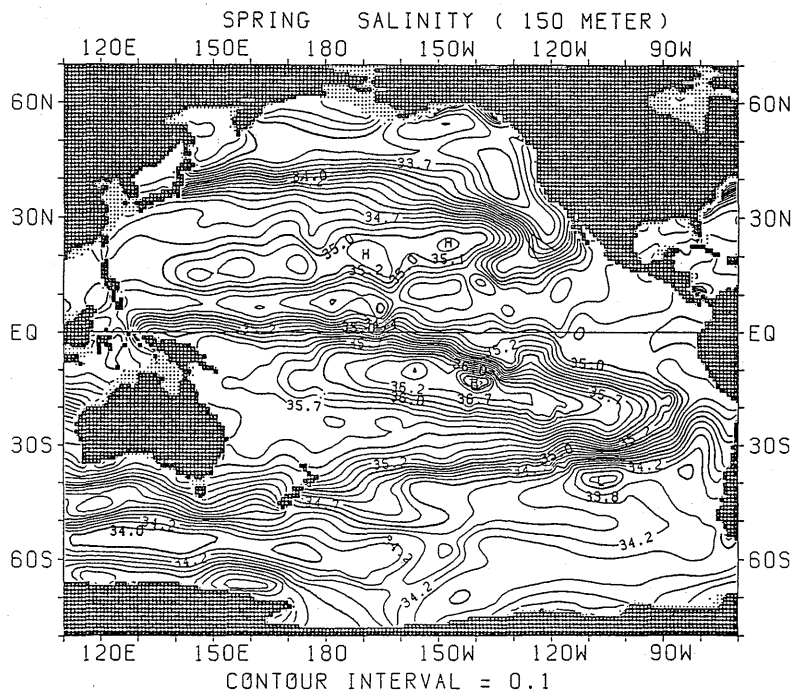
図 1.2.22 春季における塩分水平分布 (150m)
