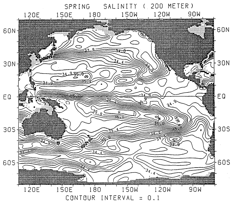
図 1.2.23 春季における塩分水平分布 (200m)
