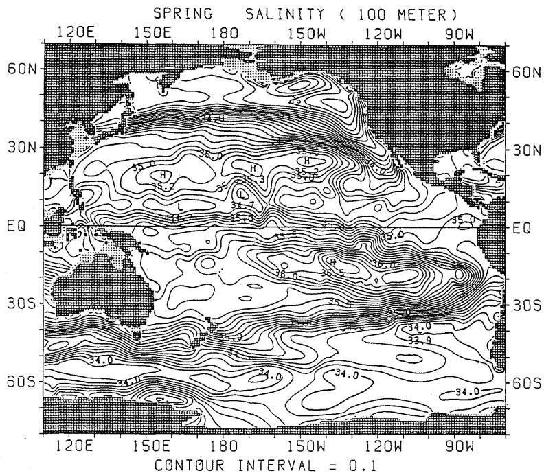
図 1.2.21 春季における塩分水平分布 (100m)
