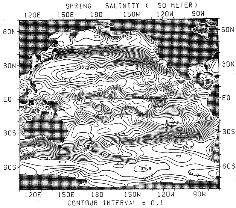
図 1.2.19 春季における塩分水平分布 (50m)
