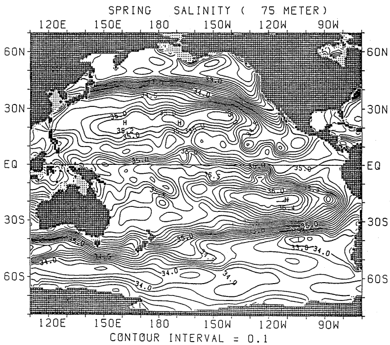
図 1.2.20 春季における塩分水平分布 (75m)
