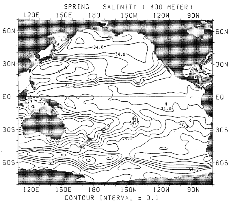
図 1.2.26 春季における塩分水平分布 (400m)
