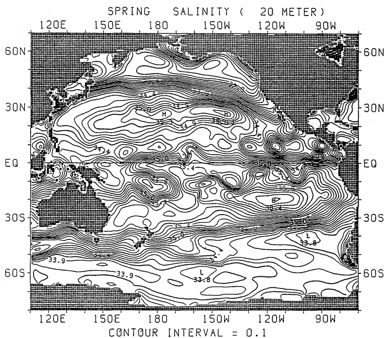
図 1.2.18 春季における塩分水平分布 (20m)
