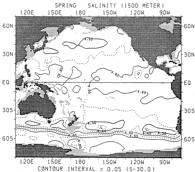
図 1.2.32 春季における塩分水平分布 (1500m)
