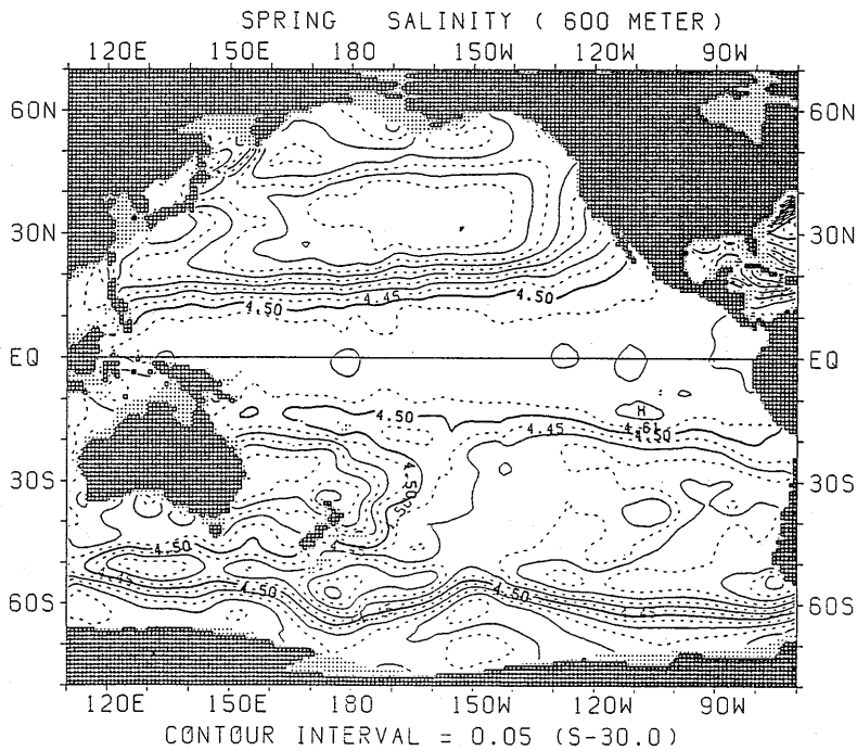
図 1.2.28 春季における塩分水平分布 (600m)
