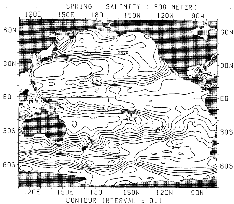
図 1.2.25 春季における塩分水平分布 (300m)
