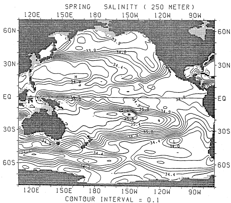
図 1.2.24 春季における塩分水平分布 (250m)
