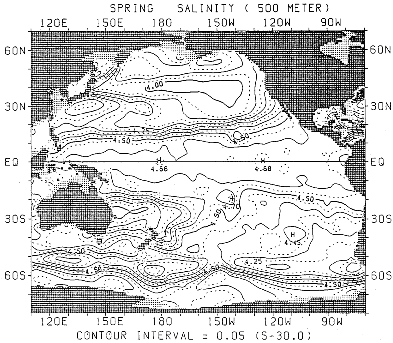
図 1.2.27 春季における塩分水平分布 (500m)
