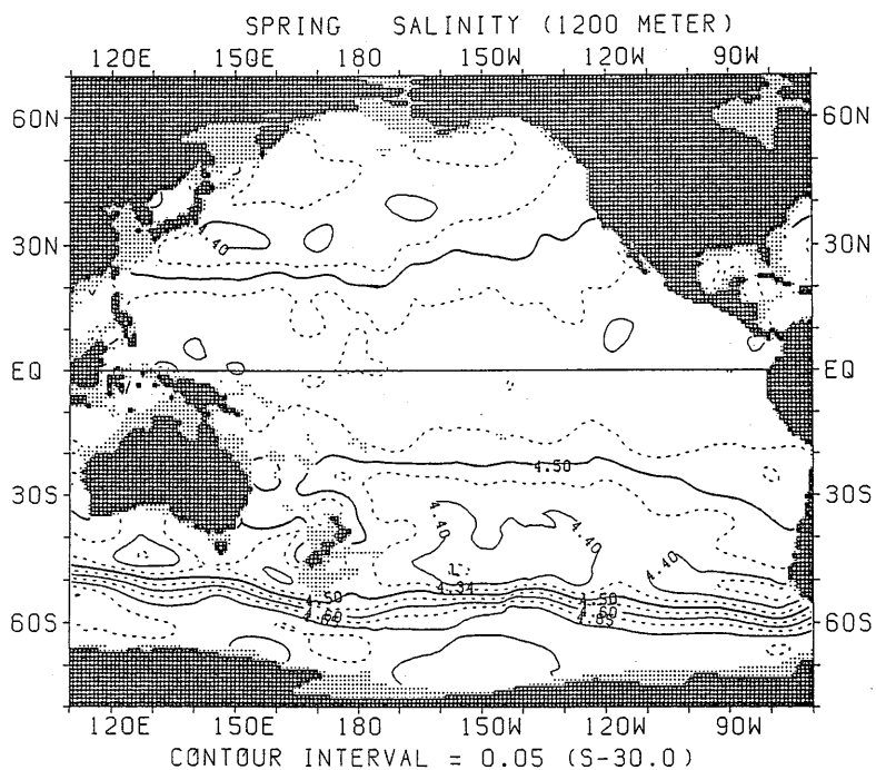
図 1.2.31 春季における塩分水平分布 (1200m)
