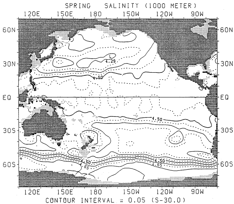
図 1.2.30 春季における塩分水平分布 (1000m)
