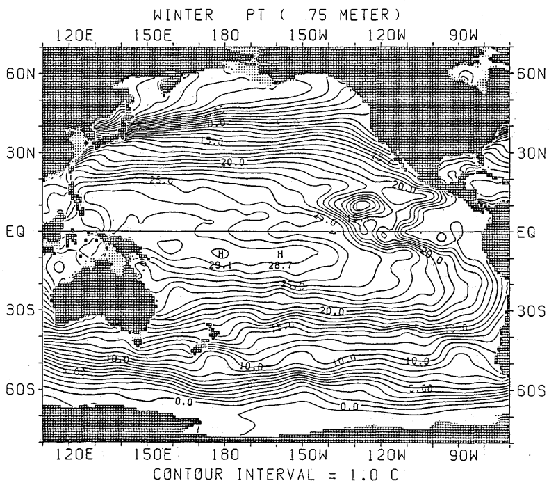
図 1.1.4 冬季におけるポテンシャル水温水平分布 (75m)
