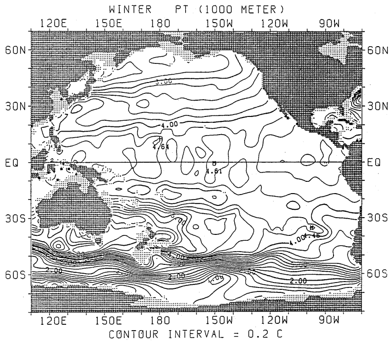
図 1.1.14 冬季におけるポテンシャル水温水平分布 (1000m)
