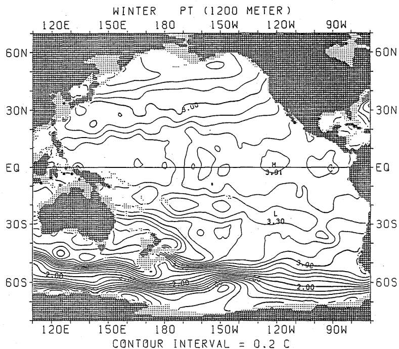
図 1.1.15 冬季におけるポテンシャル水温水平分布 (1200m)
