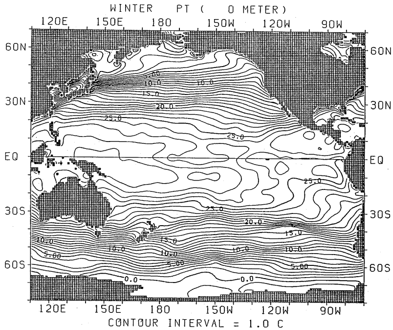
図 1.1.1 冬季におけるポテンシャル水温水平分布 (海面)
