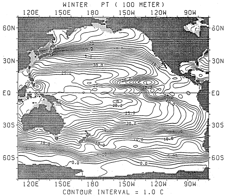
図 1.1.5 冬季におけるポテンシャル水温水平分布 (100m)
