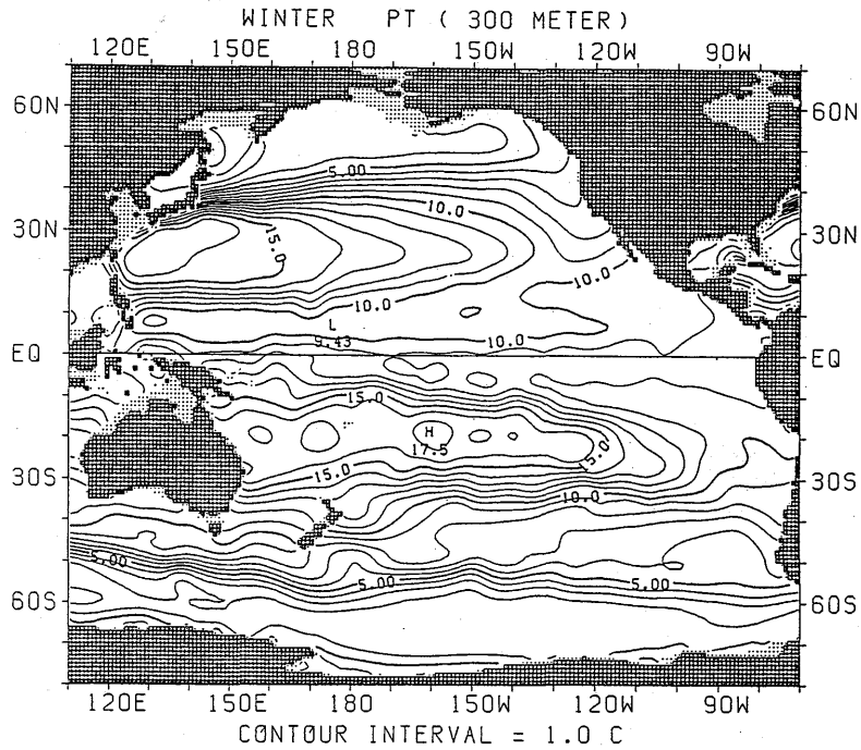
図 1.1.9 冬季におけるポテンシャル水温水平分布 (300m)
