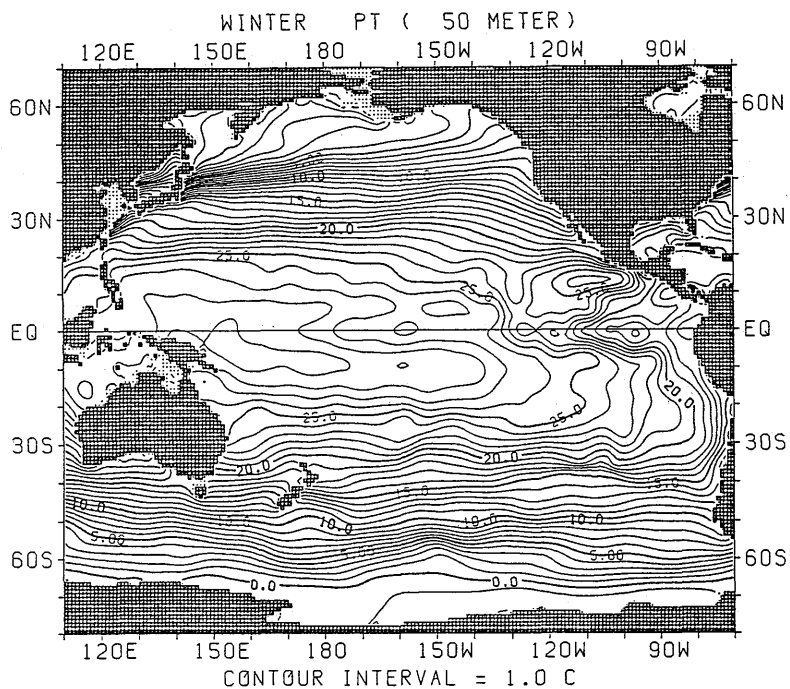
図 1.1.3 冬季におけるポテンシャル水温水平分布 (50m)
