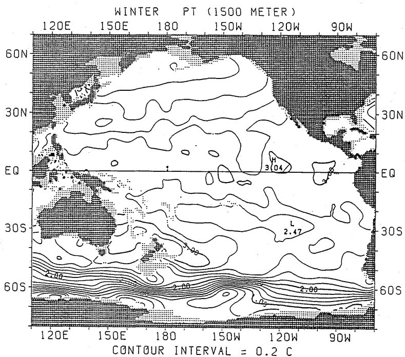
図 1.1.16 冬季におけるポテンシャル水温水平分布 (1500m)
