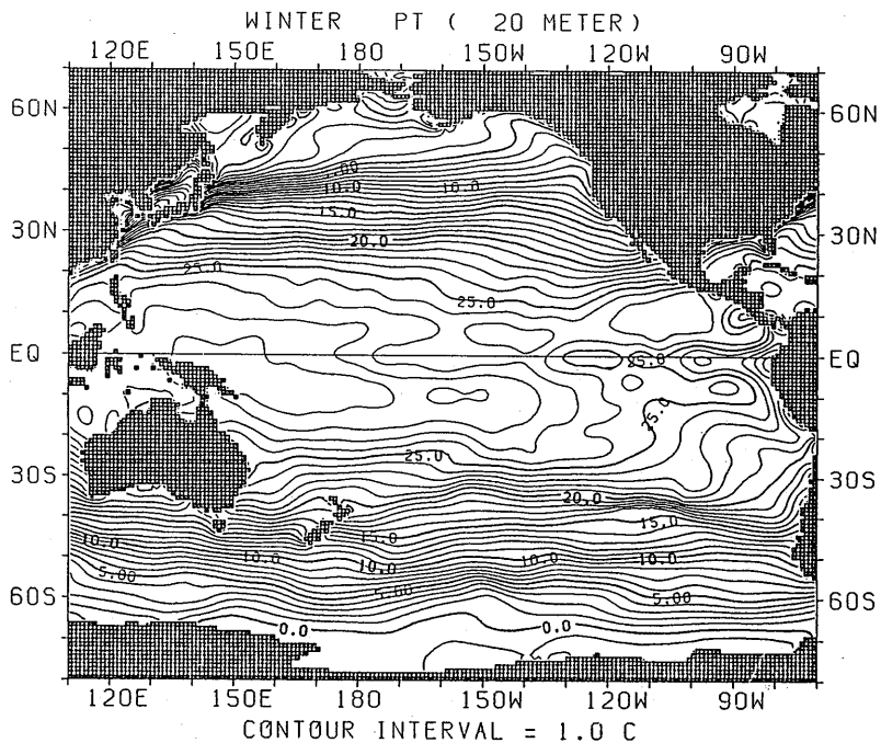
図 1.1.2 冬季におけるポテンシャル水温水平分布 (20m)
