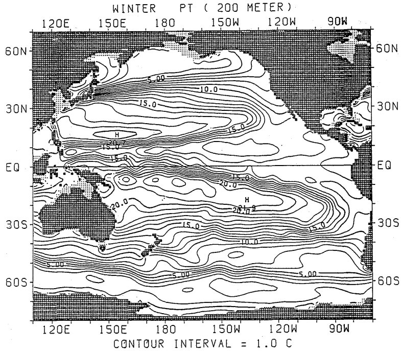
図 1.1.7 冬季におけるポテンシャル水温水平分布 (200m)
