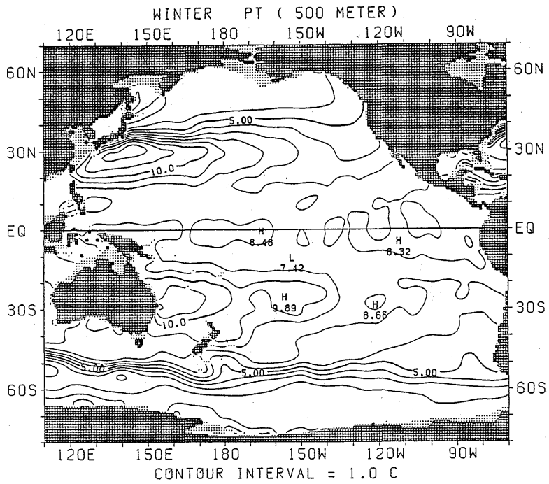
図 1.1.11 冬季におけるポテンシャル水温水平分布 (500m)
