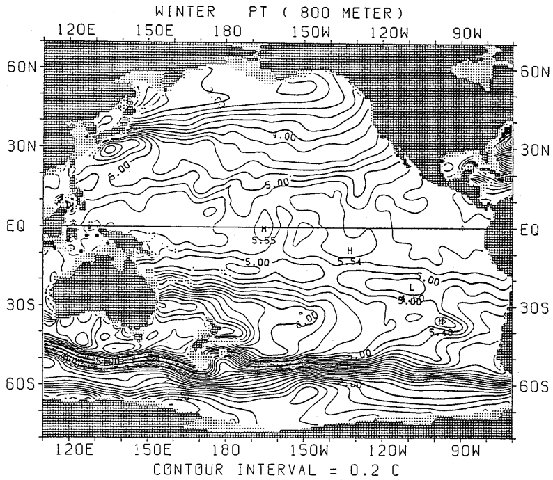
図 1.1.13 冬季におけるポテンシャル水温水平分布 (800m)
