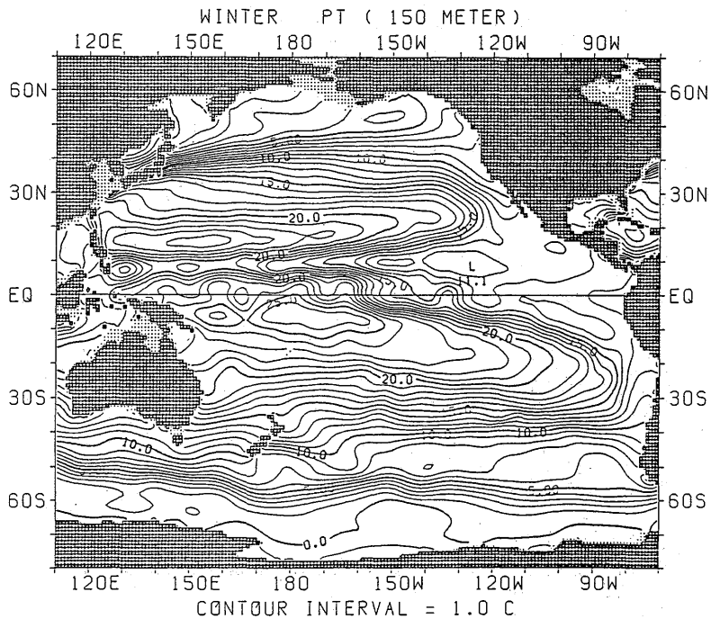
図 1.1.6 冬季におけるポテンシャル水温水平分布 (150m)
