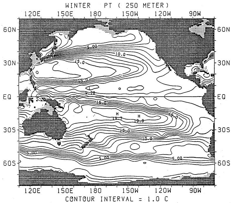
図 1.1.8 冬季におけるポテンシャル水温水平分布 (250m)
