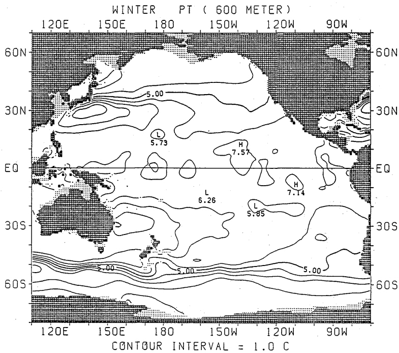
図 1.1.12 冬季におけるポテンシャル水温水平分布 (600m)
