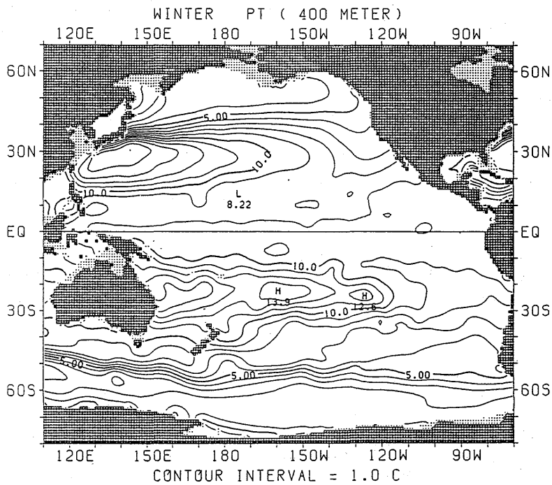
図 1.1.10 冬季におけるポテンシャル水温水平分布 (400m)
