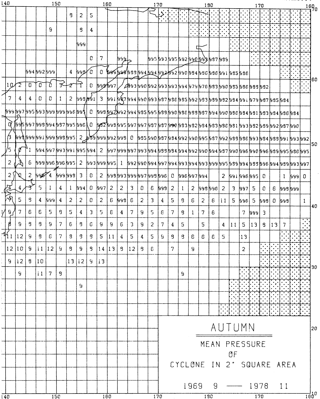
図版65 低気圧の平均中心気圧 (秋) (数値表示)
