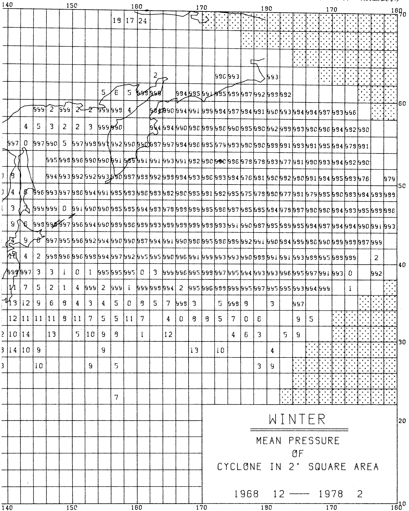
図版62 低気圧の平均中心気圧（冬）（数値表示）
