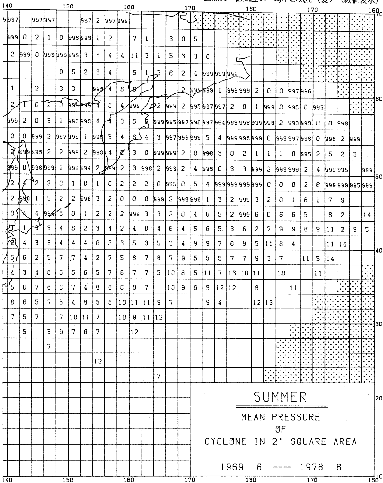
図版64 低気圧の平均中心気圧 (夏) (数値表示)
