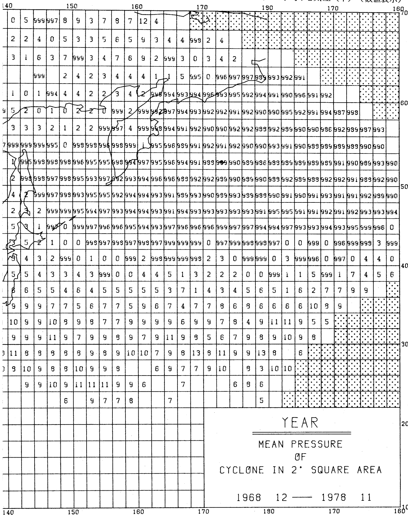
図版66 低気圧の平均中心気圧 (年) (数値表示)
