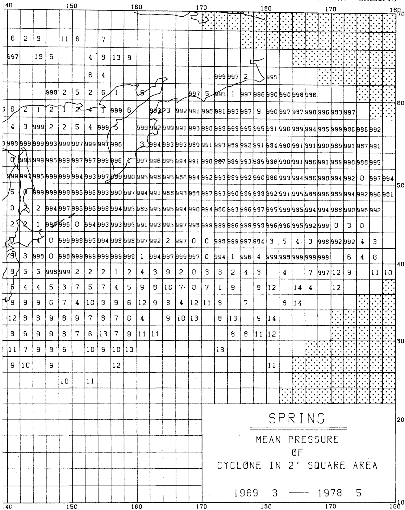
図版63 低気圧の平均中心気圧 (春) (数値表示)
