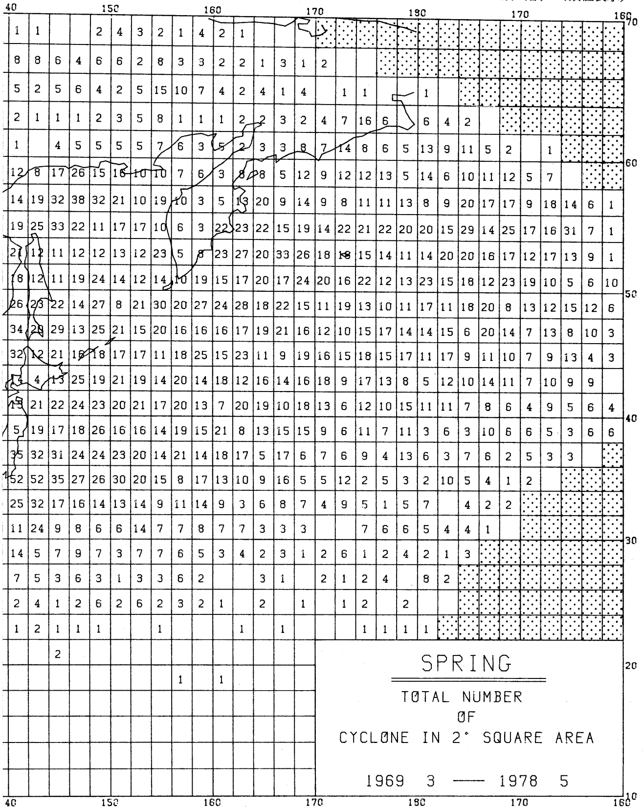
図版53 低気圧の総数（春）（数値表示）
