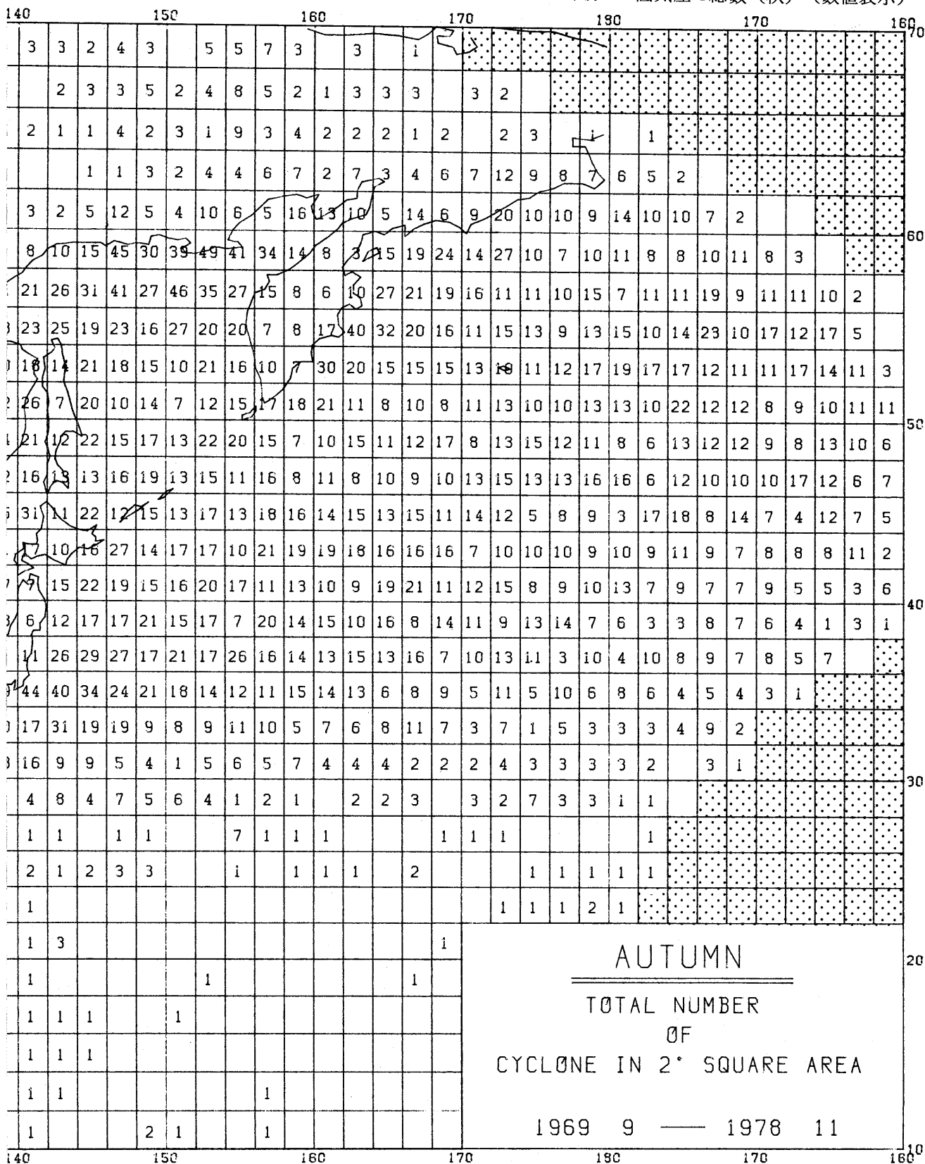
図版55 低気圧の総数（秋）（数値表示）
