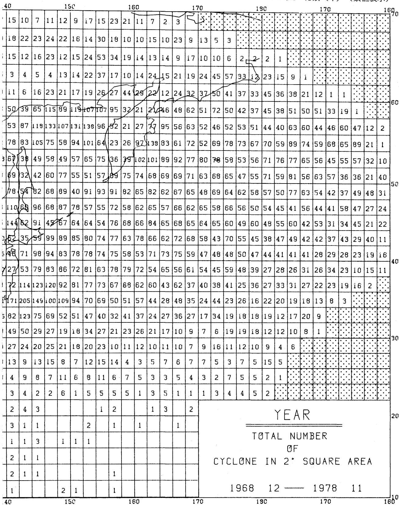
図版56 低気圧の総数（年）（数値表示）
