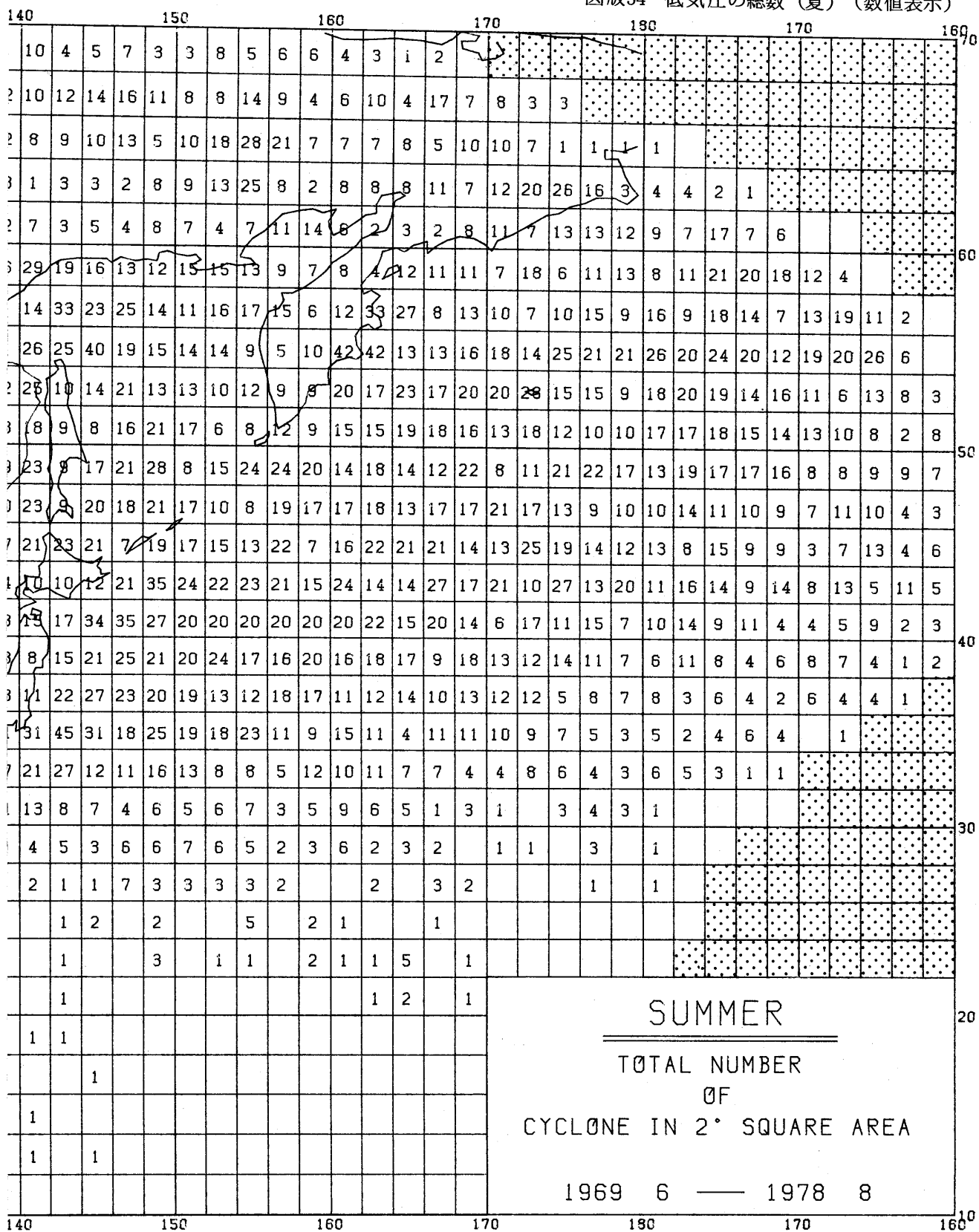
図版54 低気圧の総数（夏）（数値表示）
