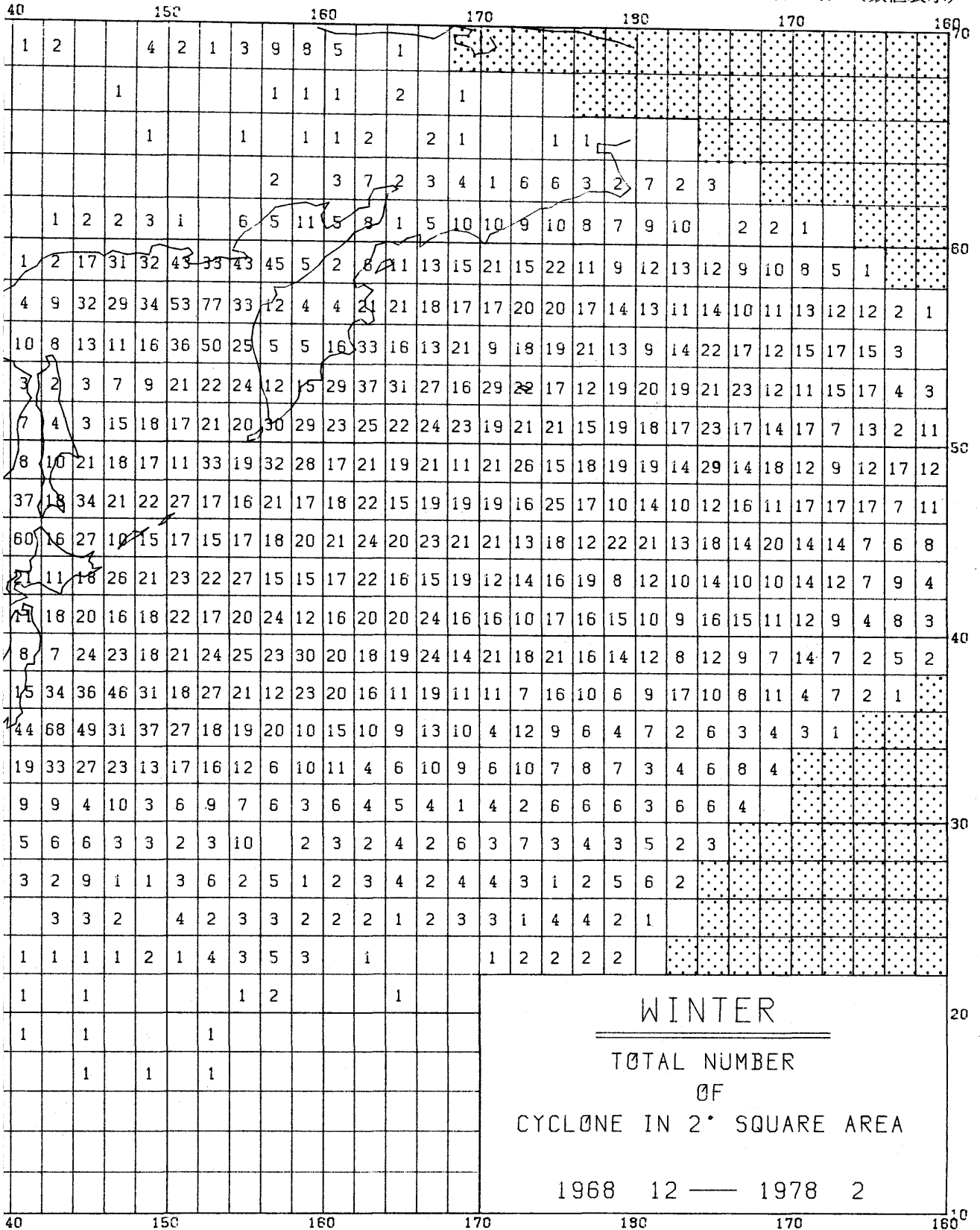
図版52 低気圧の総数（冬）（数値表示）
