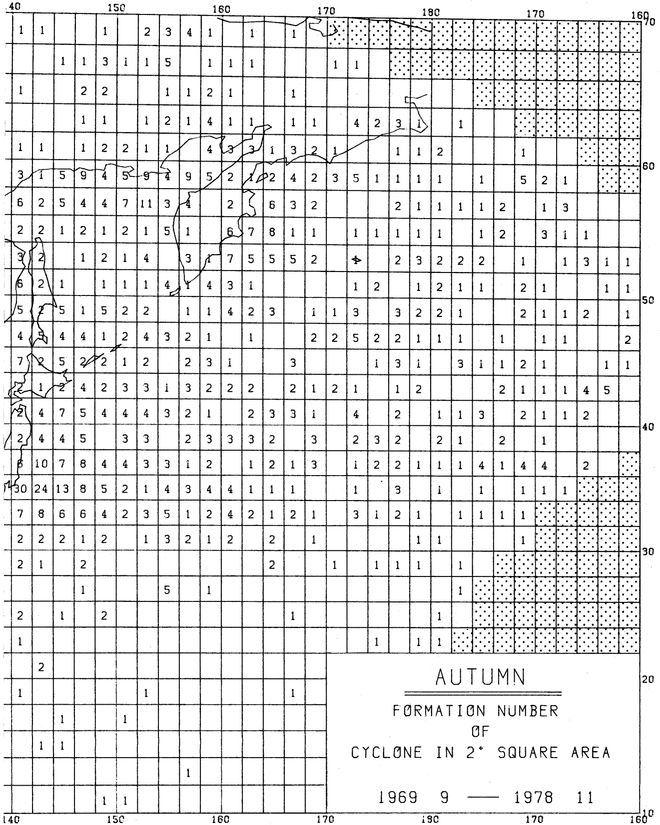
図版50 低気圧の発生数（秋）（数値表示）
