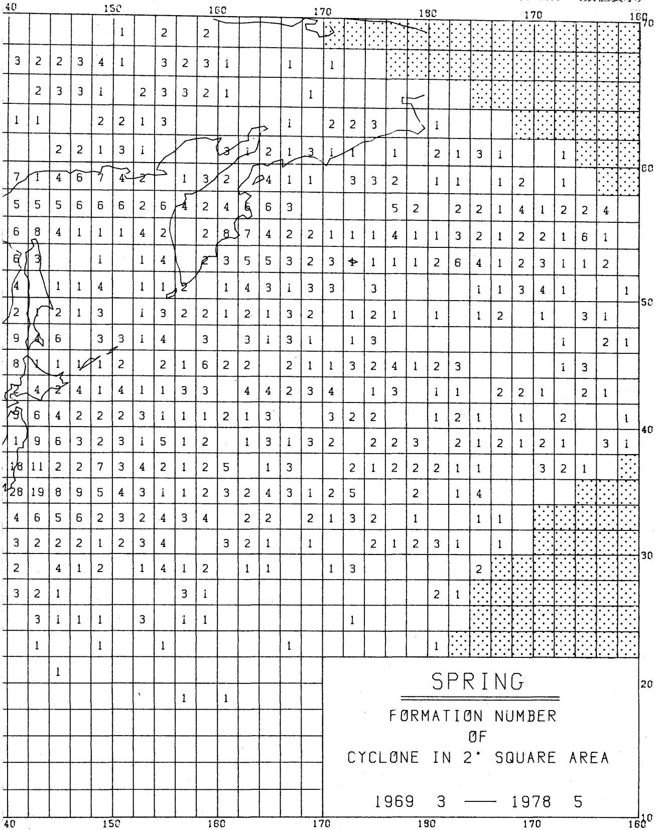
図版48 低気圧の発生数（春）（数値表示）
