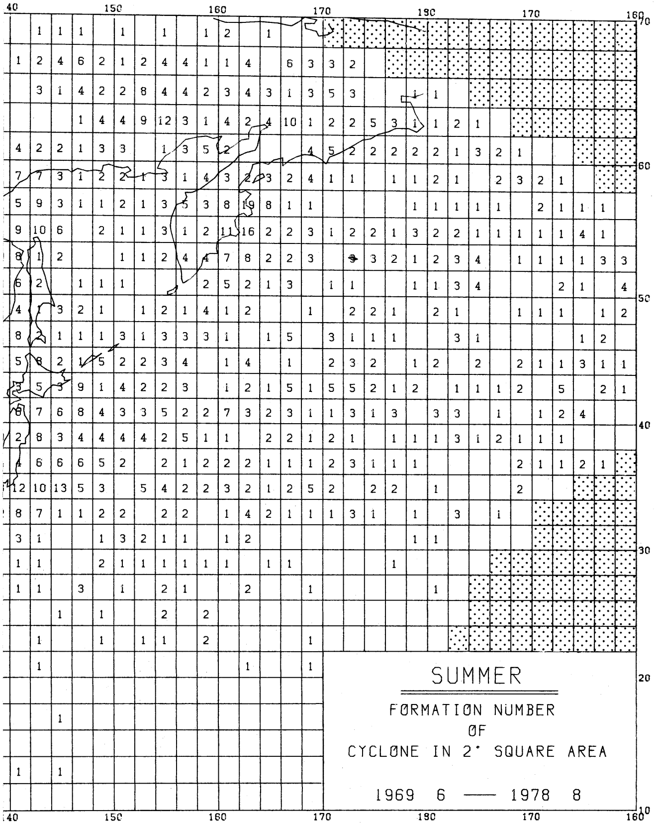
図版49 低気圧の発生数（夏）（数値表示）
