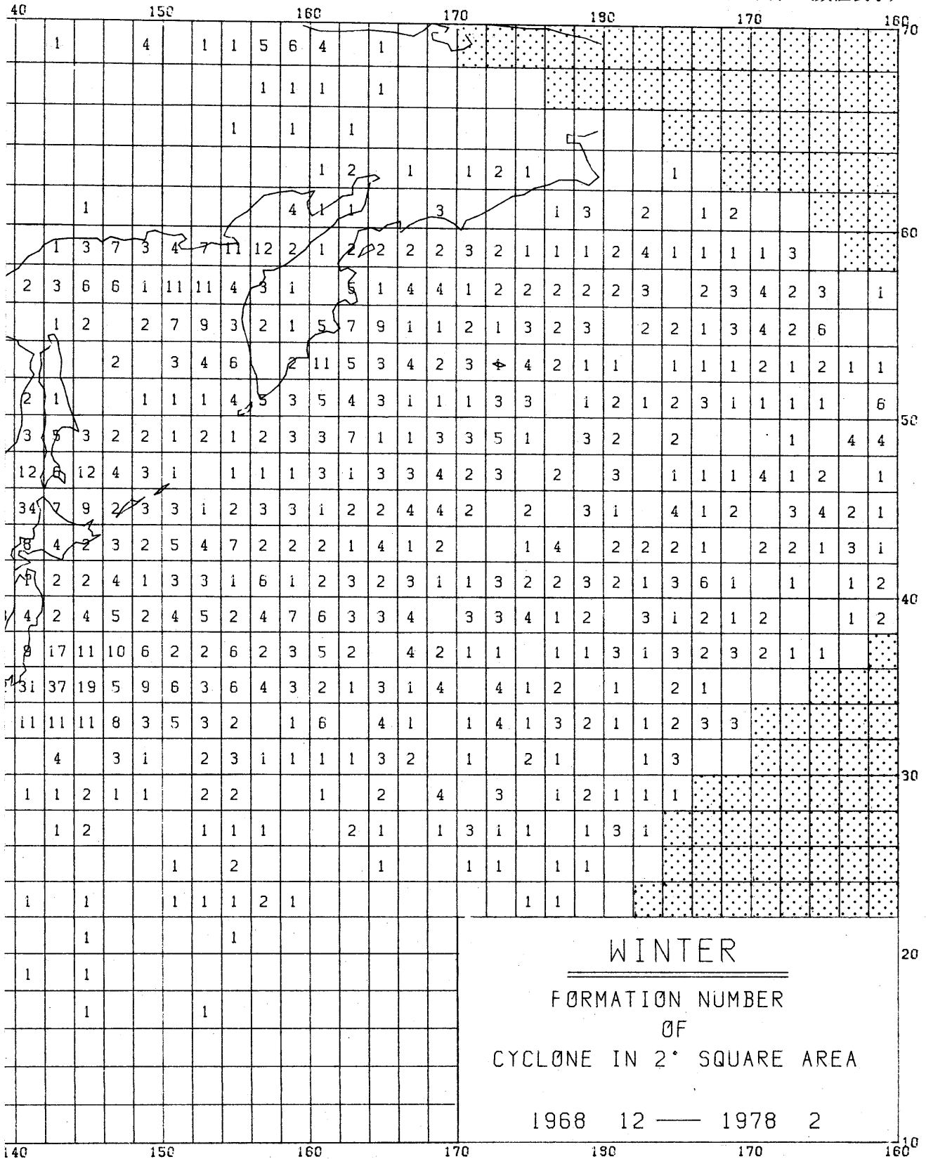
図版47 低気圧の発生数（冬）（数値表示）
