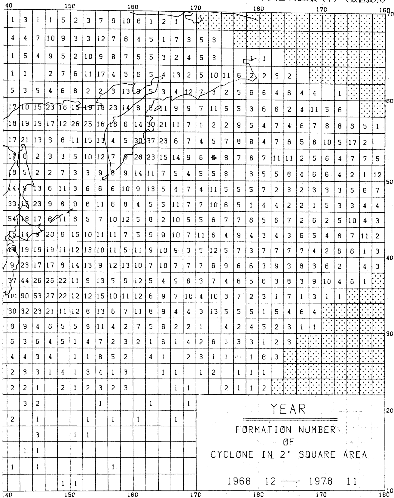
図版51 低気圧の発生数（年）（数値表示）
