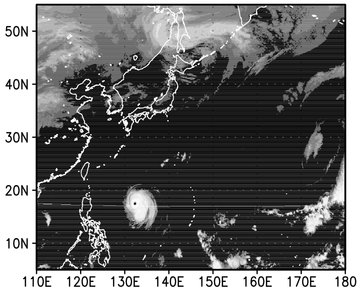
00z23oct2004
