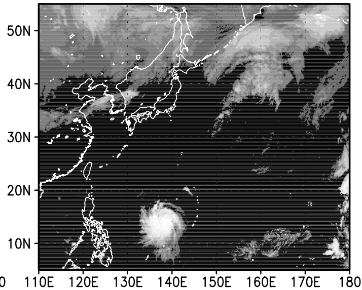
12z22oct2004
