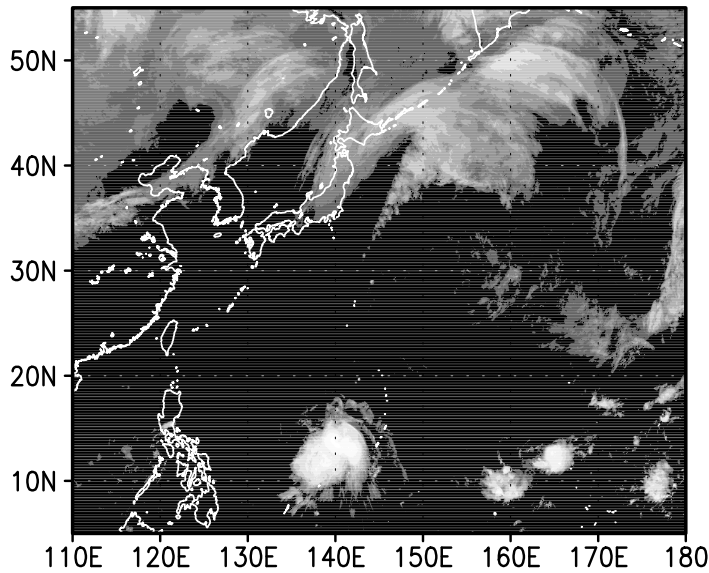
00z22oct2004
