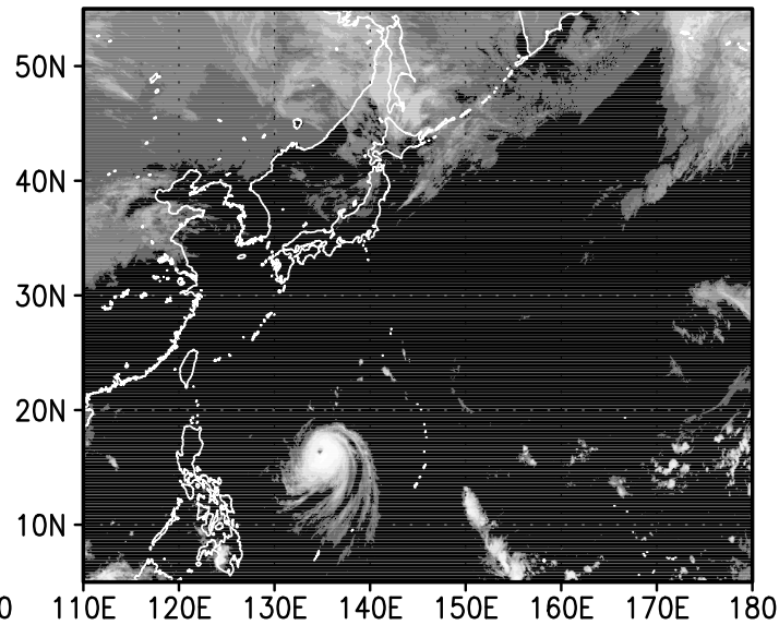
12z23oct2004
