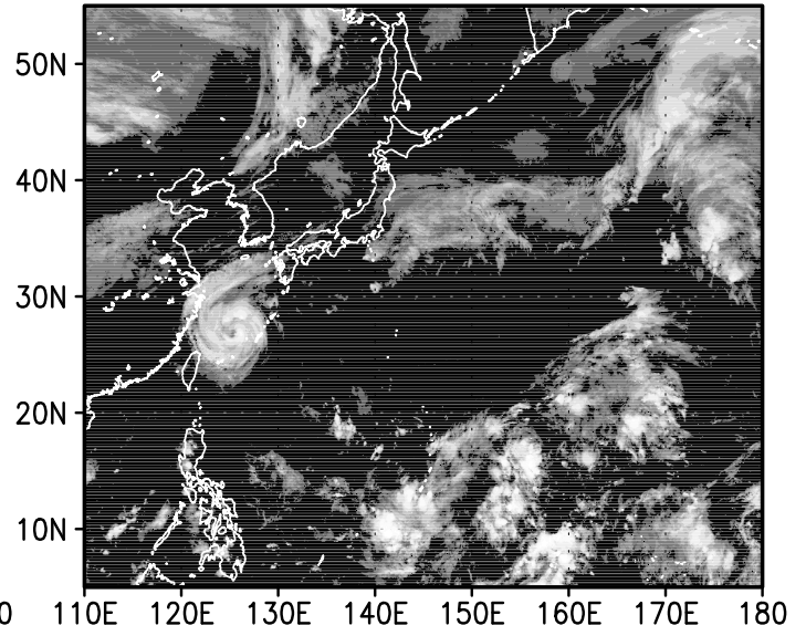
12z27sep2004
