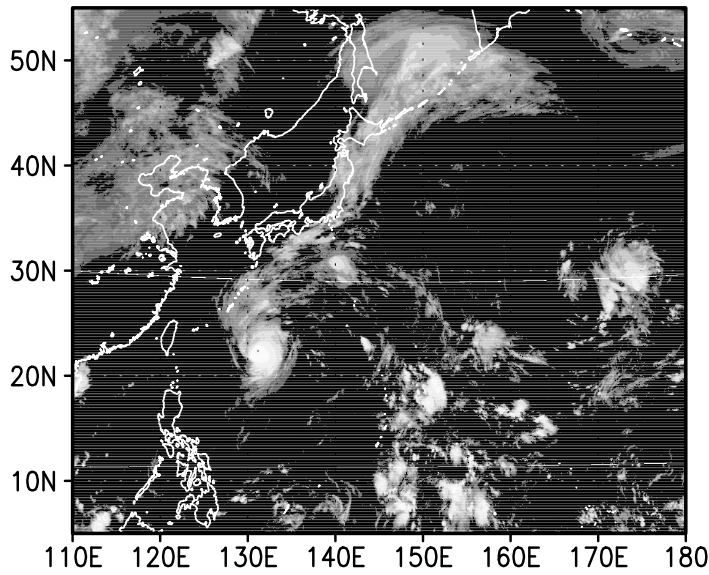
00z26sep2004
