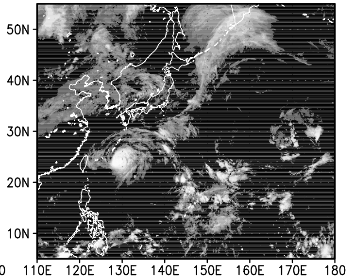
12z26sep2004
