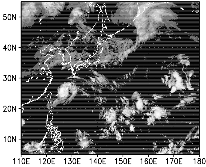
00z27sep2004
