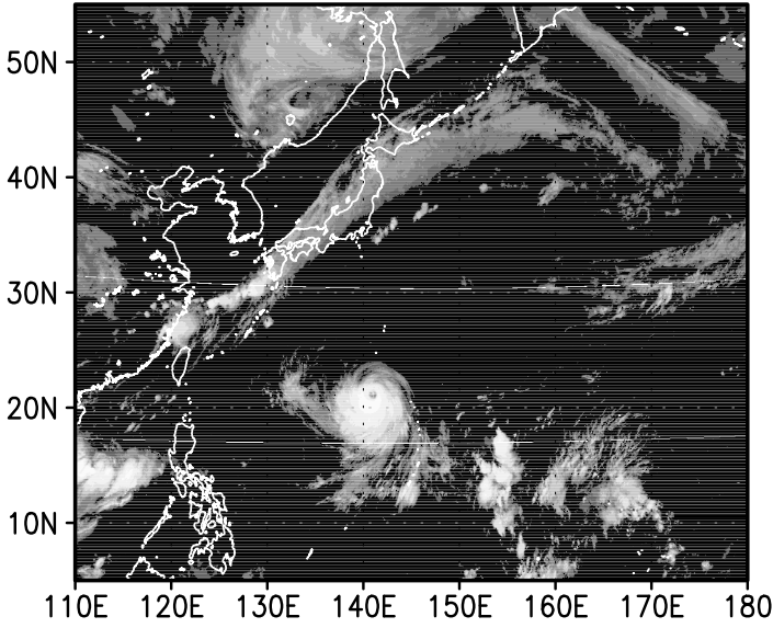
00z03sep2004
