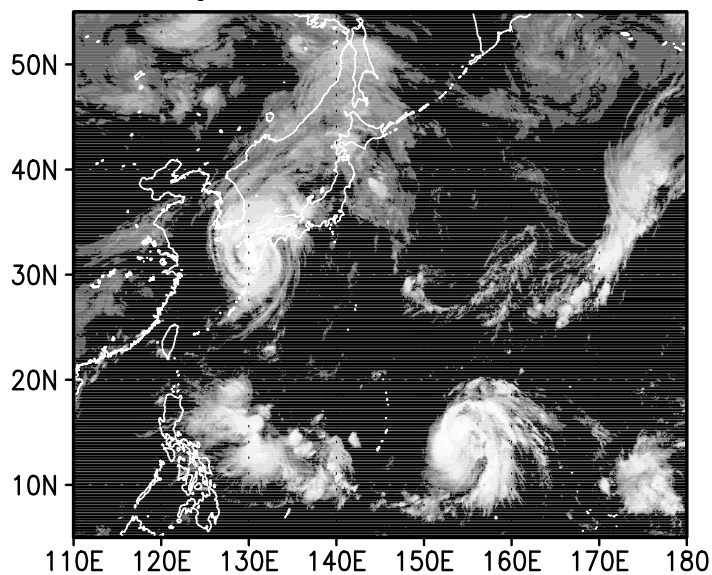
00z31aug2004
