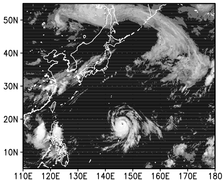
00z01sep2004
