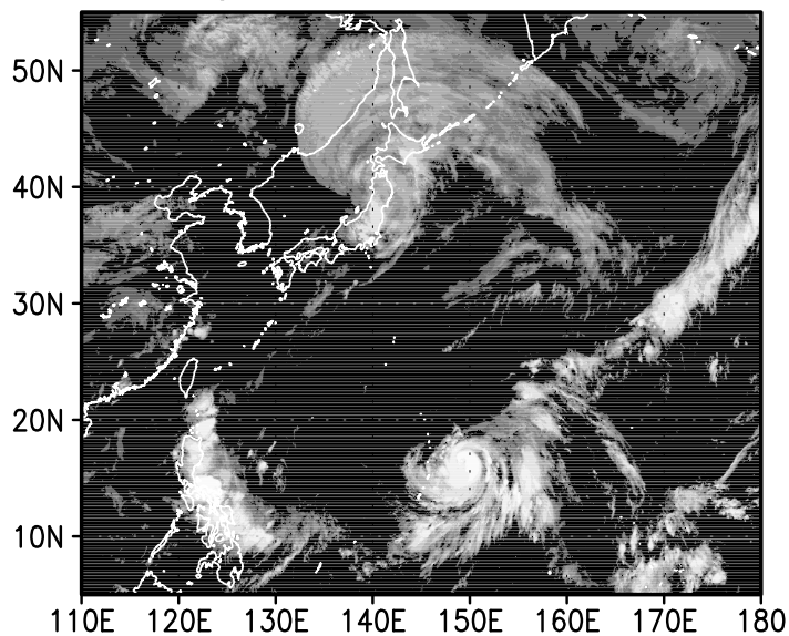
00z01sep2004
