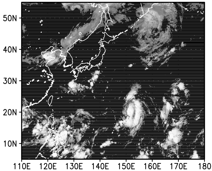
00z25jul2004
