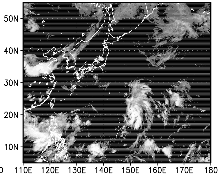
12z25jul2004
