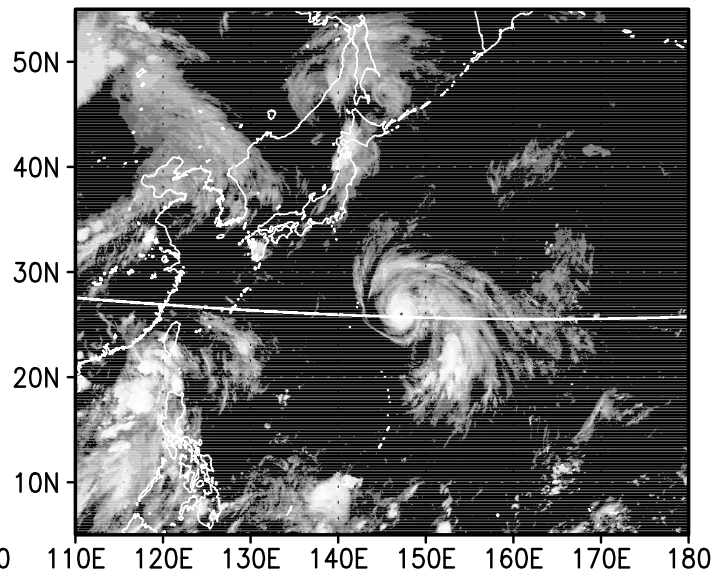
12z26jul2004
