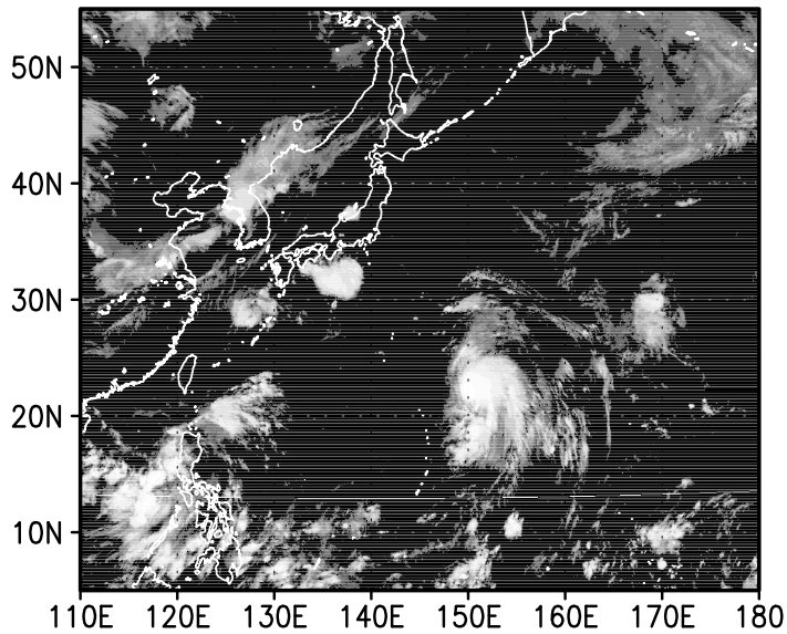
00z26jul2004
