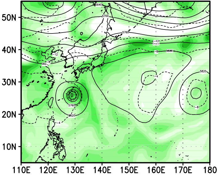
00z06sep2004
