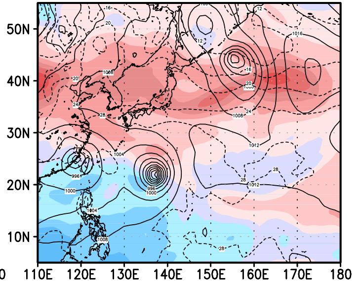
12z26aug2004
