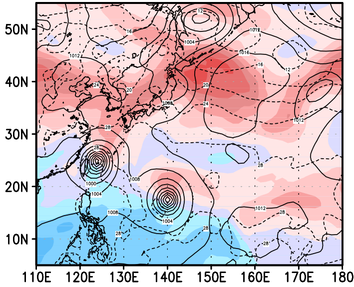
00z25aug2004
