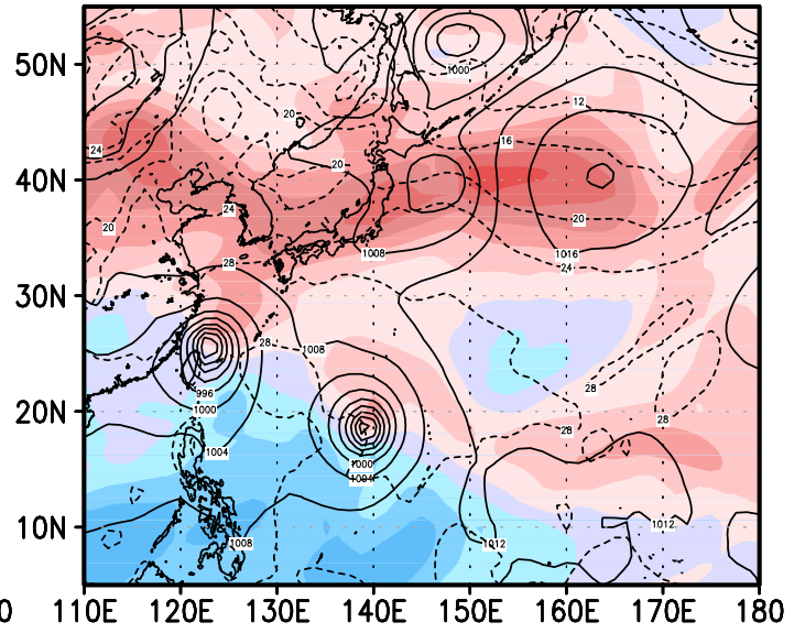
12z25aug2004
