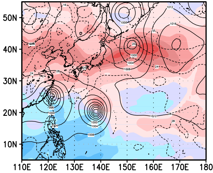
00z26aug2004
