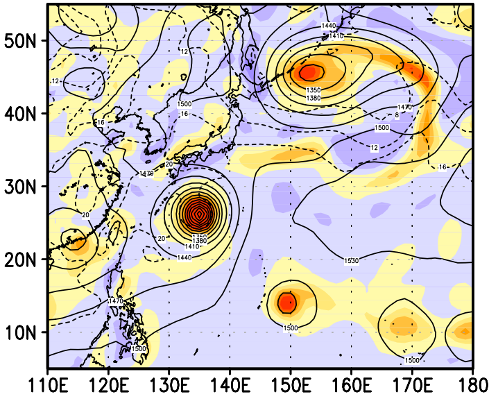
00z28aug2004
