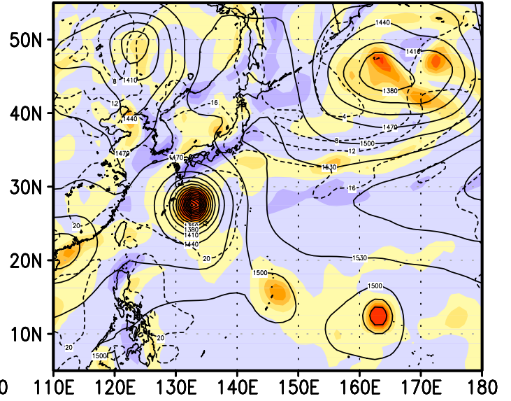
12z29aug2004
