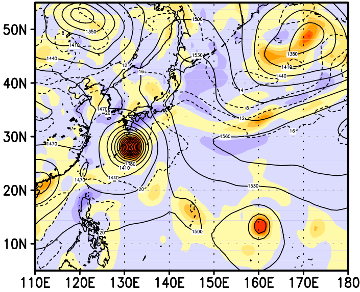
00z29aug2004
