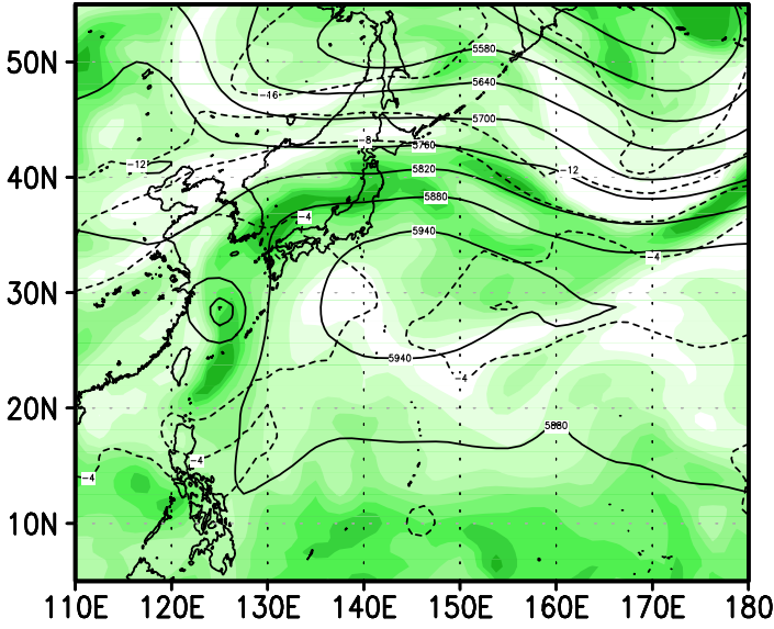
00z19aug2004
