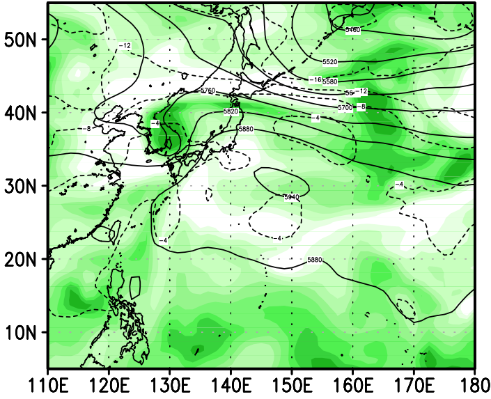
00z20aug2004
