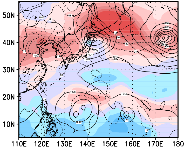
00z21aug2004
