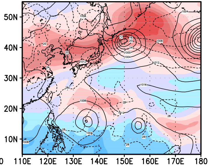
12z21aug2004
