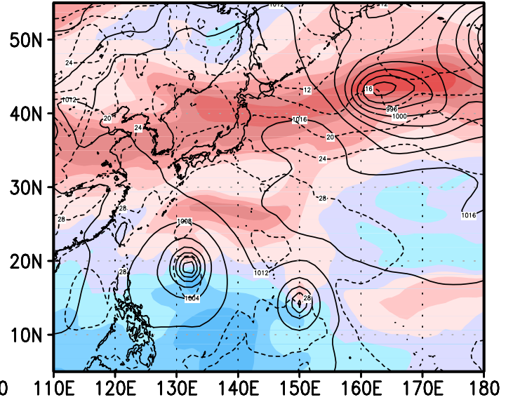
12z22aug2004
