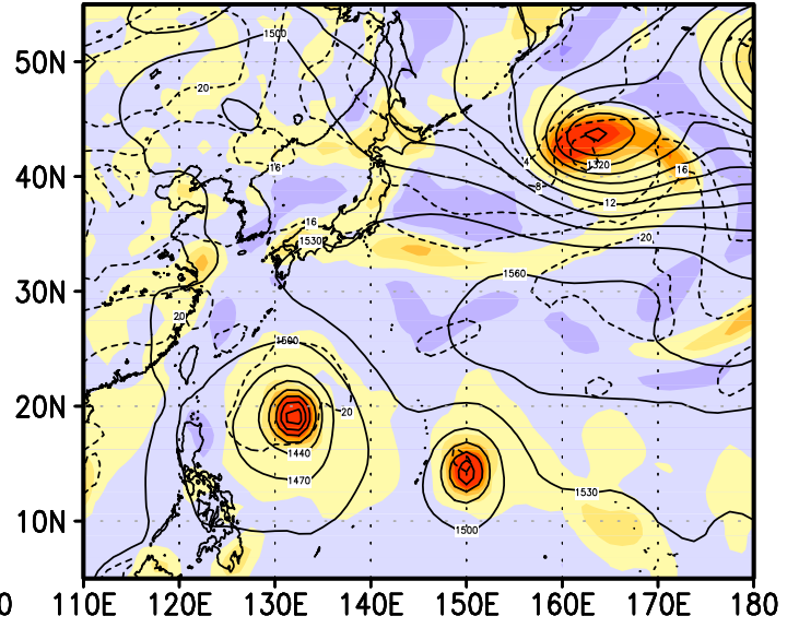
12z22aug2004
