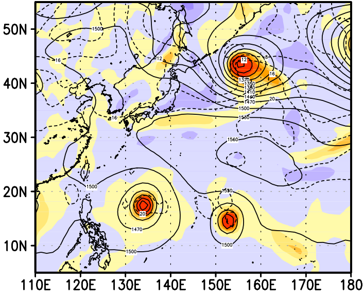
00z22aug2004
