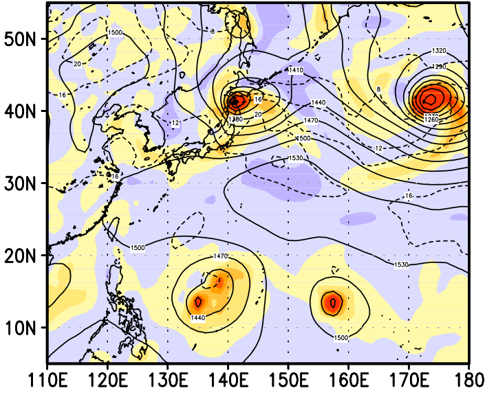
00z21aug2004
