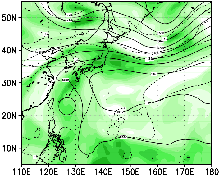
00z18aug2004
