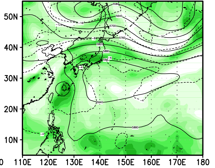
12z18aug2004
