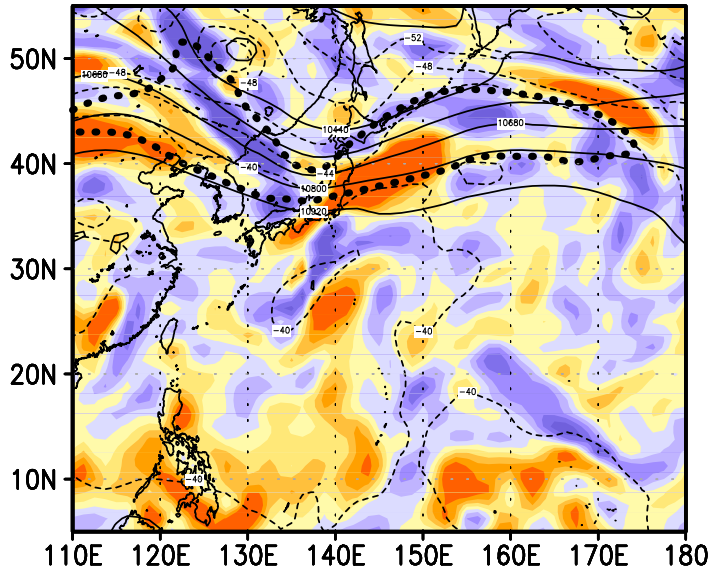
00z16aug2004
