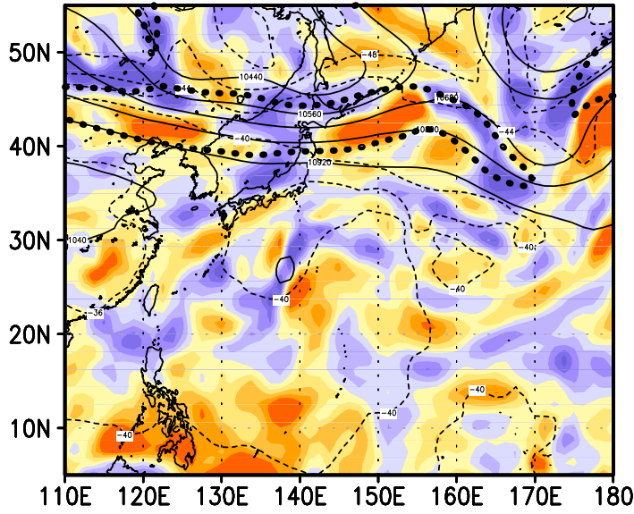
00z15aug2004
