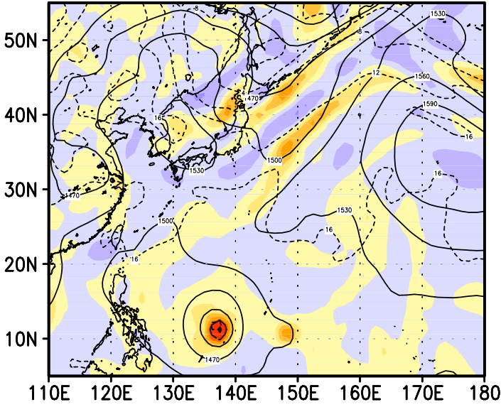
00z16jun2004
