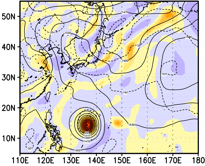
00z17jun2004
