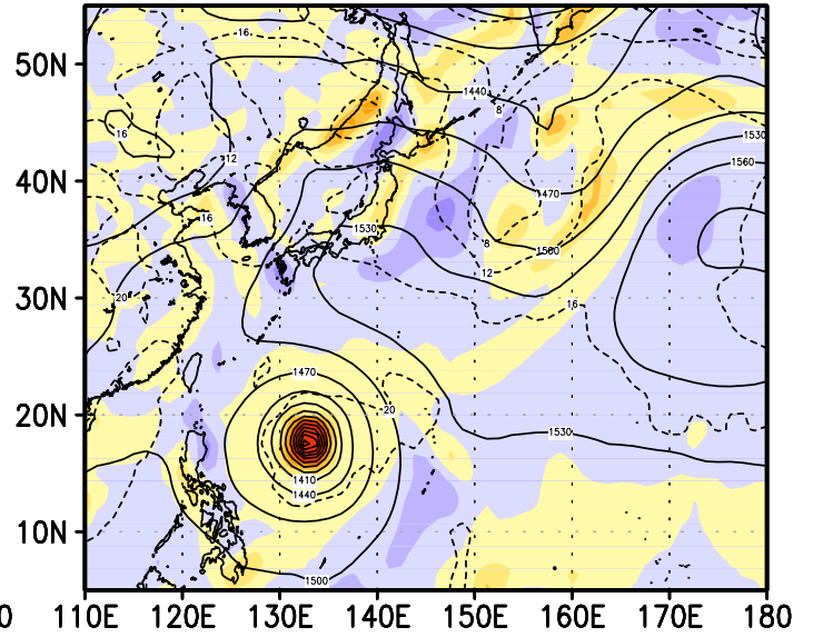
12z17jun2004
